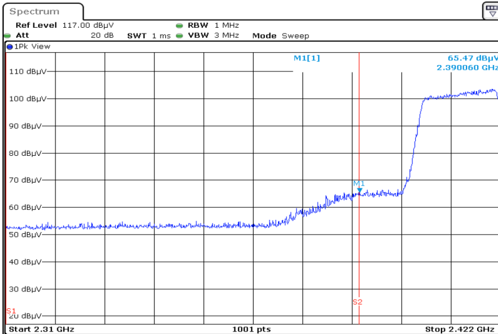
2 2422.0 F1 RestrictedBand Horizontal PEAK
