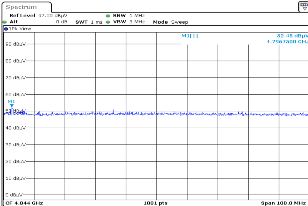
12 F1 X2 4844.0 Harmonic Vertical PEAK
