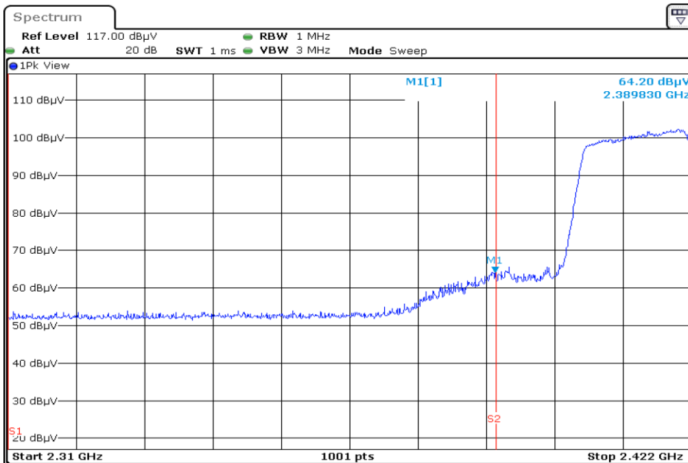
4 2422.0 F1 RestrictedBand Vertical PEAK
