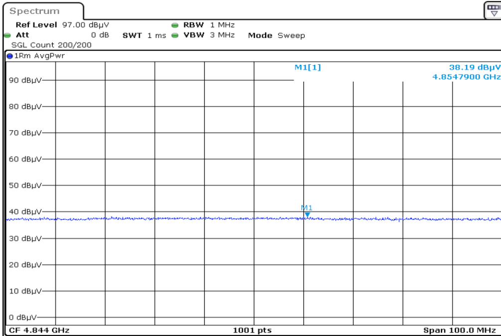
9 F1 X2 4844.0 Harmonic Horizontal AVG
