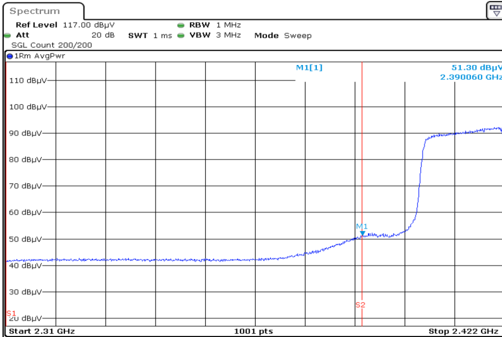
3 2422.0 F1 RestrictedBand Vertical AVG
