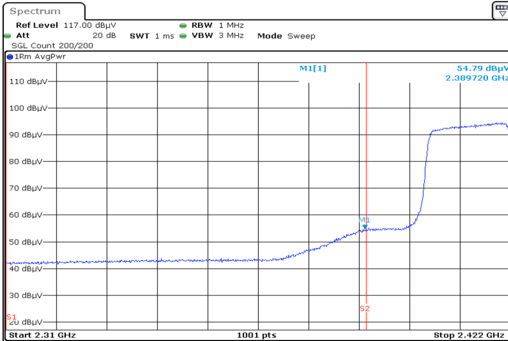
1 2422.0 F1 RestrictedBand Horizontal AVG
