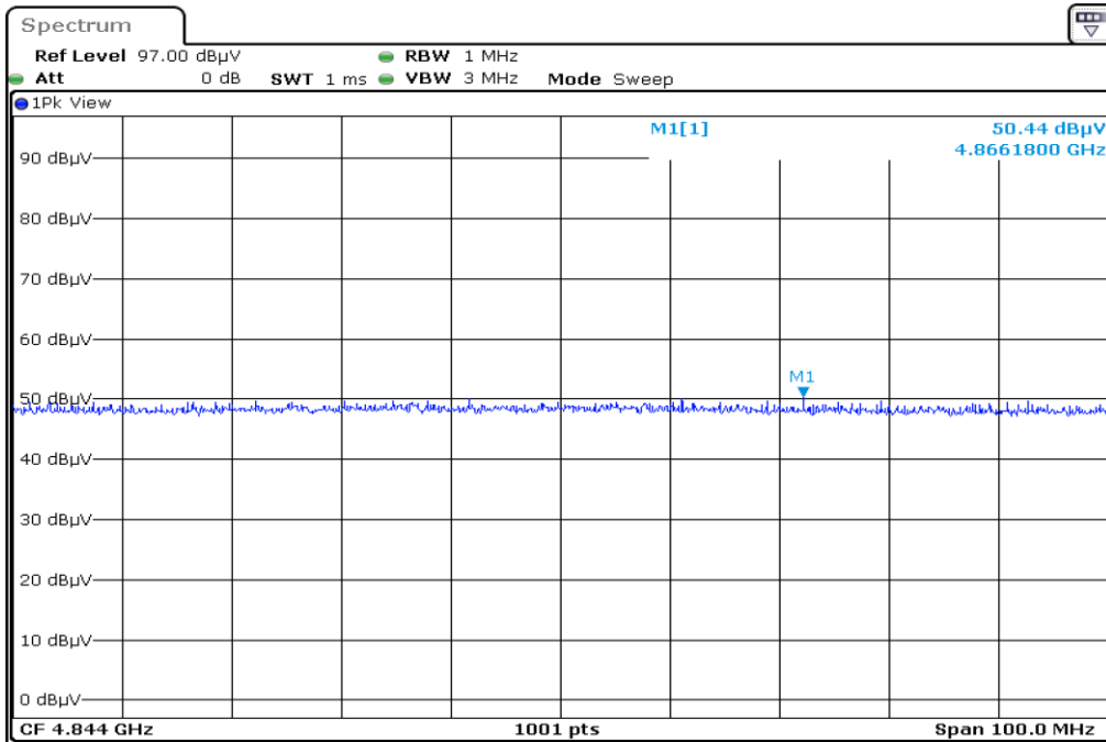
10 F1 X2 4844.0 Harmonic Horizontal PEAK
