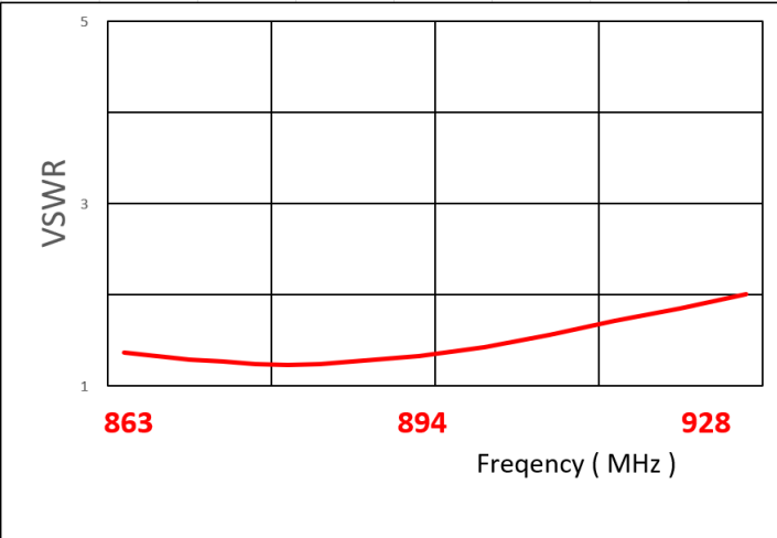
VSWR
