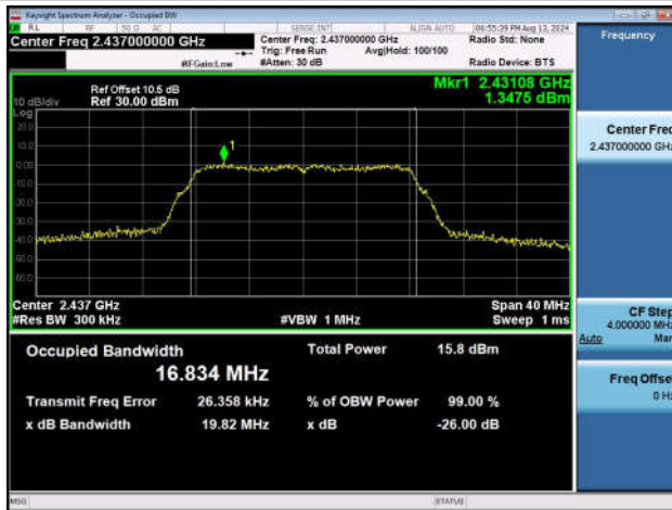
11G-Ant1-2437
