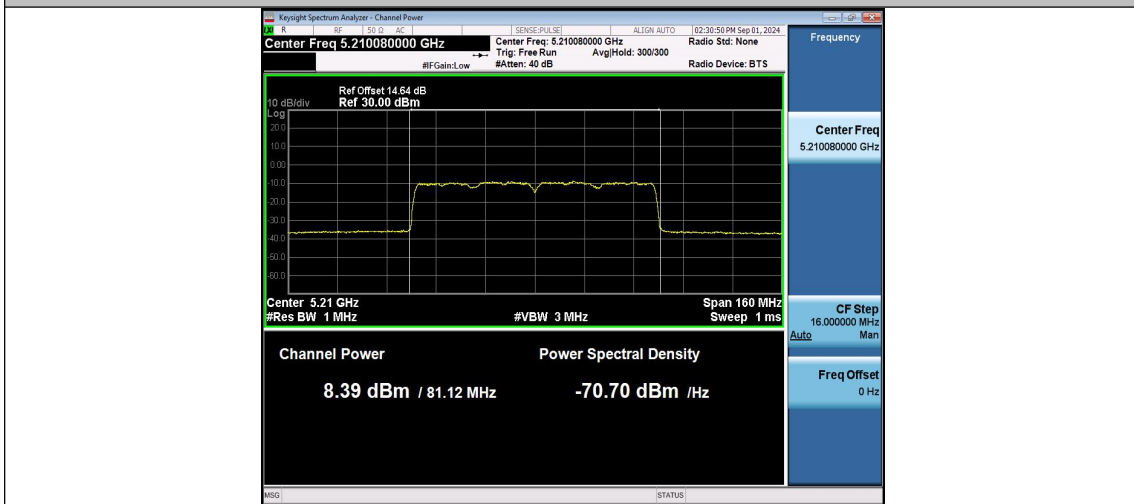
11AX80MIMO-Ant1-5210-PASS
