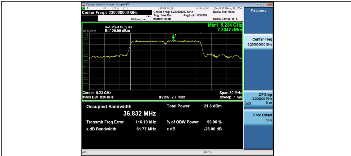
11N40MIMO-Ant2-5230
