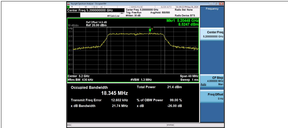
11N20MIMO-Ant2-5200
