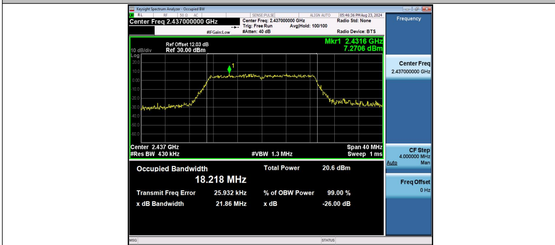
11N20MIMO_Ant2_2437
