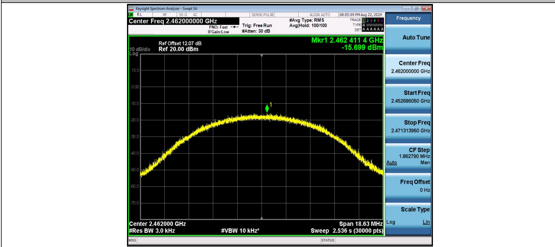
11B_Ant2_2462
