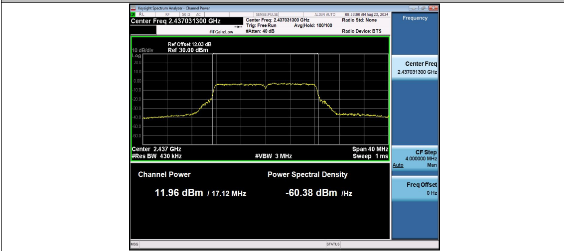
11G_Ant2_2437
