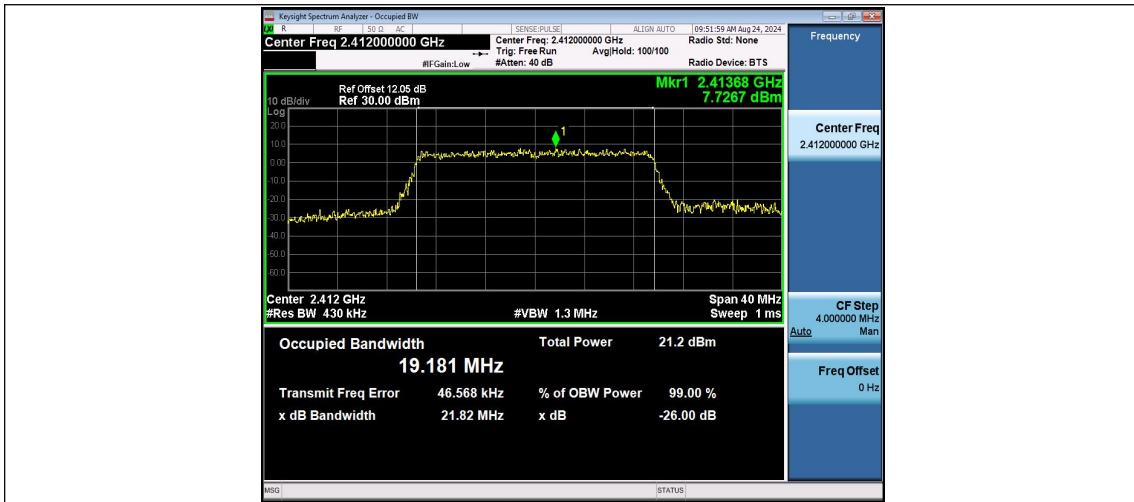
11AX20MIMO_Ant2_2412
