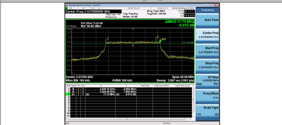
11N20MIMO_Ant2_2437
