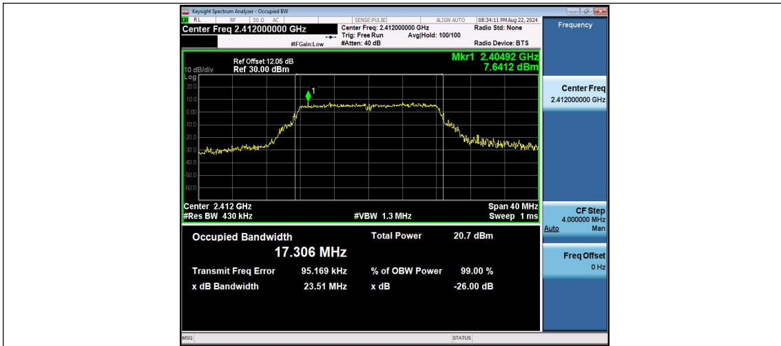
11G_Ant2_2412
