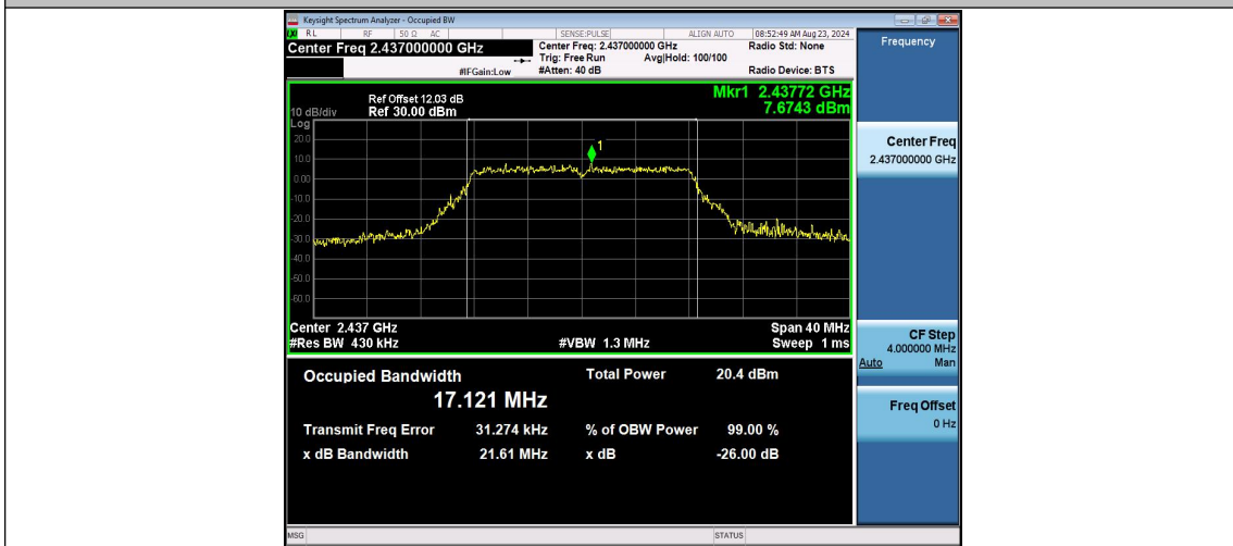
11G_Ant2_2437
