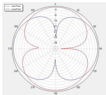
Theta=90 freq=2400MHz
