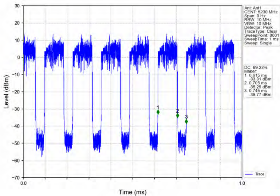
802.11ac(VHT40)_HCH_5230MHz_Ant1_NTNV
