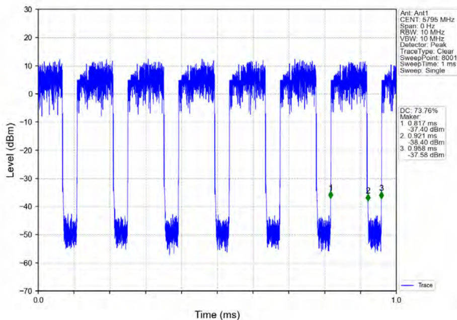
802.11n(HT40)_HCH_5795MHz_Ant1_NTNV
