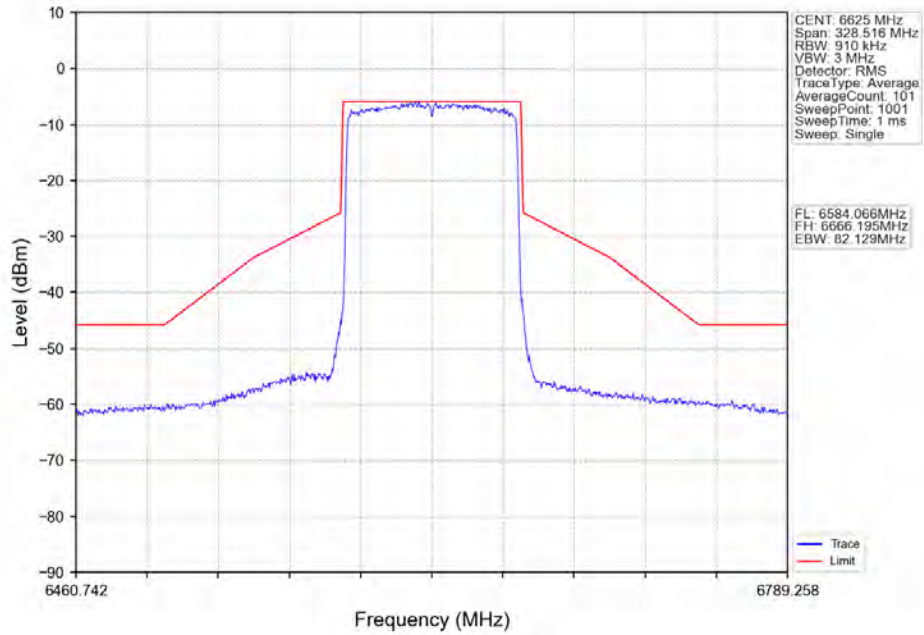
802.11ax(HE80)_LCH_6625MHz_RU996_Left_Ant2_NTNV
