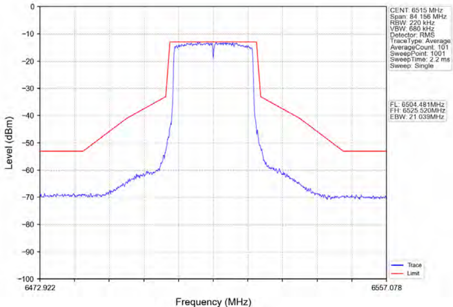
802.11ax(HE20)_HCH_6515MHz_RU242_Left_Ant2_NTNV
