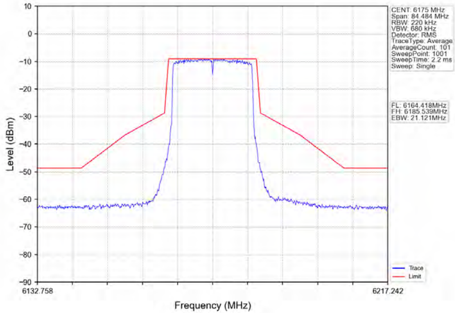
802.11ax(HE20)_MCH_6175MHz_RU242_Left_Ant2_NTNV
