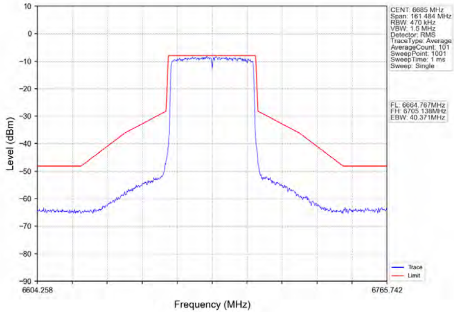
802.11ax(HE40)_MCH_6685MHz_RU484_Left_Ant2_NTNV
