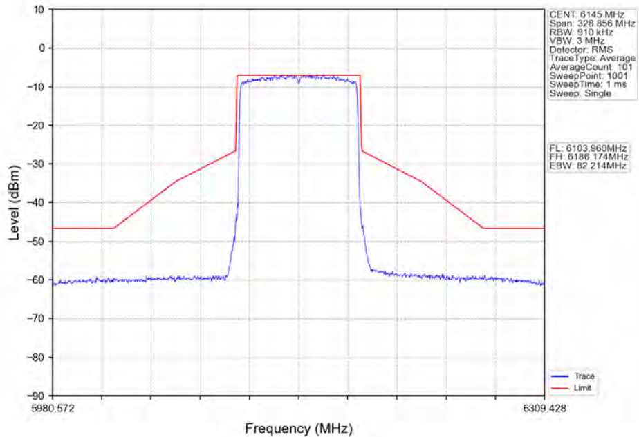
802.11ax(HE80)_MCH_6145MHz_RU996_Left_Ant2_NTNV
