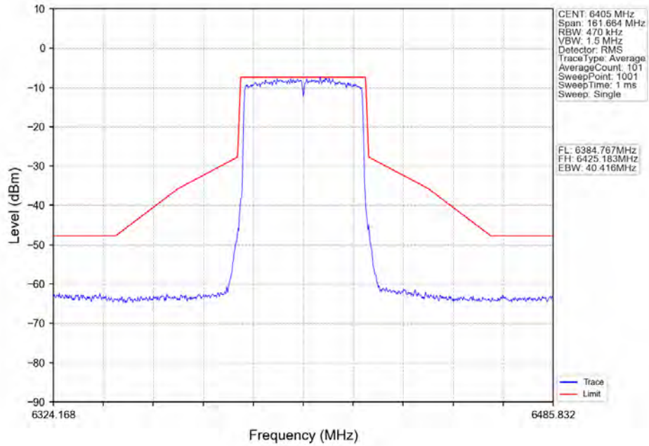
802.11ax(HE40)_HCH_6405MHz_RU484_Left_Ant2_NTNV
