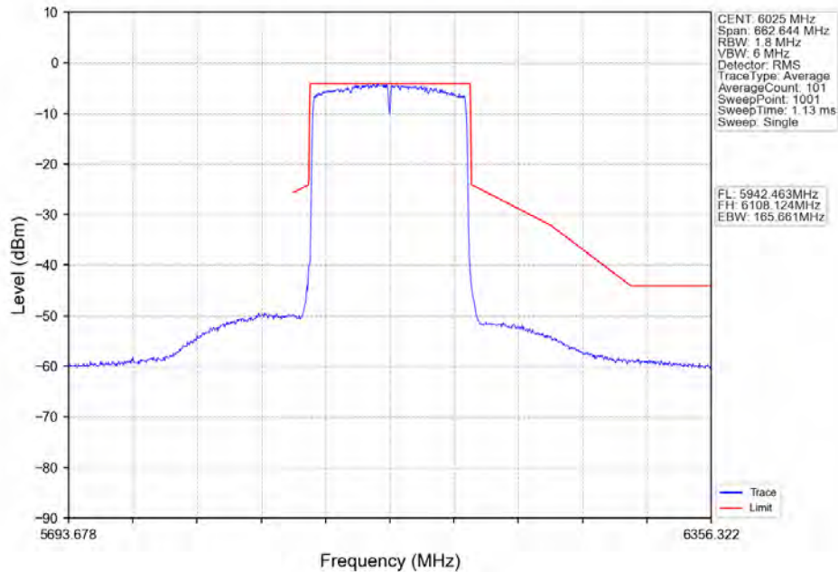
802.11ax(HE160)_LCH_6025MHz_2xRU996_Left_Ant2_NTNV
