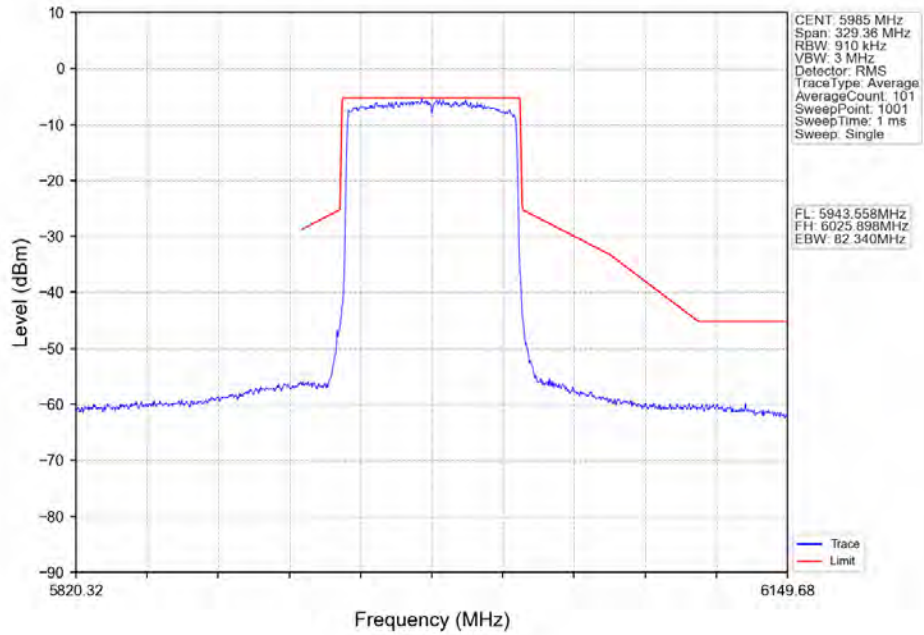
802.11ax(HE80)_LCH_5985MHz_RU996_Left_Ant2_NTNV
