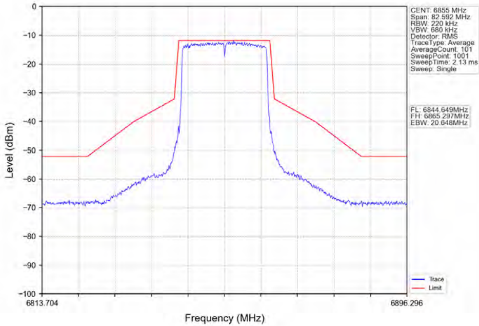
802.11ax(HE20)_HCH_6855MHz_RU242_Left_Ant2_NTNV
