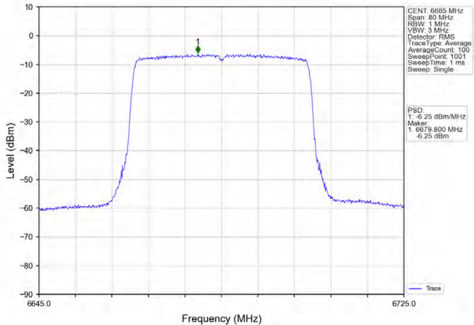
802.11ax(HE40)_MCH_6685MHz_RU484_Left_Ant2_NTNV
