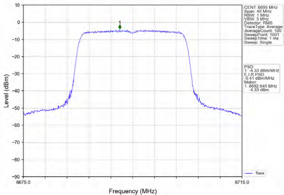
802.11ax(HE20)_MCH_6695MHz_RU242_Left_Ant1_NTNV
