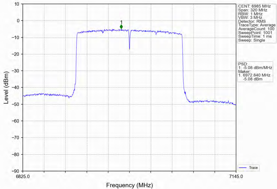
802.11ax(HE160)_MCH_6985MHz_2xRU996_Left_Ant2_NTNV
