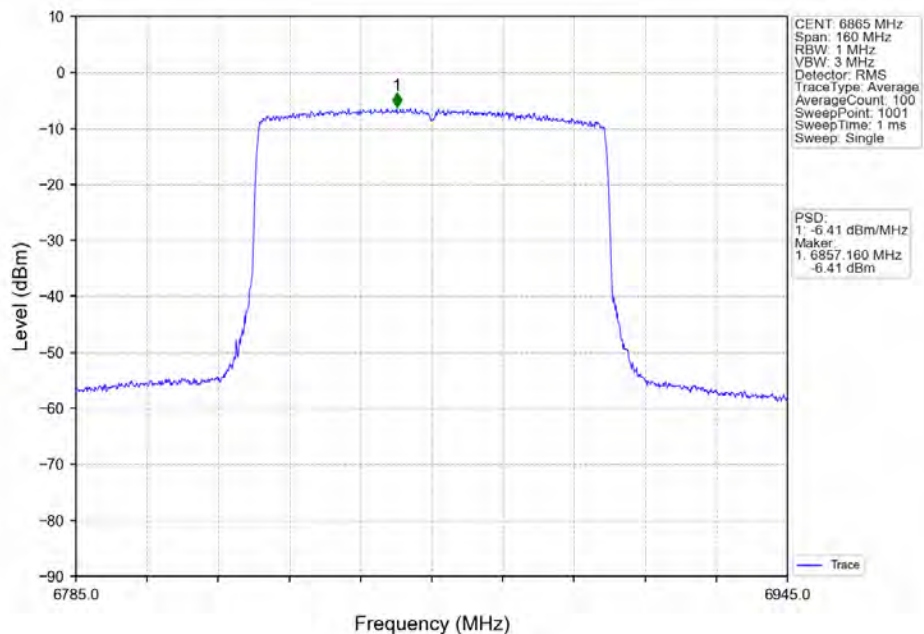
802.11ax(HE80)_HCH_6865MHz_RU996_Left_Ant2_NTNV
