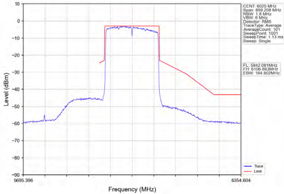
802.11ax(HE160)_LCH_6025MHz_2xRU996_Left_Ant2_NTNV
