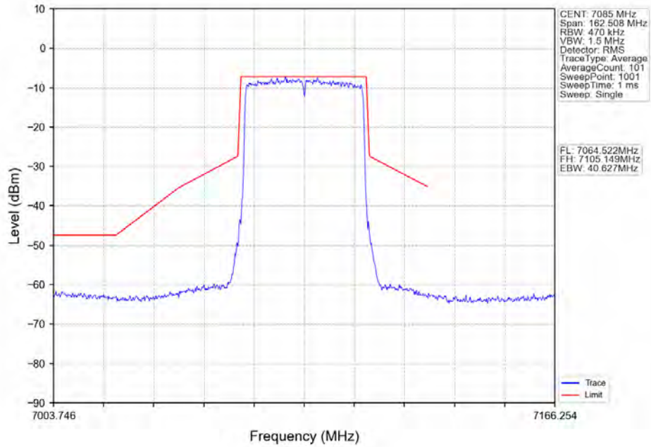
802.11ax(HE40)_HCH_7085MHz_RU484_Left_Ant2_NTNV
