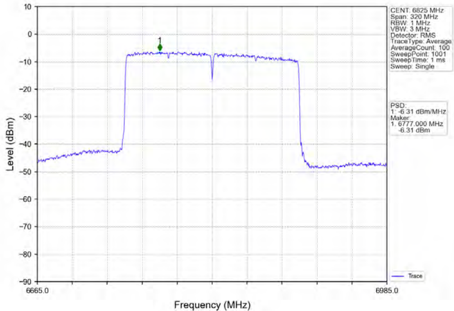
802.11ax(HE160)_HCH_6825MHz_2xRU996_Left_Ant1_NTNV
