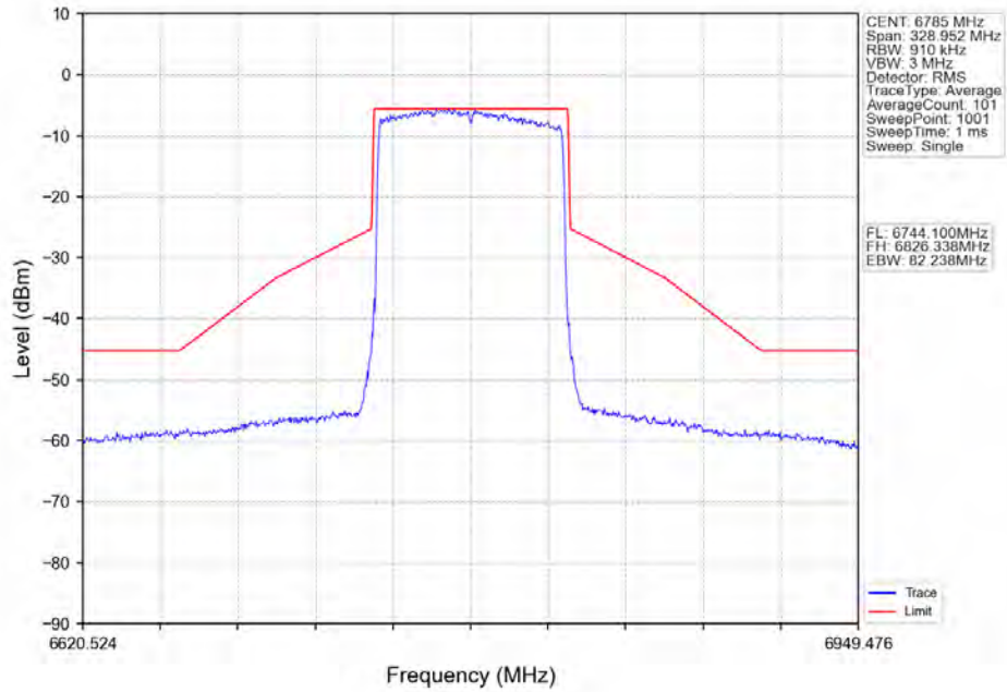
802.11ax(HE80)_HCH_6785MHz_RU996_Left_Ant2_NTNV
