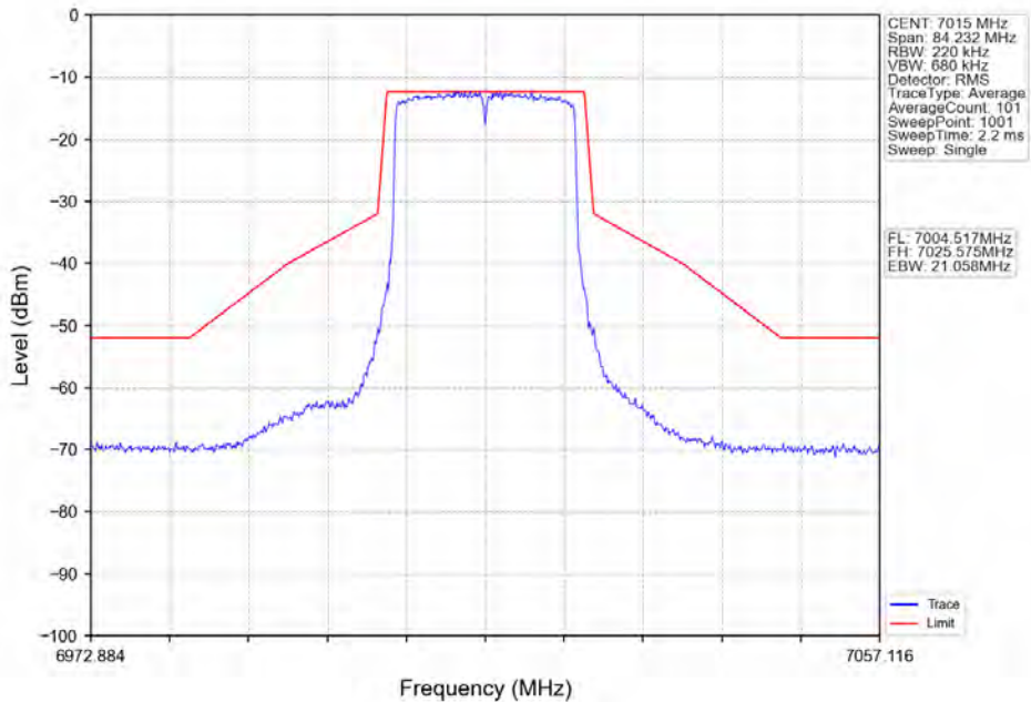
802.11ax(HE20)_MCH_7015MHz_RU242_Left_Ant2_NTNV
