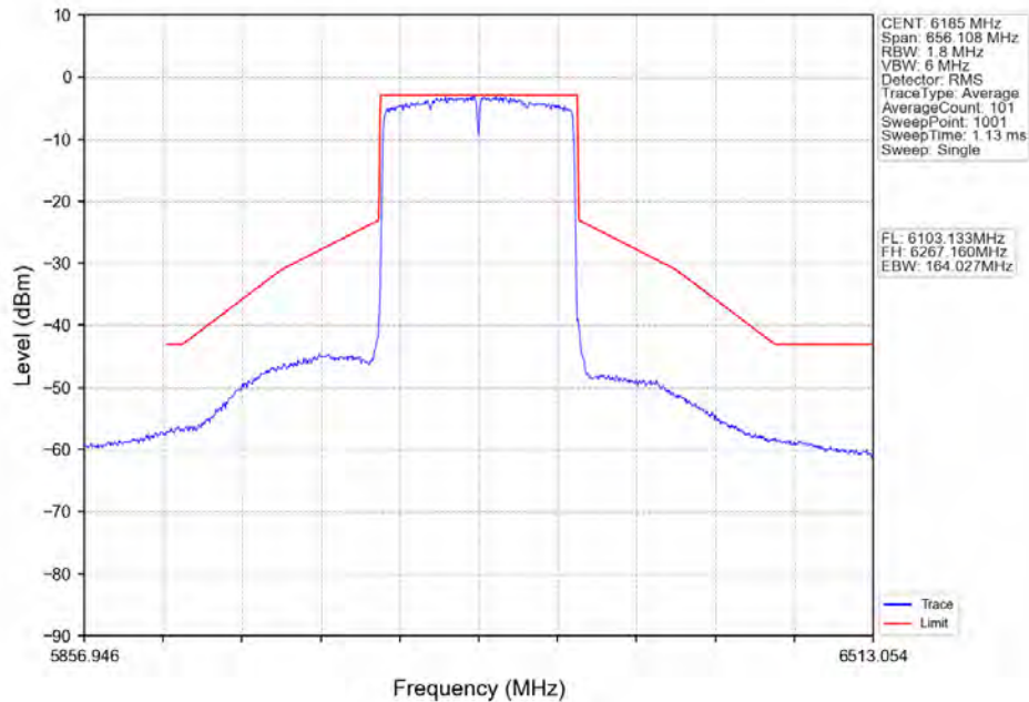
802.11ax(HE160)_MCH_6185MHz_2xRU996_Left_Ant2_NTNV
