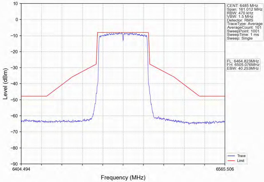
802.11ax(HE40)_MCH_6485MHz_RU484_Left_Ant2_NTNV
