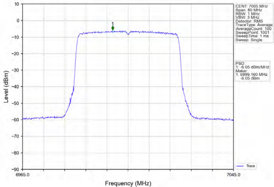
802.11ax(HE40)_MCH_7005MHz_RU484_Left_Ant2_NTNV
