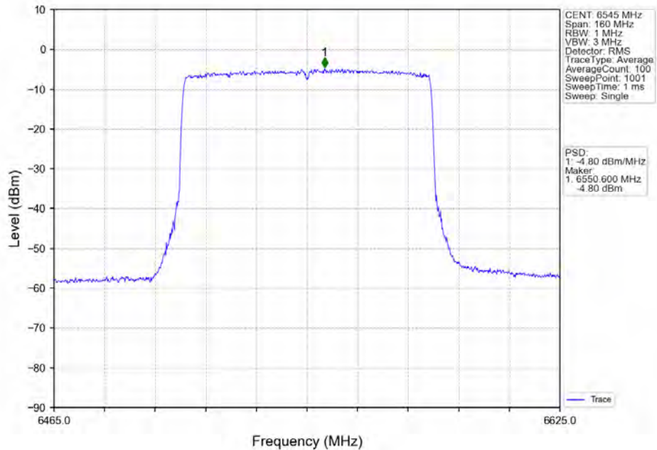
802.11ax(HE80)_HCH_6545MHz_RU996_Left_Ant1_NTNV
