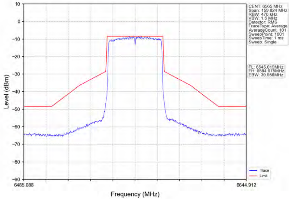
802.11ax(HE40)_LCH_6565MHz_RU484_Left_Ant2_NTNV
