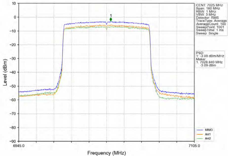
802.11ax(HE80)_HCH_7025MHz_RU996_Left_MIMO_NTNV
