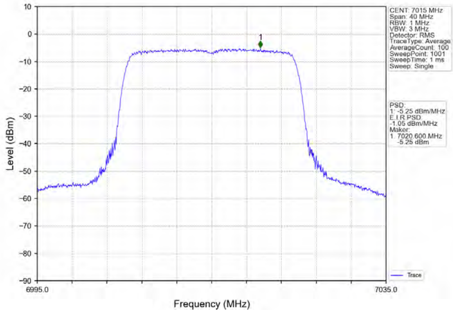
802.11ax(HE20)_MCH_7015MHz_RU242_Left_Ant1_NTNV
