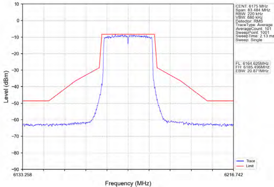
802.11ax(HE20)_MCH_6175MHz_RU242_Left_Ant2_NTNV
