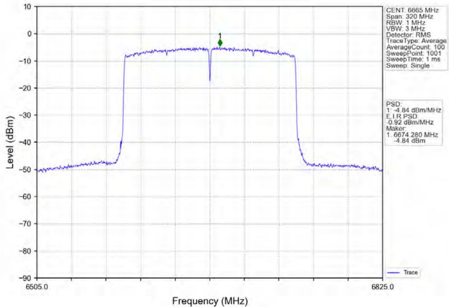
802.11ax(HE160)_MCH_6665MHz_2xRU996_Left_Ant1_NTNV
