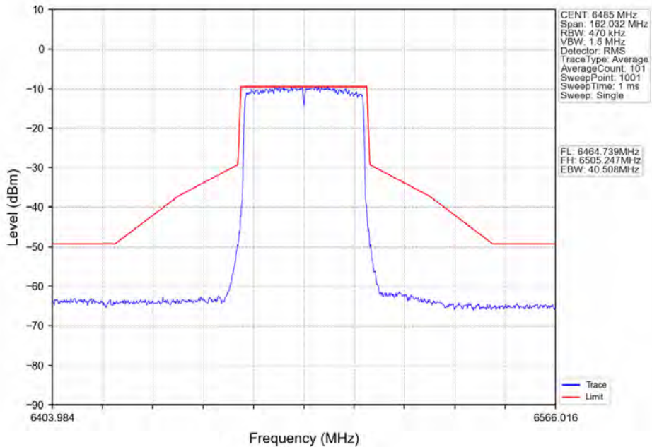
802.11ax(HE40)_MCH_6485MHz_RU484_Left_Ant2_NTNV
