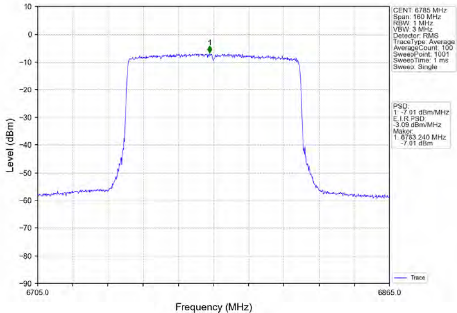
802.11ax(HE80)_HCH_6785MHz_RU996_Left_Ant2_NTNV
