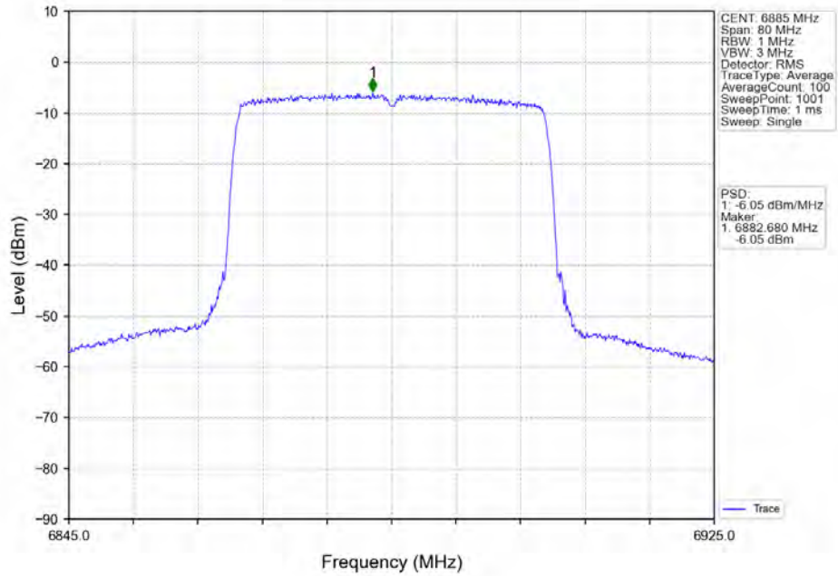
802.11ax(HE40)_HCH_6885MHz_RU484_Left_MIMO_NTNV
