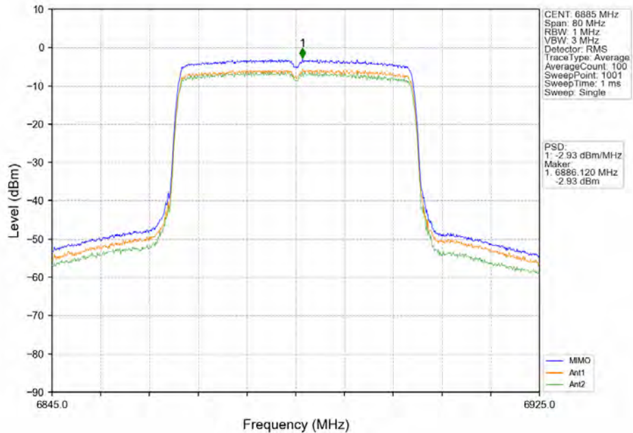
802.11ax(HE40)_HCH_6885MHz_RU484_Left_MIMO_NTNV
