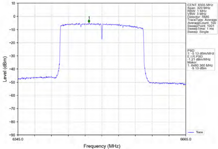
802.11ax(HE160)_HCH_6505MHz_2xRU996_Left_Ant2_NTNV
