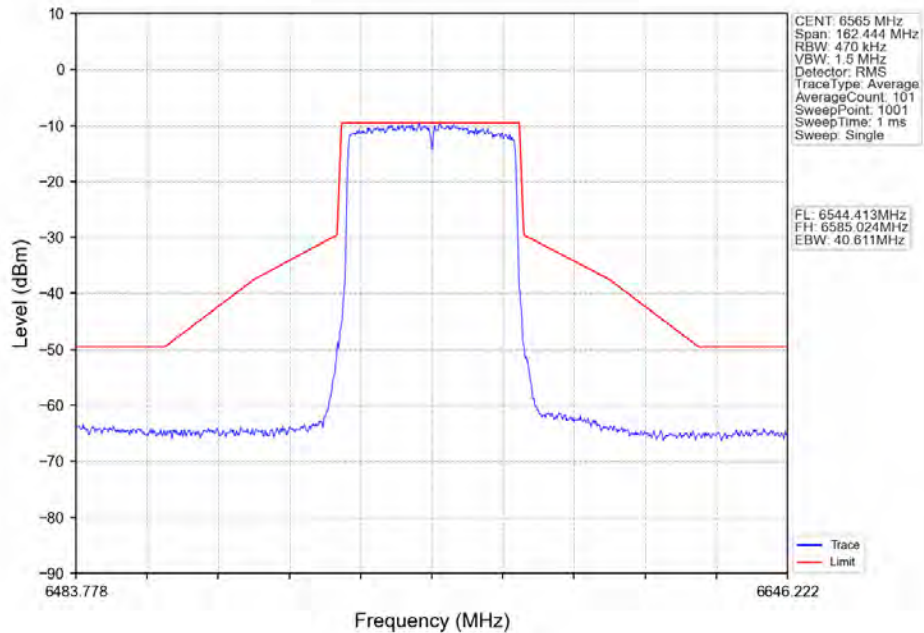
802.11ax(HE40)_LCH_6565MHz_RU484_Left_Ant2_NTNV
