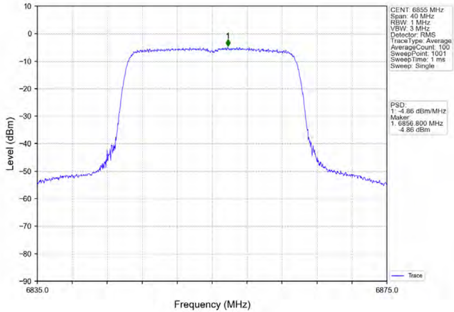
802.11ax(HE20)_HCH_6855MHz_RU242_Left_Ant2_NTNV
