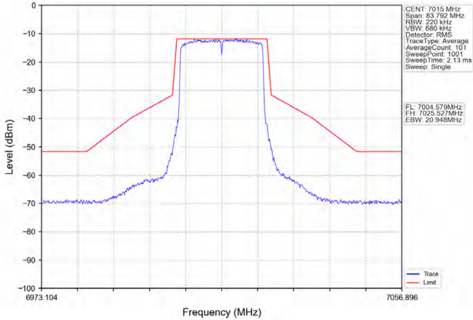
802.11ax(HE20)_MCH_7015MHz_RU242_Left_Ant2_NTNV
