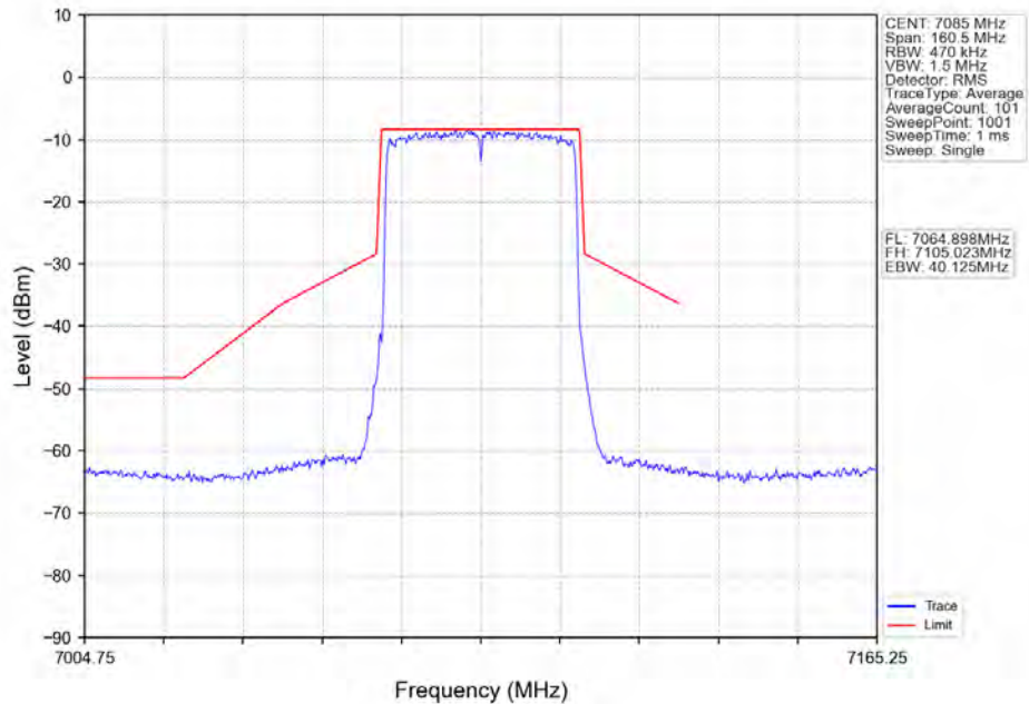
802.11ax(HE40)_HCH_7085MHz_RU484_Left_Ant2_NTNV
