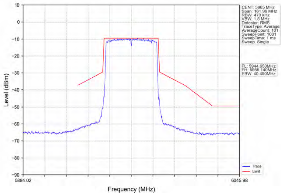
802.11ax(HE40)_LCH_5965MHz_RU484_Left_Ant2_NTNV
