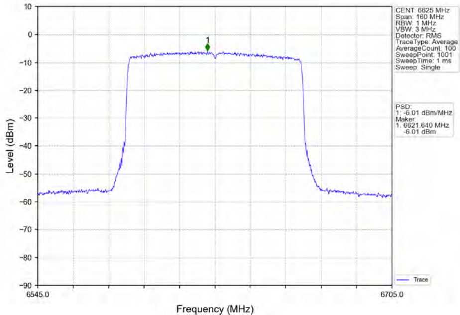
802.11ax(HE80)_LCH_6625MHz_RU996_Left_Ant2_NTNV
