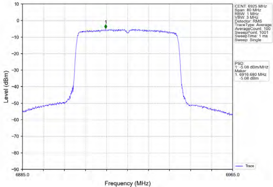
802.11ax(HE40)_LCH_6925MHz_RU484_Left_Ant1_NTNV
