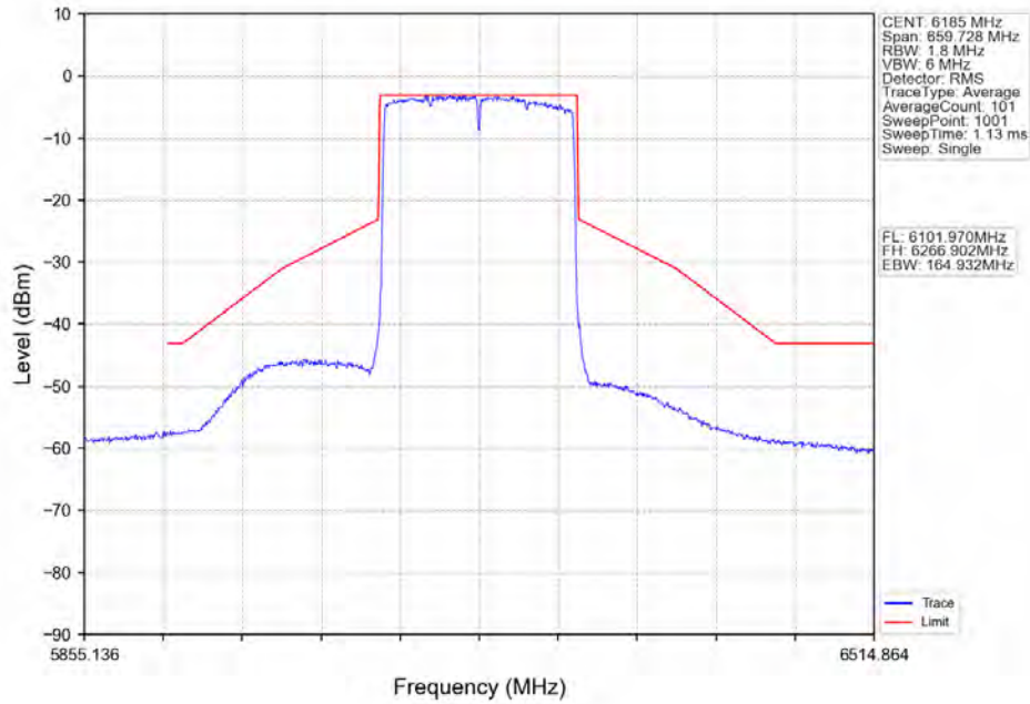
802.11ax(HE160)_MCH_6185MHz_2xRU996_Left_Ant2_NTNV
