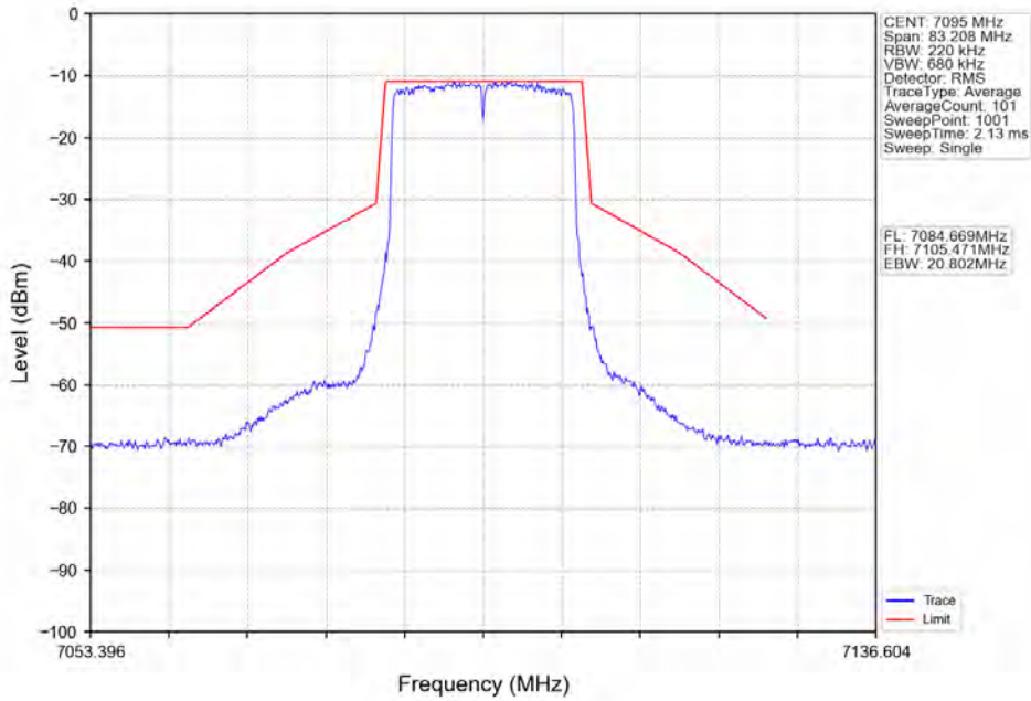
802.11ax(HE20)_HCH_7095MHz_RU242_Left_Ant2_NTNV
