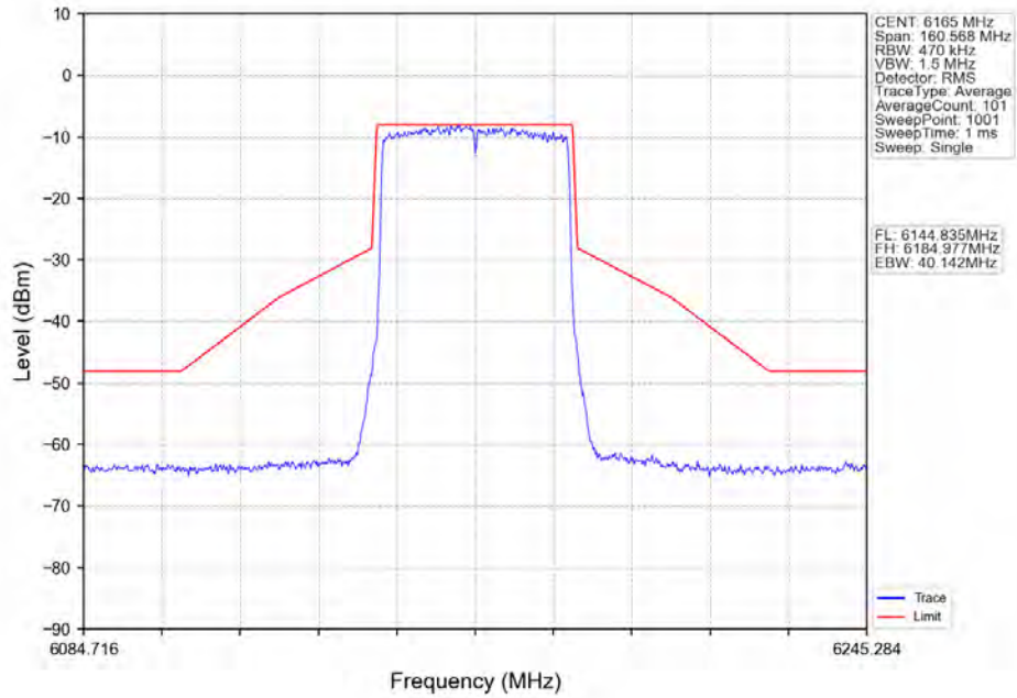
802.11ax(HE40)_MCH_6165MHz_RU484_Left_Ant2_NTNV
