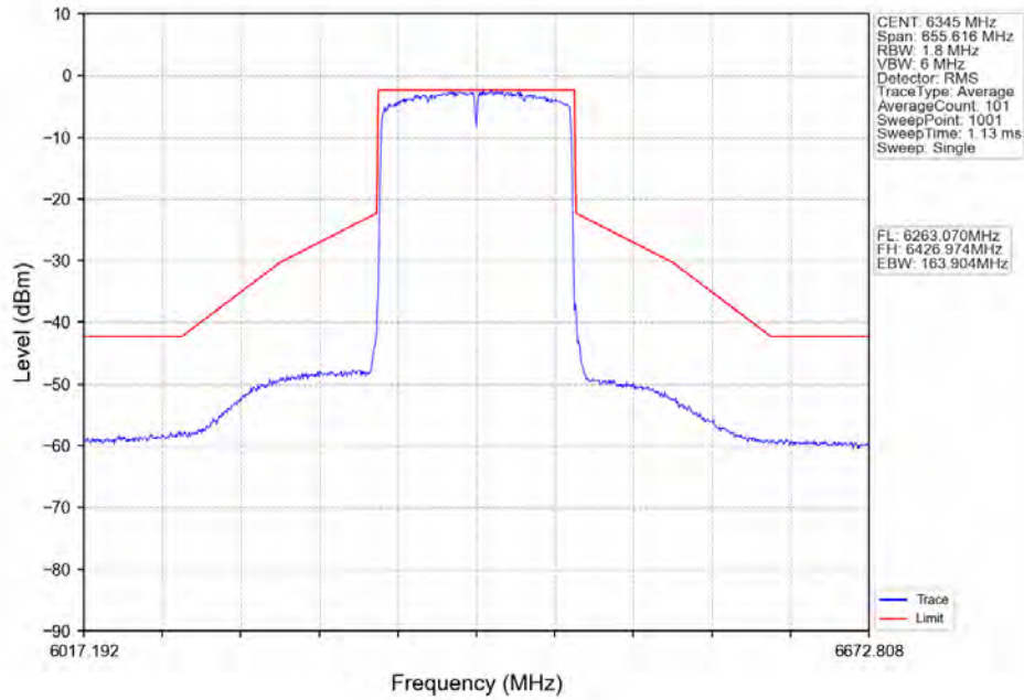
802.11ax(HE160)_HCH_6345MHz_2xRU996_Left_Ant2_NTNV
