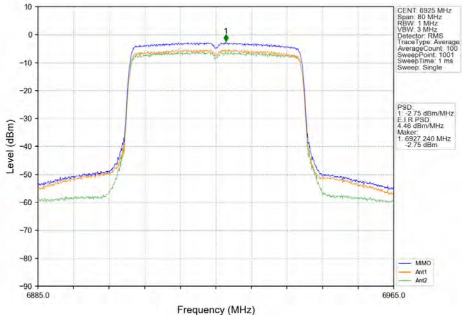
802.11ax(HE40)_LCH_6925MHz_RU484_Left_MIMO_NTNV
