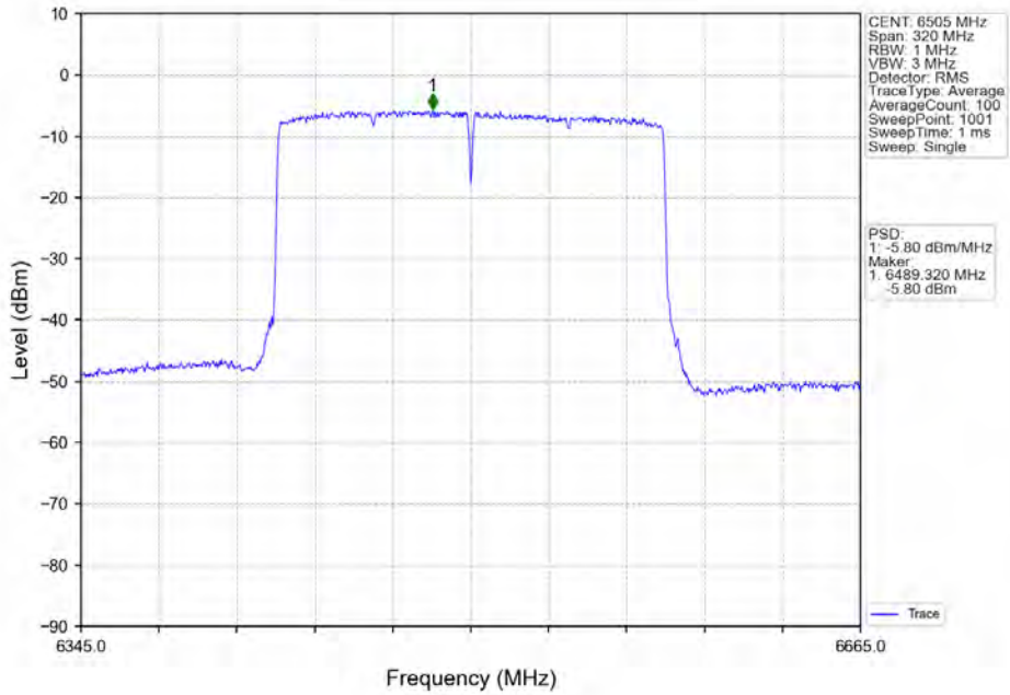
802.11ax(HE160)_HCH_6505MHz_2xRU996_Left_Ant2_NTNV
