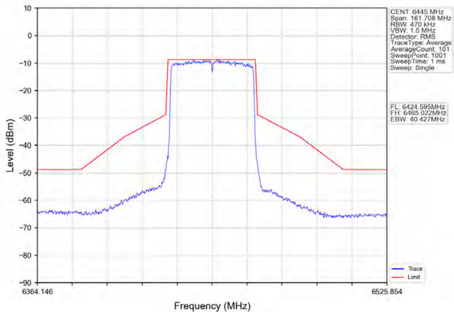
802.11ax(HE40)_LCH_6445MHz_RU484_Left_Ant2_NTNV
