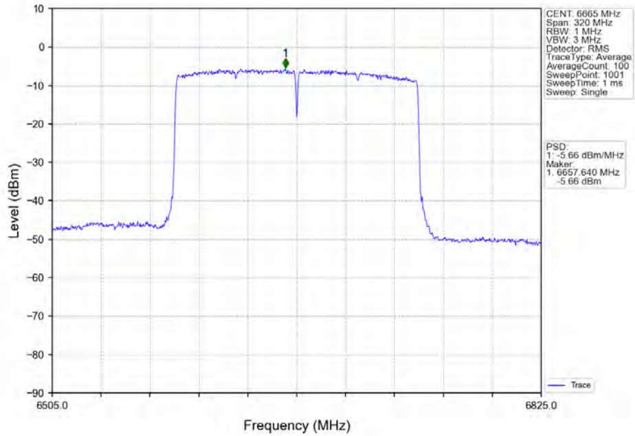
802.11ax(HE160)_MCH_6665MHz_2xRU996_Left_MIMO_NTNV
