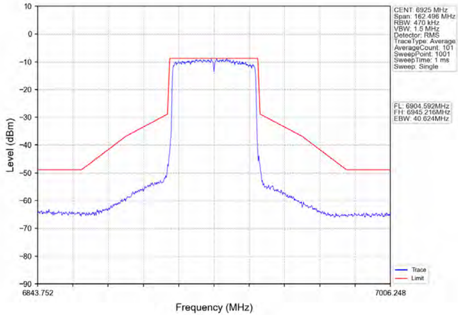
802.11ax(HE40)_LCH_6925MHz_RU484_Left_Ant2_NTNV
