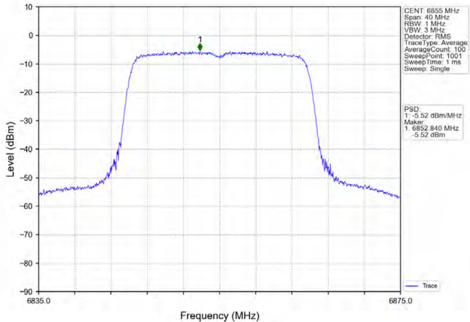
802.11ax(HE20)_HCH_6855MHz_RU242_Left_Ant2_NTNV
