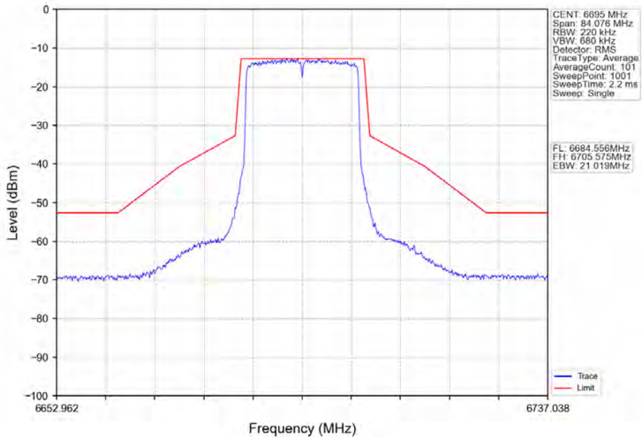
802.11ax(HE20)_MCH_6695MHz_RU242_Left_Ant2_NTNV
