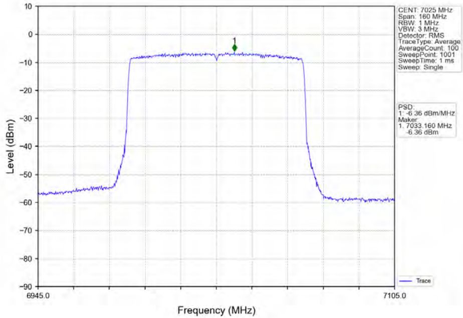
802.11ax(HE80)_HCH_7025MHz_RU996_Left_MIMO_NTNV
