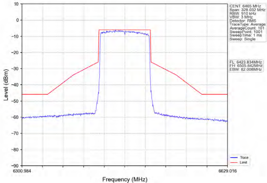
802.11ax(HE80)_LCH_6465MHz_RU996_Left_Ant2_NTNV
