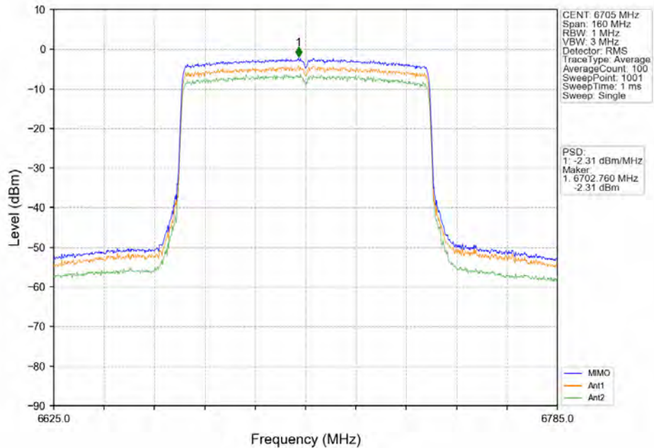
802.11ax(HE80)_MCH_6705MHz_RU996_Left_MIMO_NTNV
