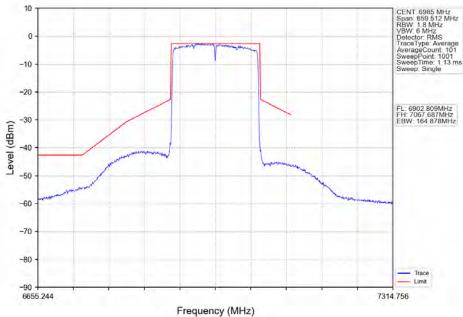
802.11ax(HE160)_MCH_6985MHz_2xRU996_Left_Ant2_NTNV
