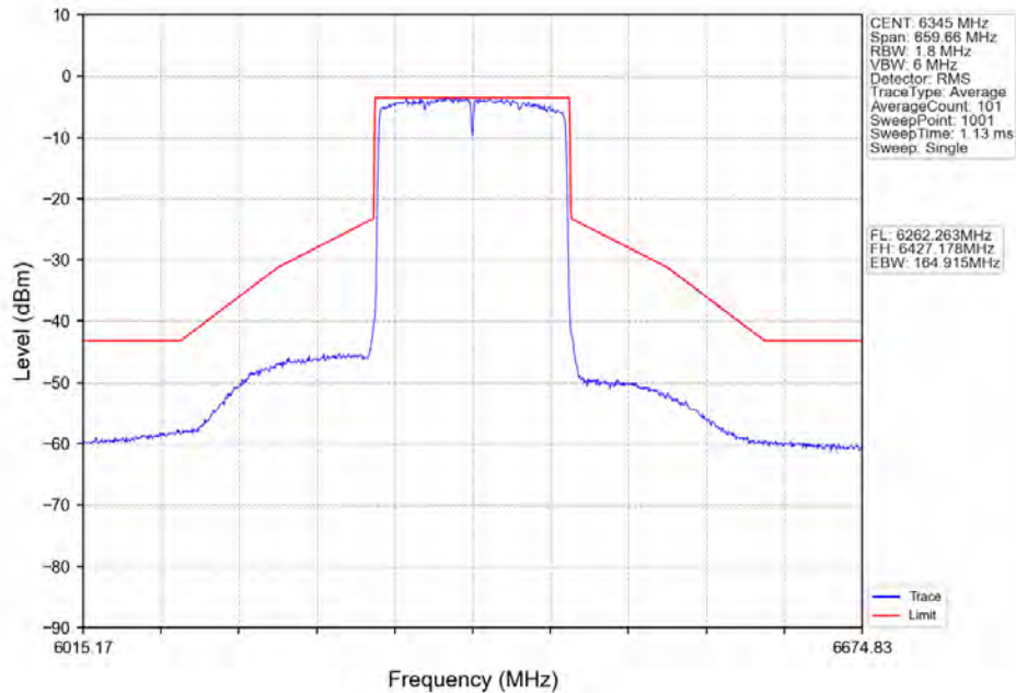
802.11ax(HE160)_HCH_6345MHz_2xRU996_Left_Ant2_NTNV
