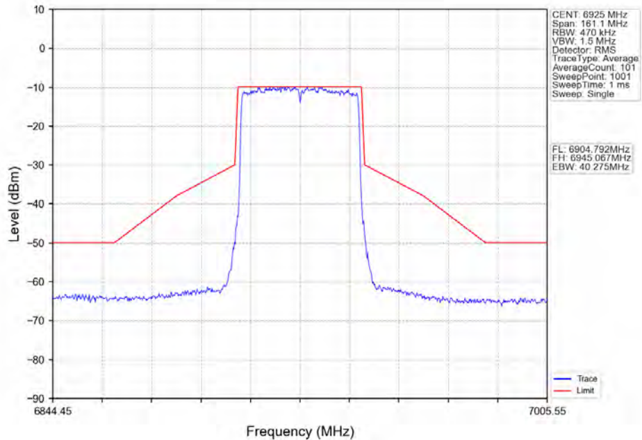
802.11ax(HE40)_LCH_6925MHz_RU484_Left_Ant2_NTNV
