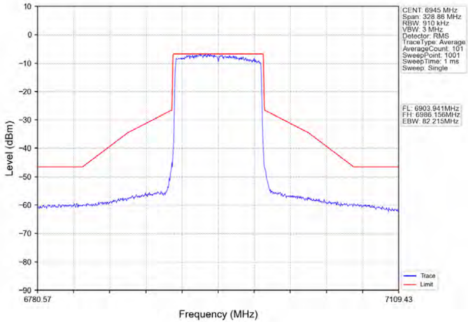
802.11ax(HE80)_LCH_6945MHz_RU996_Left_Ant2_NTNV
