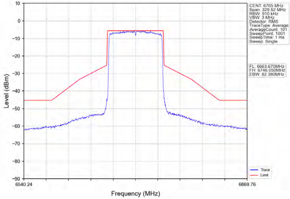
802.11ax(HE80)_MCH_6705MHz_RU996_Left_Ant2_NTNV
