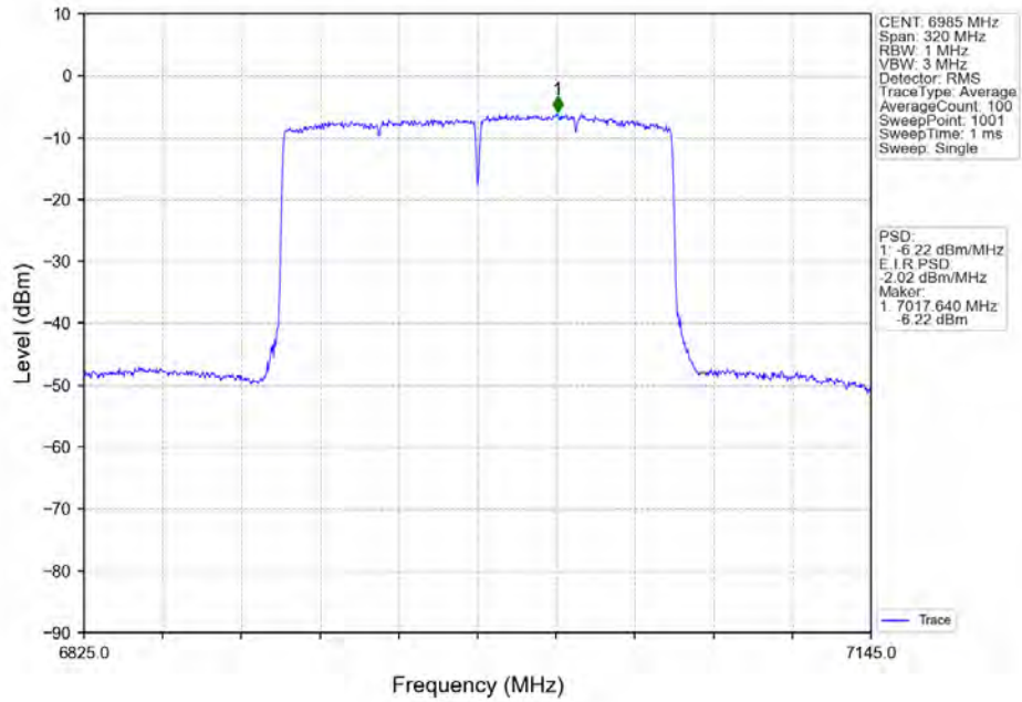
802.11ax(HE160)_MCH_6985MHz_2xRU996_Left_Ant2_NTNV
