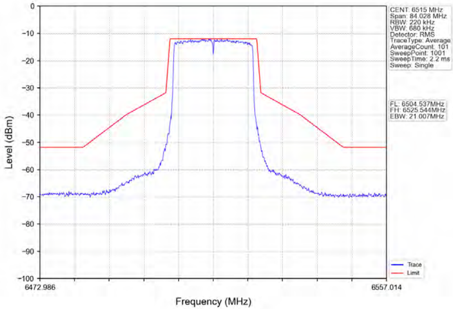
802.11ax(HE20)_HCH_6515MHz_RU242_Left_Ant2_NTNV
