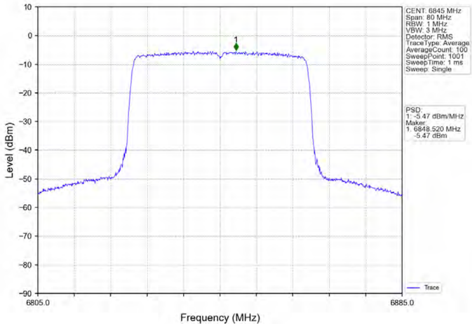
802.11ax(HE40)_HCH_6845MHz_RU484_Left_Ant1_NTNV
