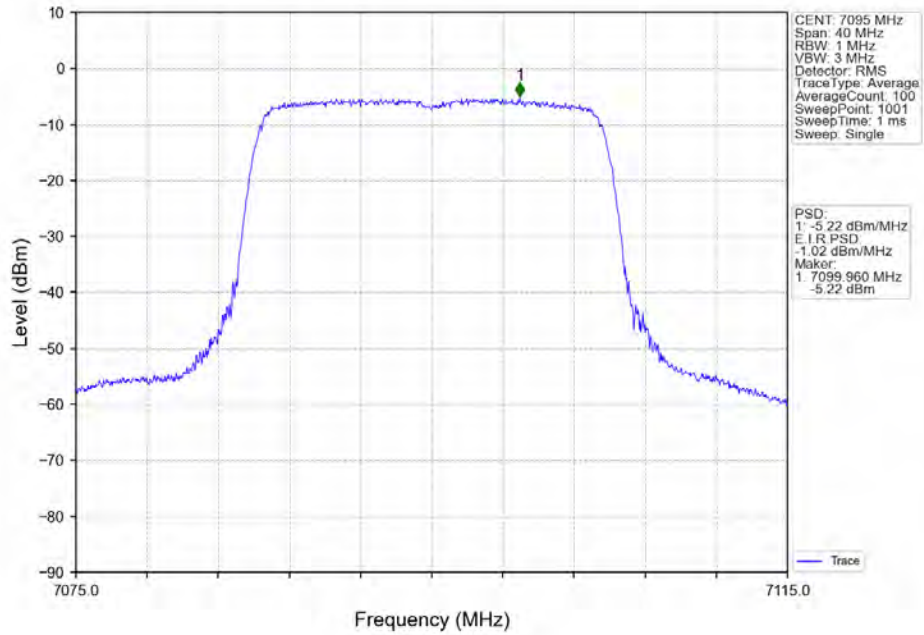
802.11ax(HE20)_HCH_7095MHz_RU242_Left_Ant2_NTNV
