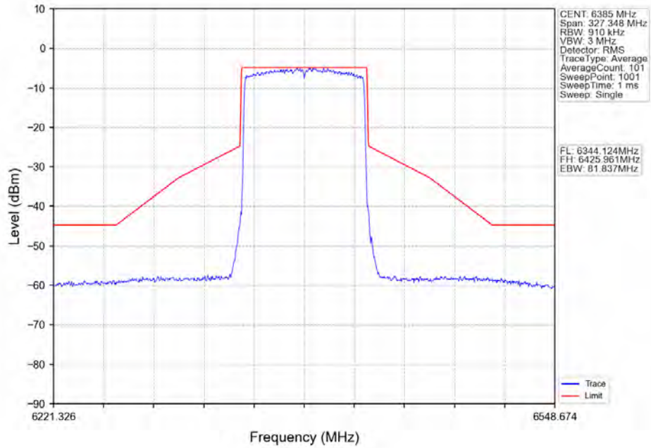
802.11ax(HE80)_HCH_6385MHz_RU996_Left_Ant2_NTNV
