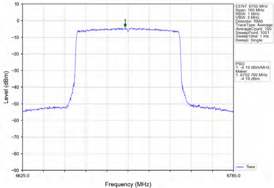
802.11ax(HE80)_MCH_6705MHz_RU996_Left_Ant1_NTNV
