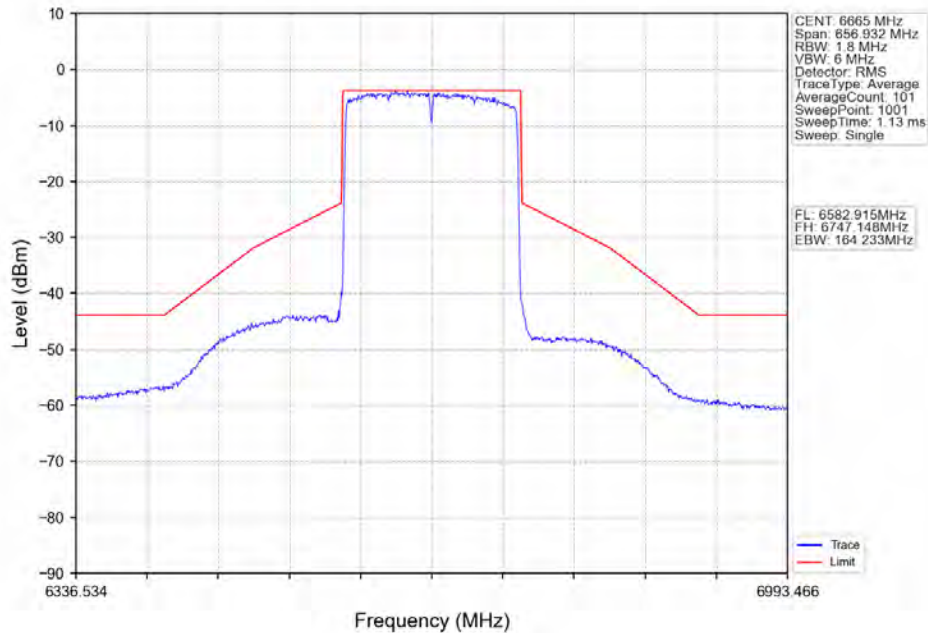
802.11ax(HE160)_MCH_6665MHz_2xRU996_Left_Ant2_NTNV
