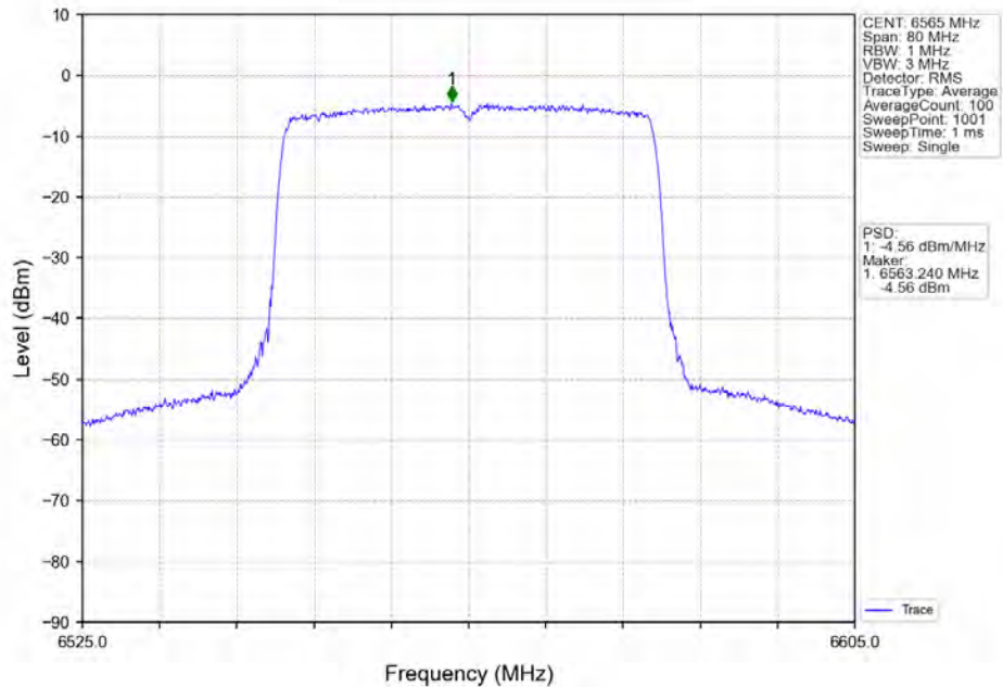
802.11ax(HE40)_LCH_6565MHz_RU484_Left_Ant1_NTNV
