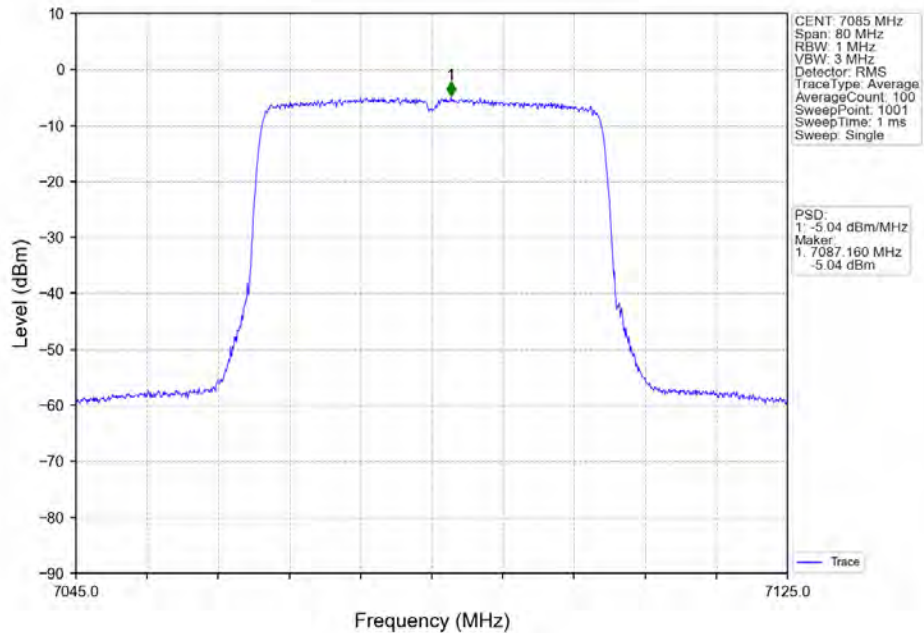
802.11ax(HE40)_HCH_7085MHz_RU484_Left_Ant1_NTNV
