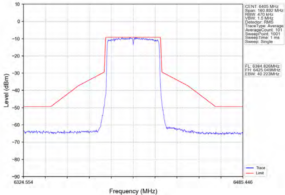
802.11ax(HE40)_HCH_6405MHz_RU484_Left_Ant2_NTNV
