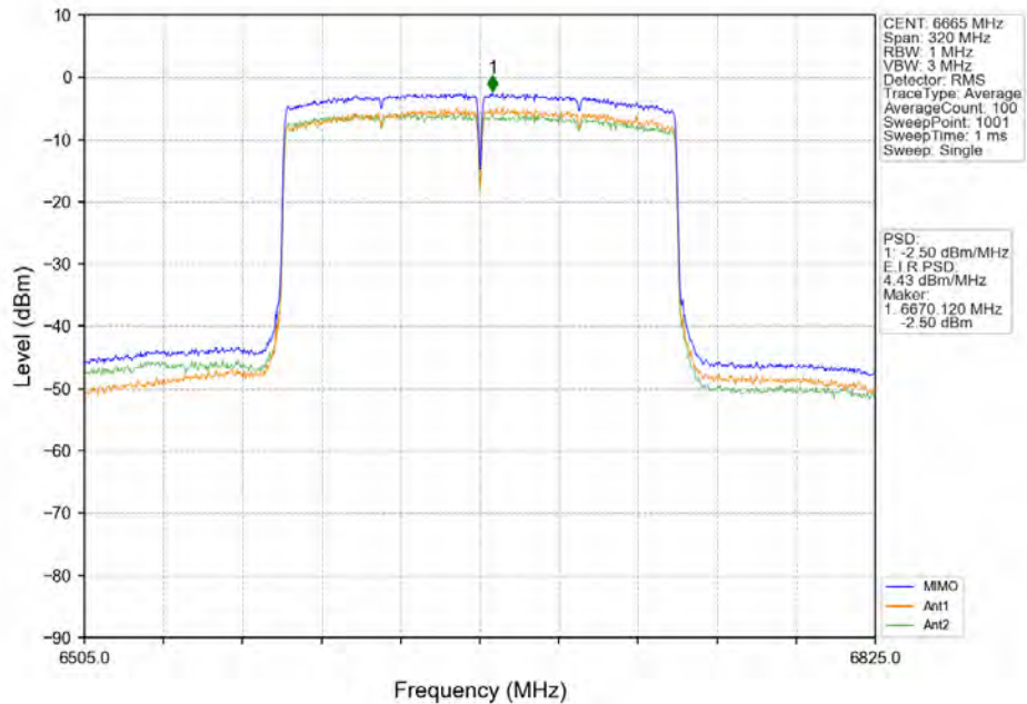
802.11ax(HE160)_MCH_6665MHz_2xRU996_Left_MIMO_NTNV
