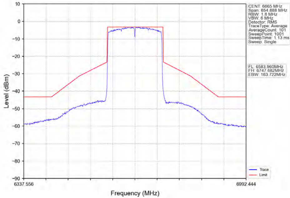
802.11ax(HE160)_MCH_6665MHz_2xRU996_Left_Ant2_NTNV
