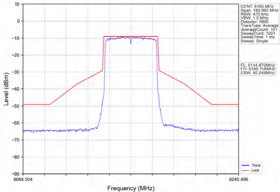
802.11ax(HE40)_MCH_6165MHz_RU484_Left_Ant2_NTNV
