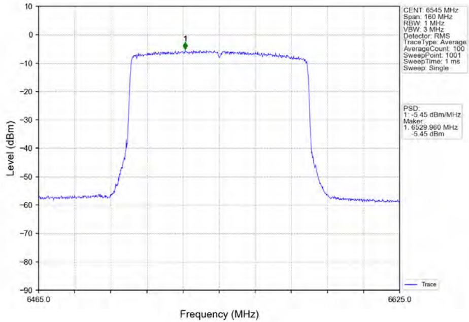
802.11ax(HE80)_HCH_6545MHz_RU996_Left_MIMO_NTNV
