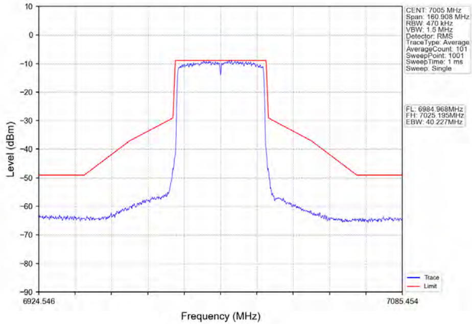
802.11ax(HE40)_MCH_7005MHz_RU484_Left_Ant2_NTNV
