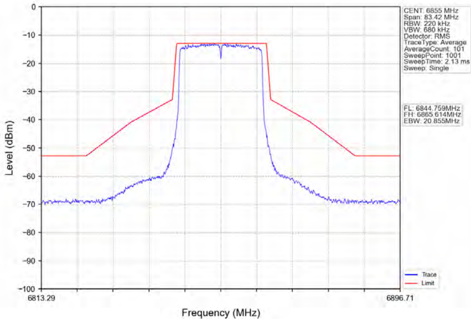
802.11ax(HE20)_HCH_6855MHz_RU242_Left_Ant2_NTNV
