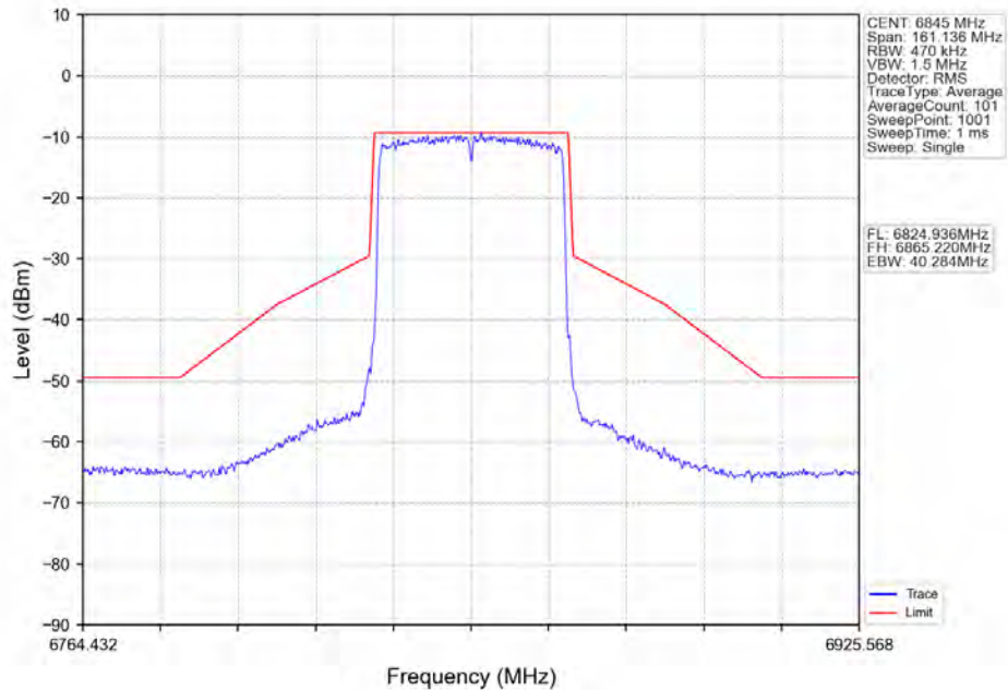
802.11ax(HE40)_HCH_6845MHz_RU484_Left_Ant2_NTNV
