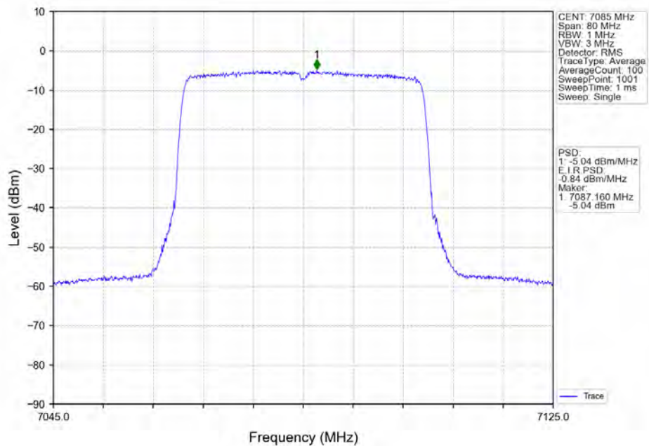
802.11ax(HE40)_HCH_7085MHz_RU484_Left_Ant1_NTNV
