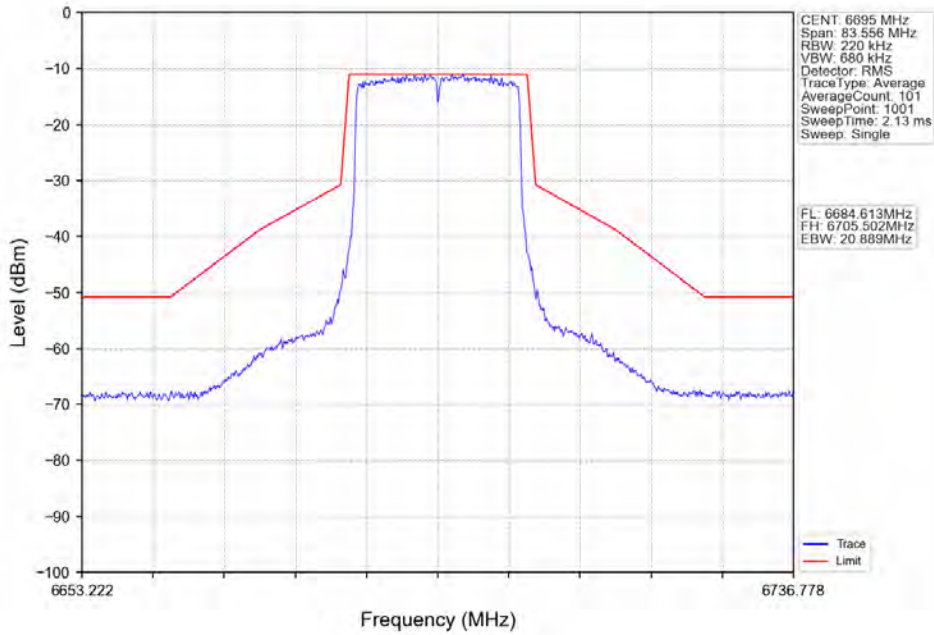
802.11ax(HE20)_MCH_6695MHz_RU242_Left_Ant2_NTNV
