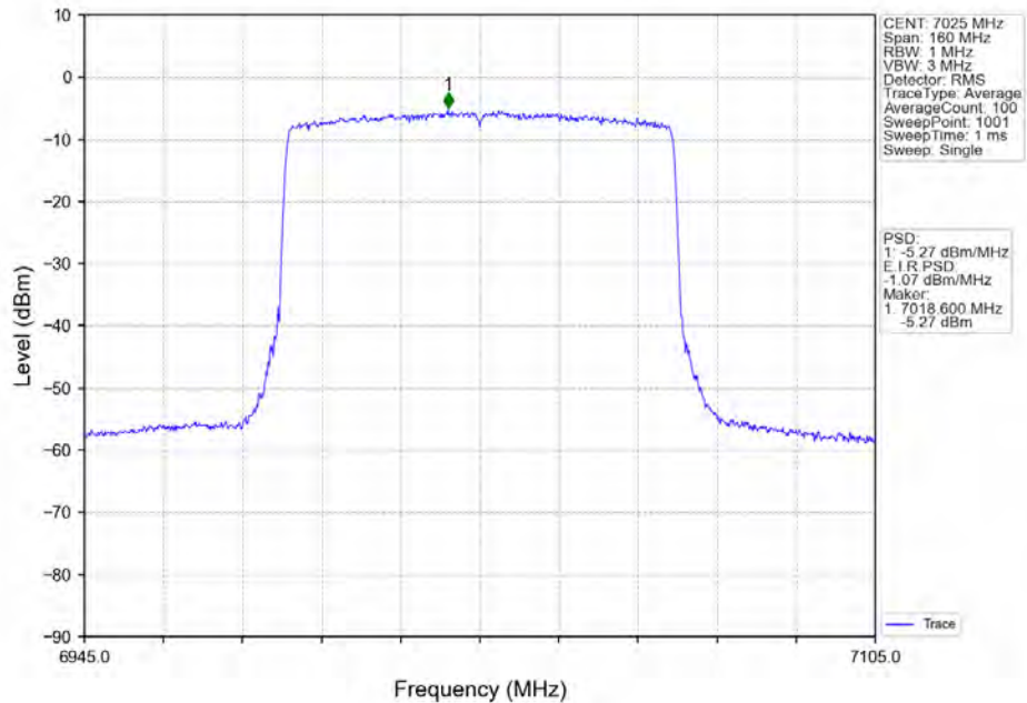
802.11ax(HE80)_HCH_7025MHz_RU996_Left_Ant1_NTNV
