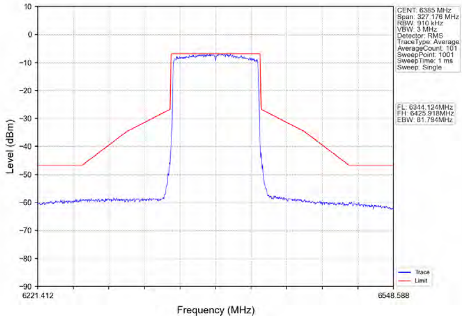
802.11ax(HE80)_HCH_6385MHz_RU996_Left_Ant2_NTNV
