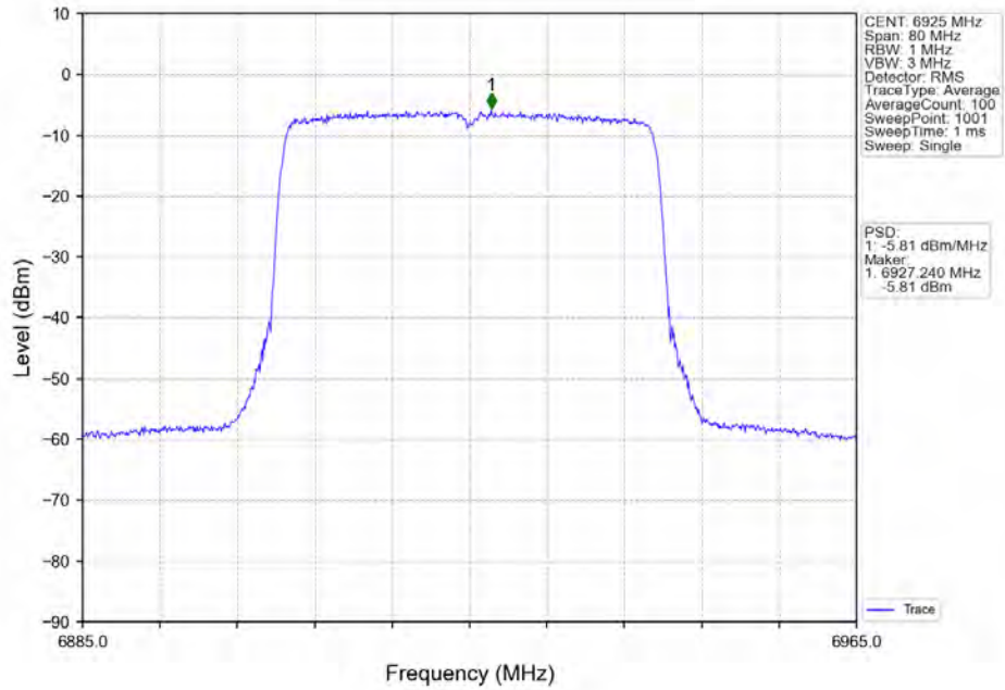
802.11ax(HE40)_LCH_6925MHz_RU484_Left_MIMO_NTNV
