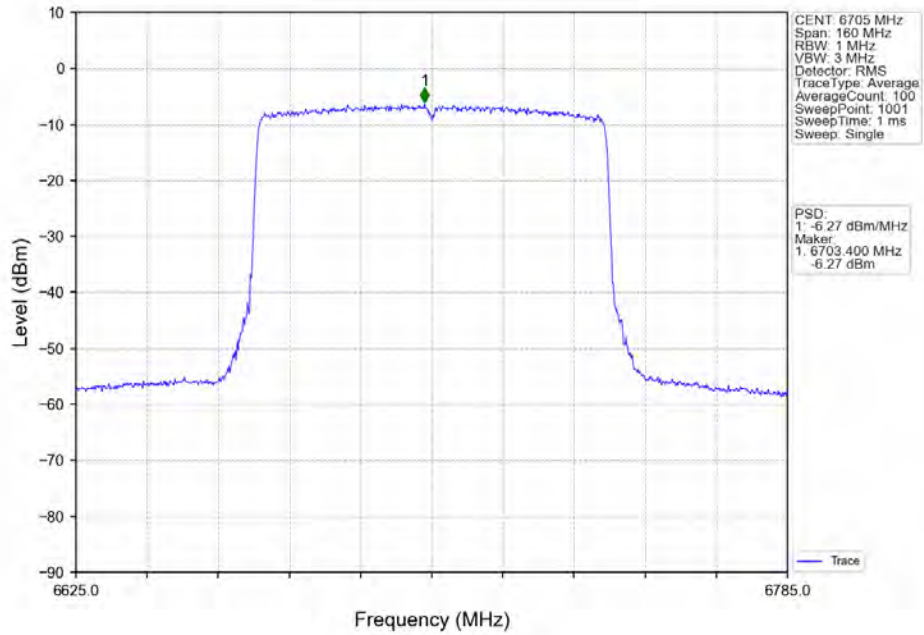
802.11ax(HE80)_MCH_6705MHz_RU996_Left_MIMO_NTNV
