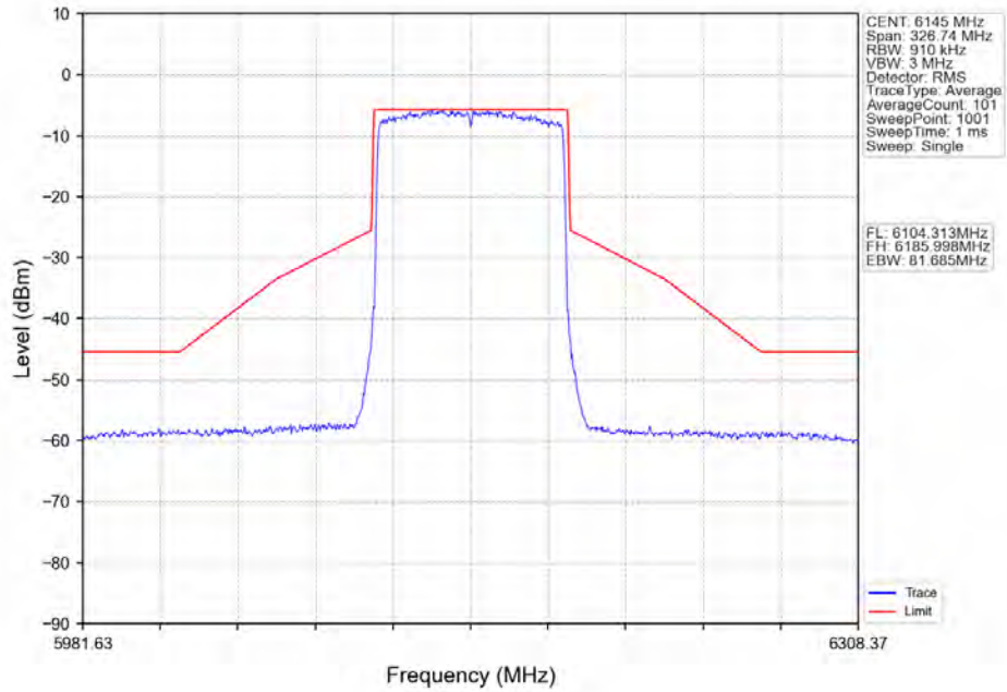
802.11ax(HE80)_MCH_6145MHz_RU996_Left_Ant2_NTNV
