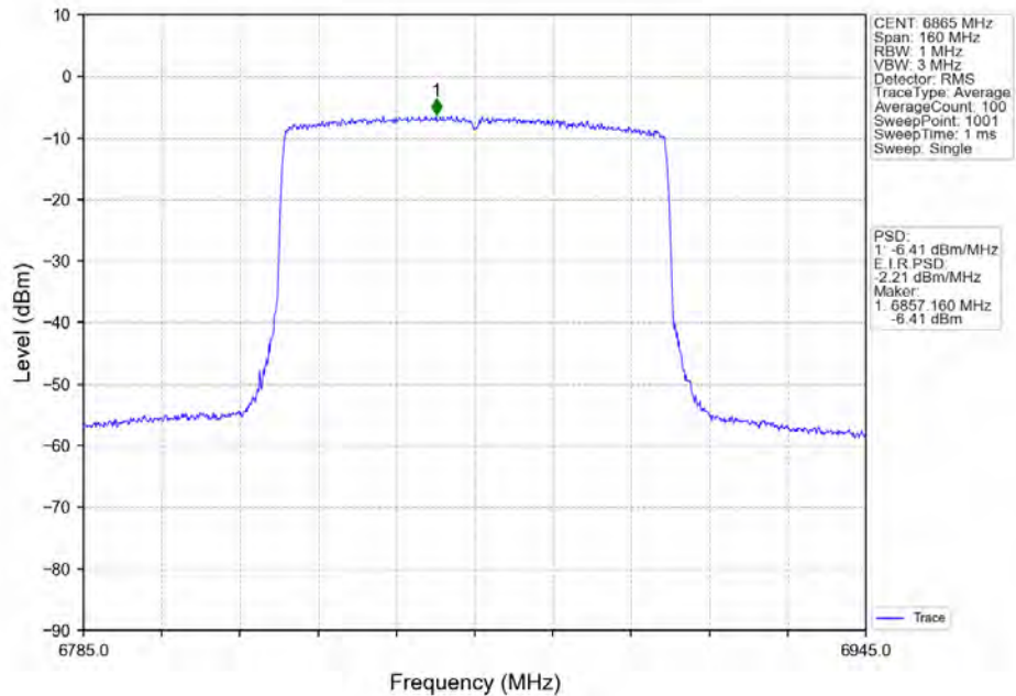
802.11ax(HE80)_HCH_6865MHz_RU996_Left_Ant2_NTNV
