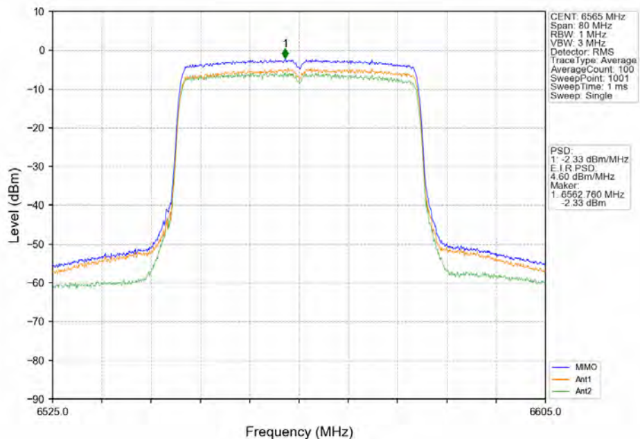
802.11ax(HE40)_LCH_6565MHz_RU484_Left_MIMO_NTNV
