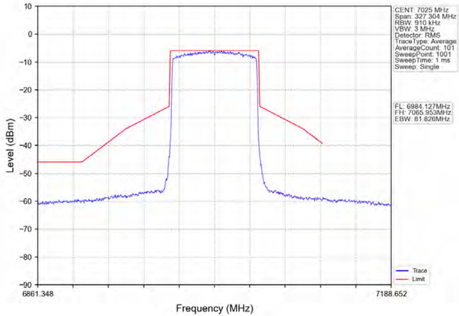
802.11ax(HE80)_HCH_7025MHz_RU996_Left_Ant2_NTNV
