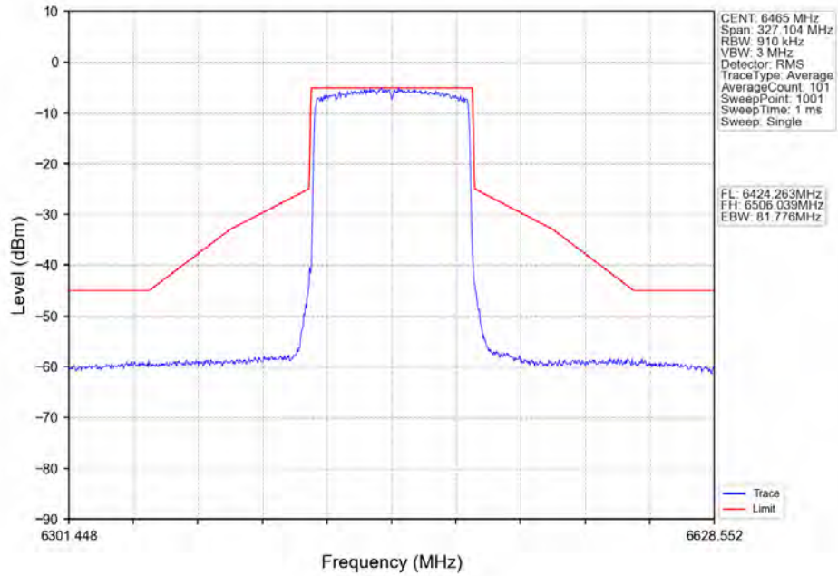
802.11ax(HE80)_LCH_6465MHz_RU996_Left_Ant2_NTNV
