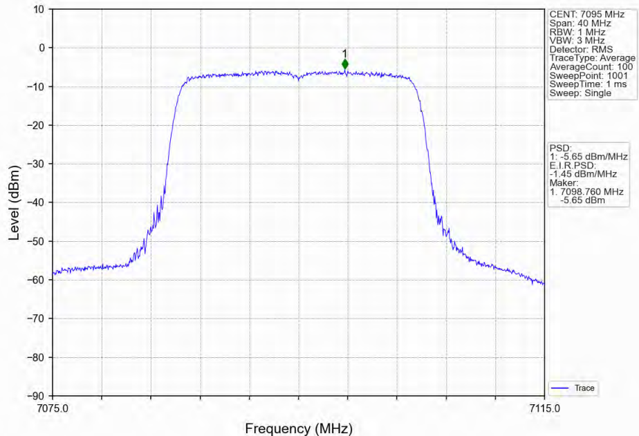
802.11ax(HE20)_HCH_7095MHz_RU242_Left_Ant2_NTNV
