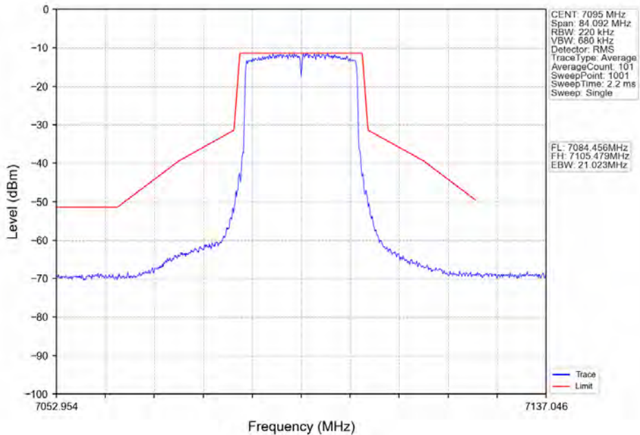
802.11ax(HE20)_HCH_7095MHz_RU242_Left_Ant2_NTNV
