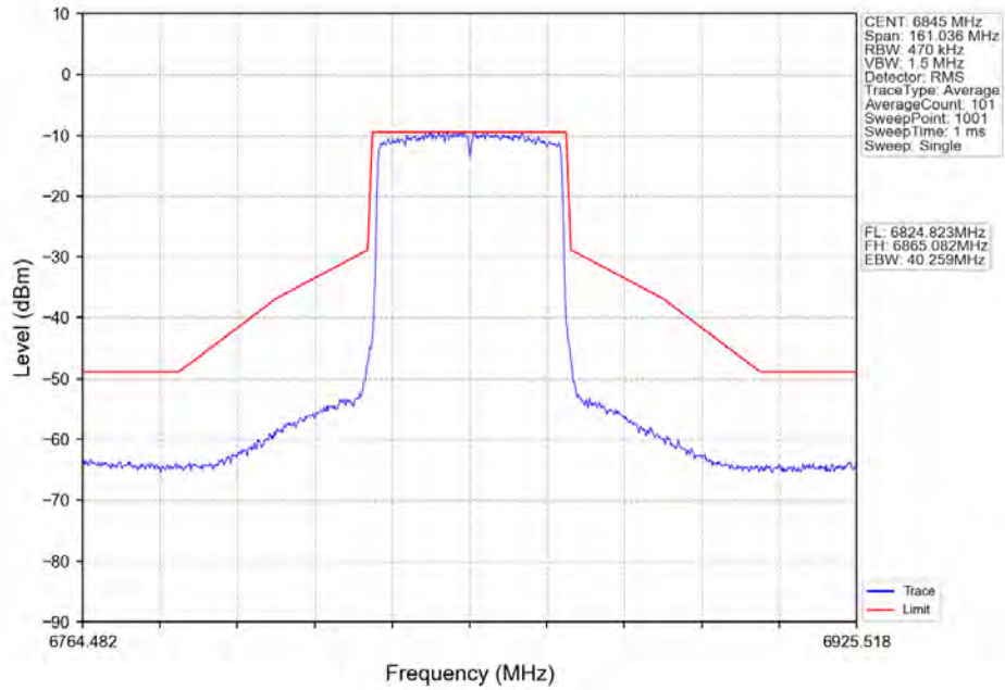
802.11ax(HE40)_HCH_6845MHz_RU484_Left_Ant2_NTNV
