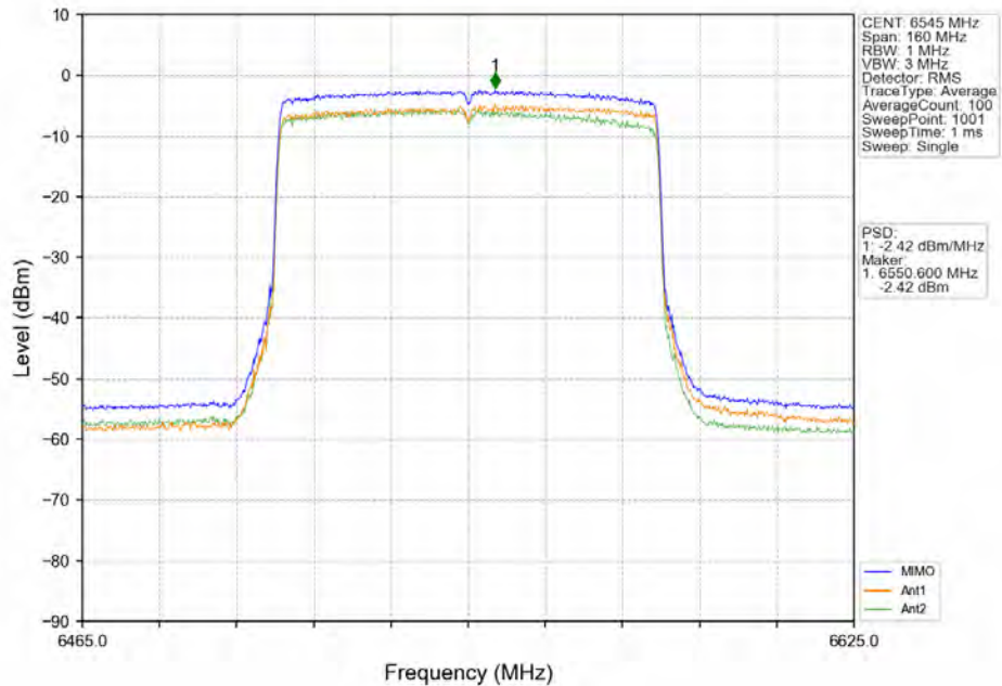
802.11ax(HE80)_HCH_6545MHz_RU996_Left_MIMO_NTNV
