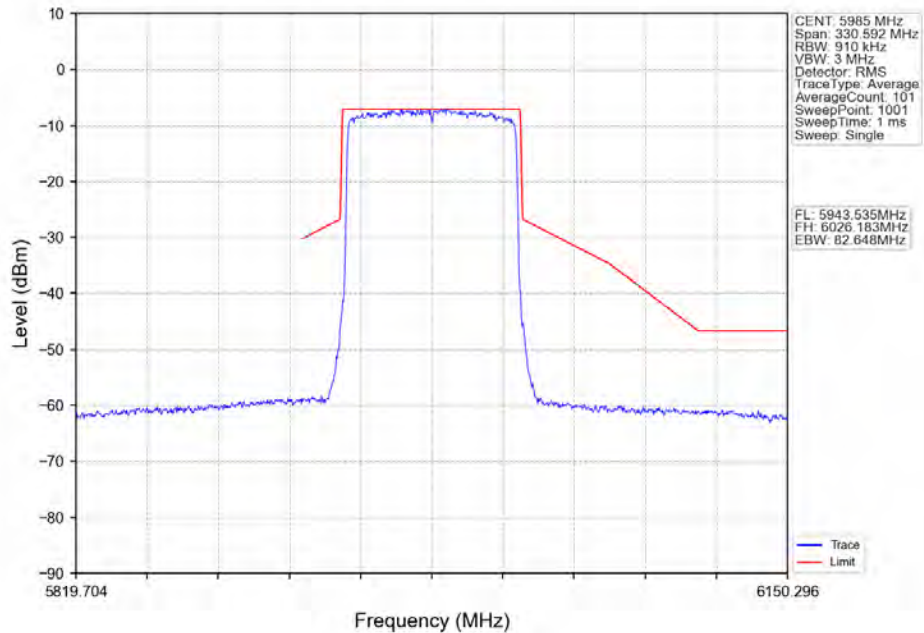
802.11ax(HE80)_LCH_5985MHz_RU996_Left_Ant2_NTNV
