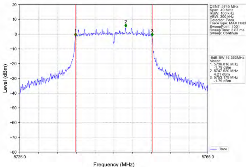
802.11a LCH 5745MHz Ant2 NTV
