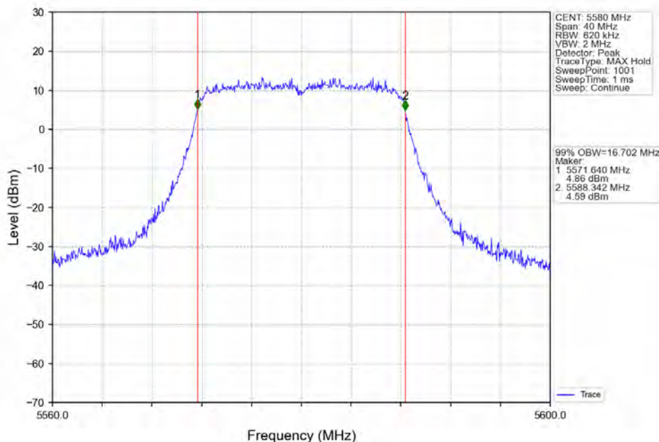
802.11a MCH 5580MHz Ant2 NTNV
