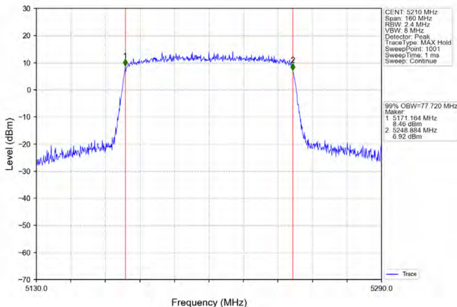
802.11ax(HE80) MCH 5210MHz RU996 Left Ant2 NTNv
