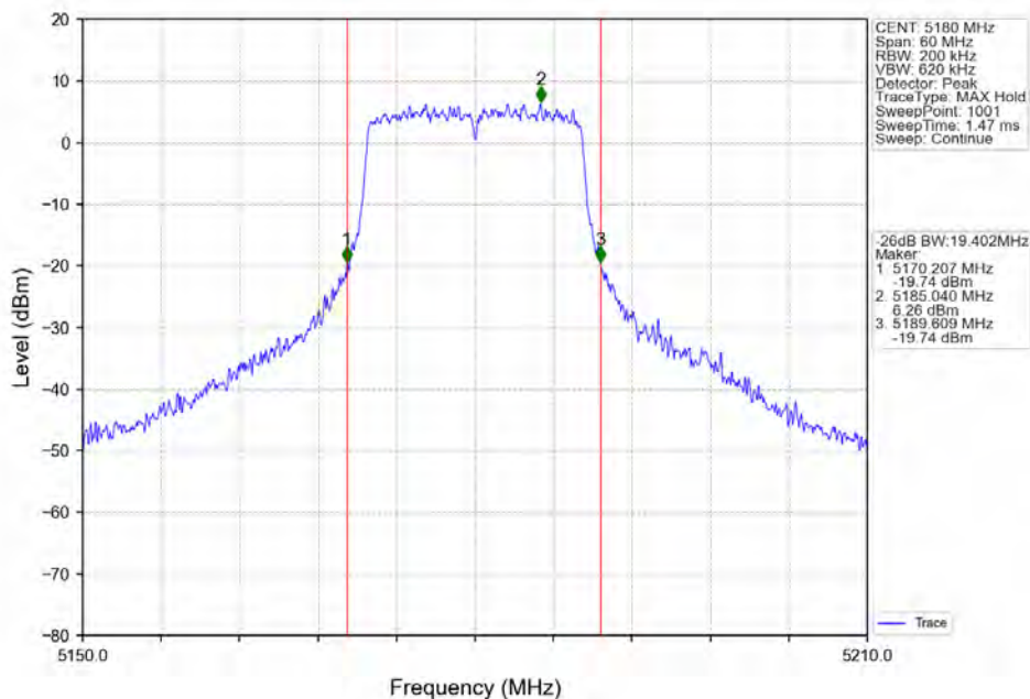
802.11a LCH 5180MHz Ant2 NTV
