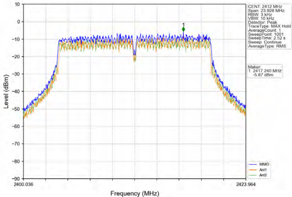
802.11g LCH 2412MHz MIMO NTNV
