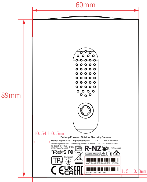
尺寸图
