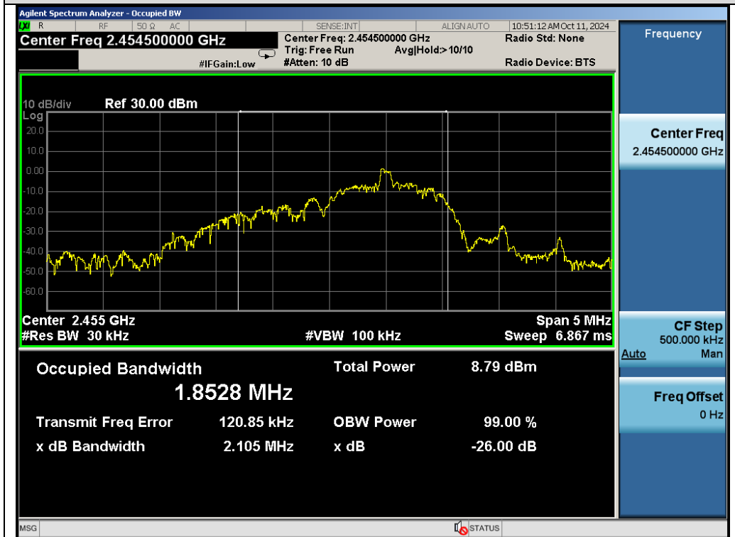
Test_Graph_GFSK_ANT1_2454.5_OBW
