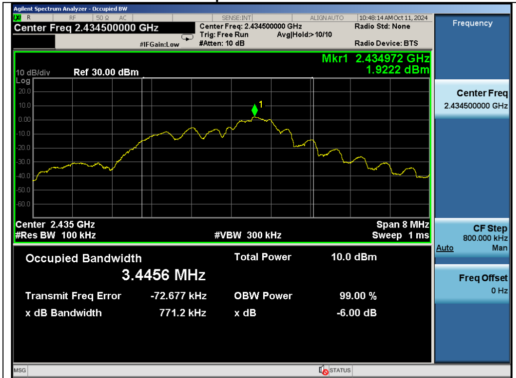
Test_Graph_GFSK_ANT1_2434.5_DTBSW
