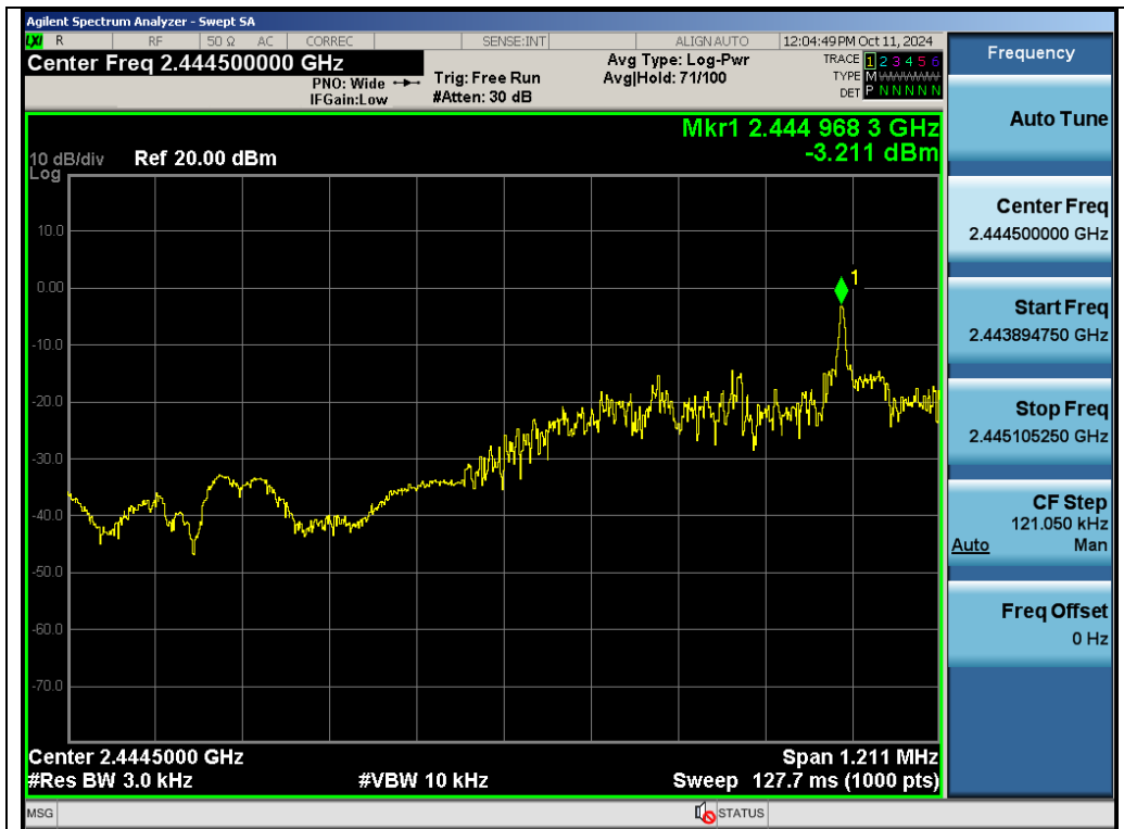
Test_Graph_GFSK_ANT1_2444.5_PSD
