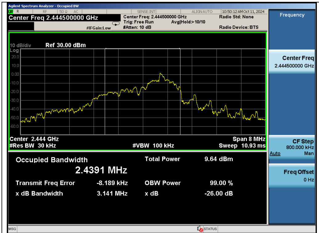
Test_Graph_GFSK_ANT1_2444.5_OBW
