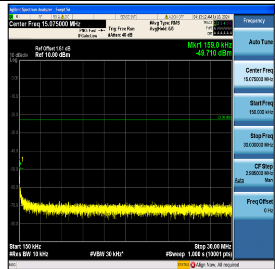
150KHz-30MHz
