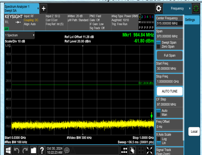
11G-Ant1-2412-30~1000-PASS
