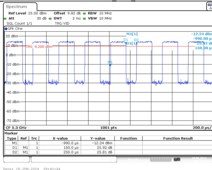
11AC20MIMO_Ant2_5300
