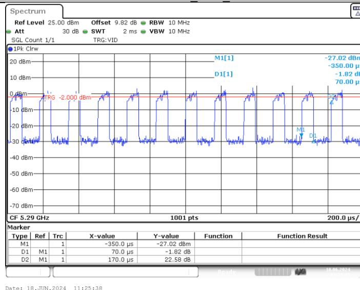
11AC80MIMO_Ant2_5290
