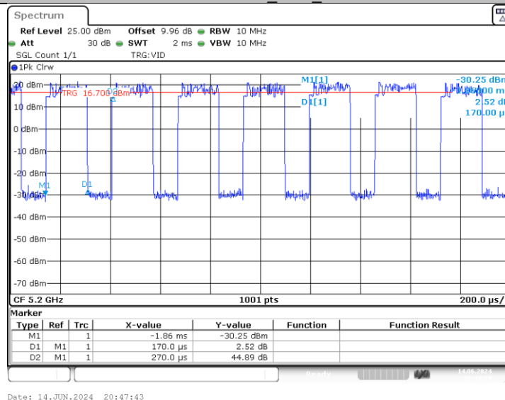
11AC20MIMO_Ant2_5200
