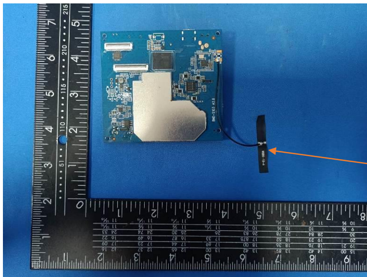
PIFA antenna
