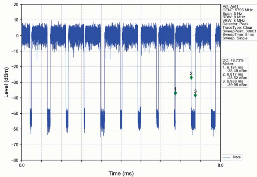
802.11n(HT40) HCH_5795MHz_Ant1_NTNV
