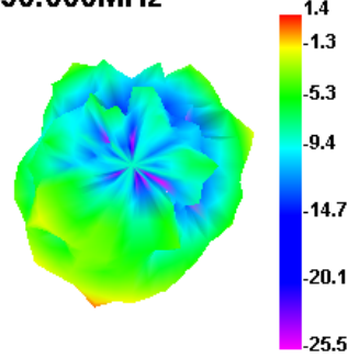
5450.000MHz
