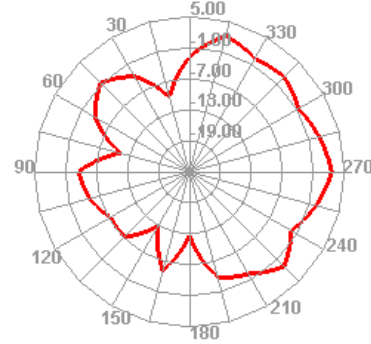
5850.000MHz H
