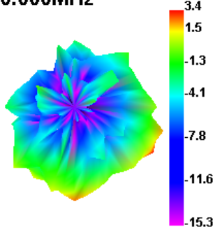
5850.000MHz
