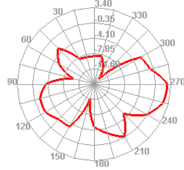
5850.000MHz E2
