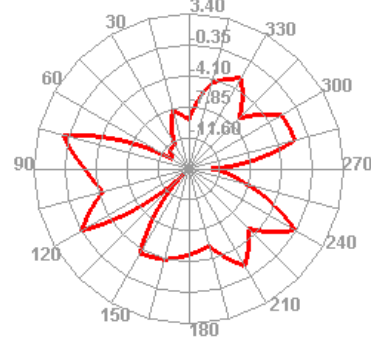
5850.000MHz E1
