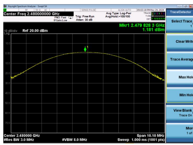
GFSK(CH78)
