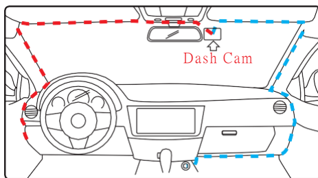
— — — — — Hardwire Kit Wiring (2.3.1) — — — — — Car Charging Cable Wiring (2.3.2)
