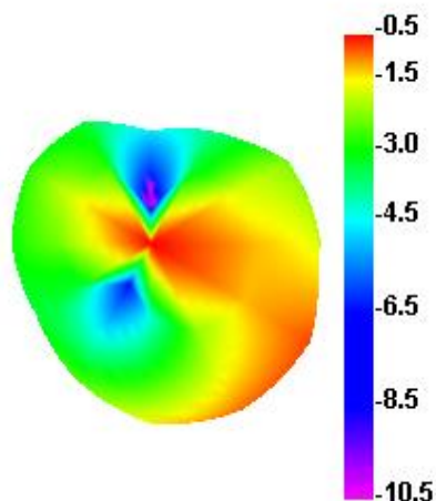
2450.000MHz E1
