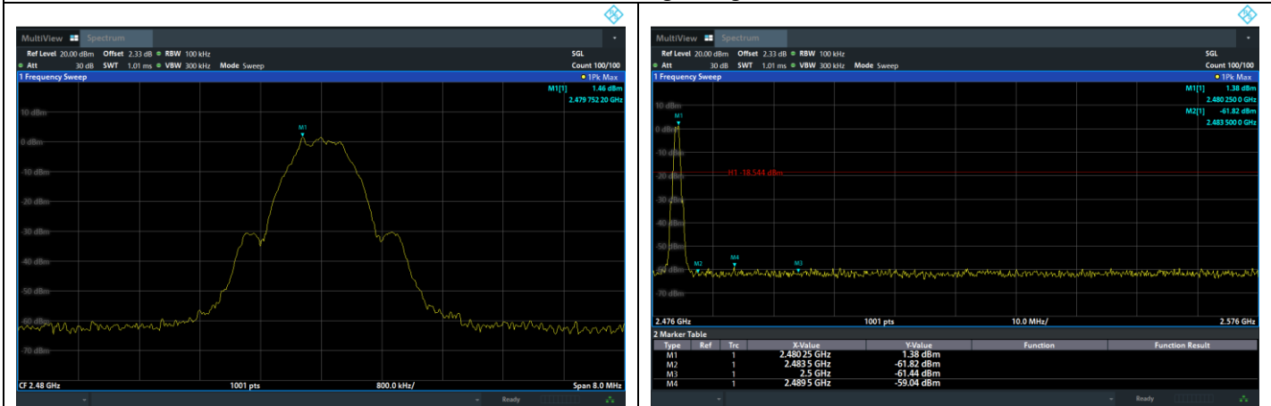
BLE 1M: Band Edge, Right Side
