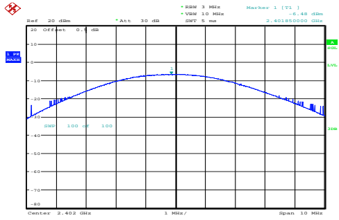
Low -6.48dBm
