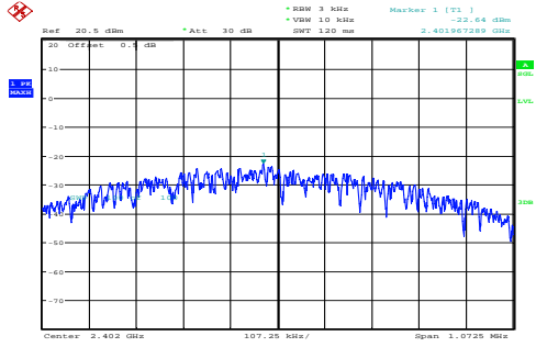
Low -22.64dBm/3kHz
