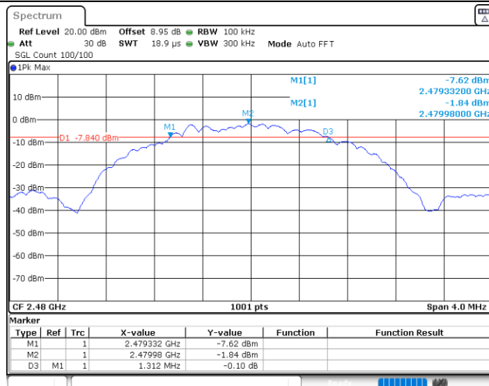
BLE_2M_Ant1_2480
