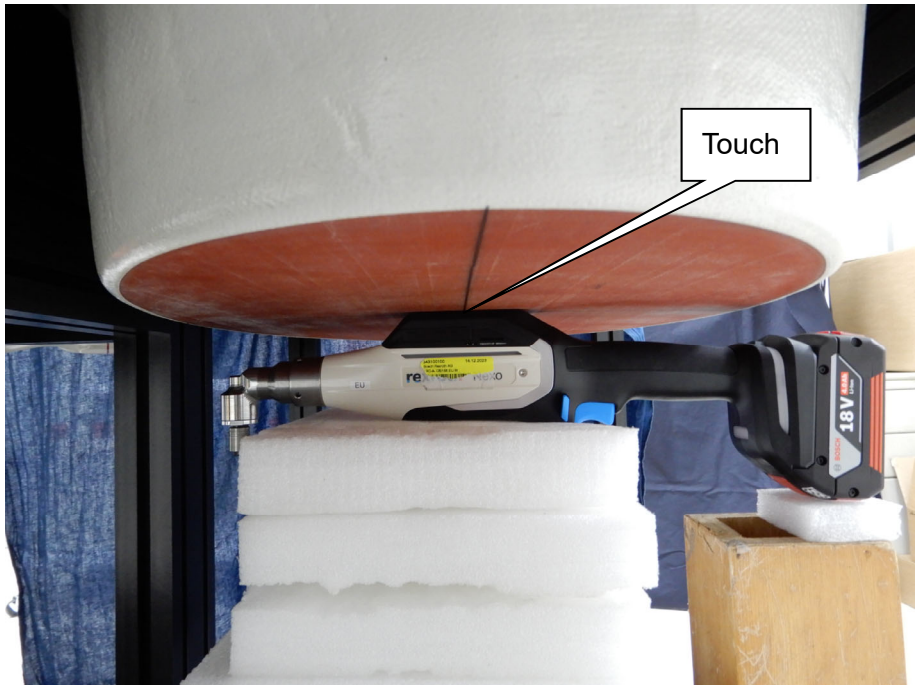
EUT Top_NX_-A
