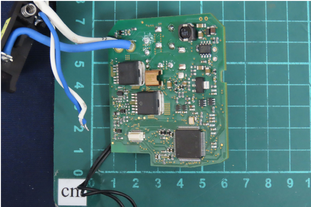
(62) EUT Photo
