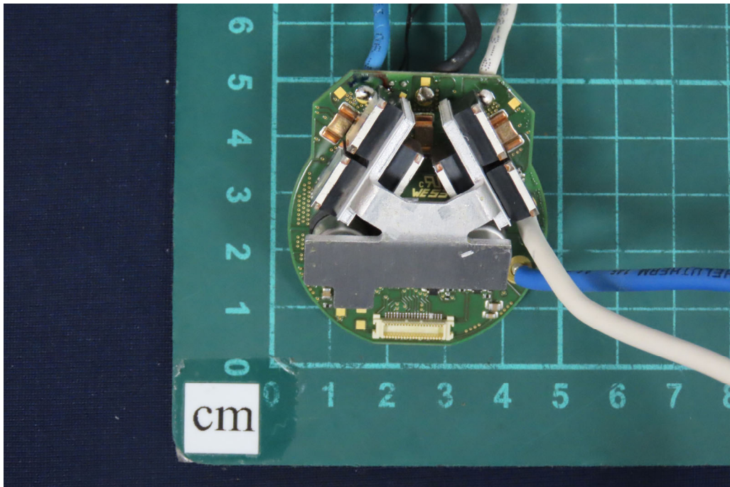
(64) EUT Photo
