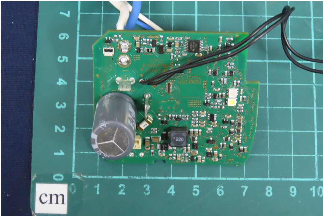
(61) EUT Photo
