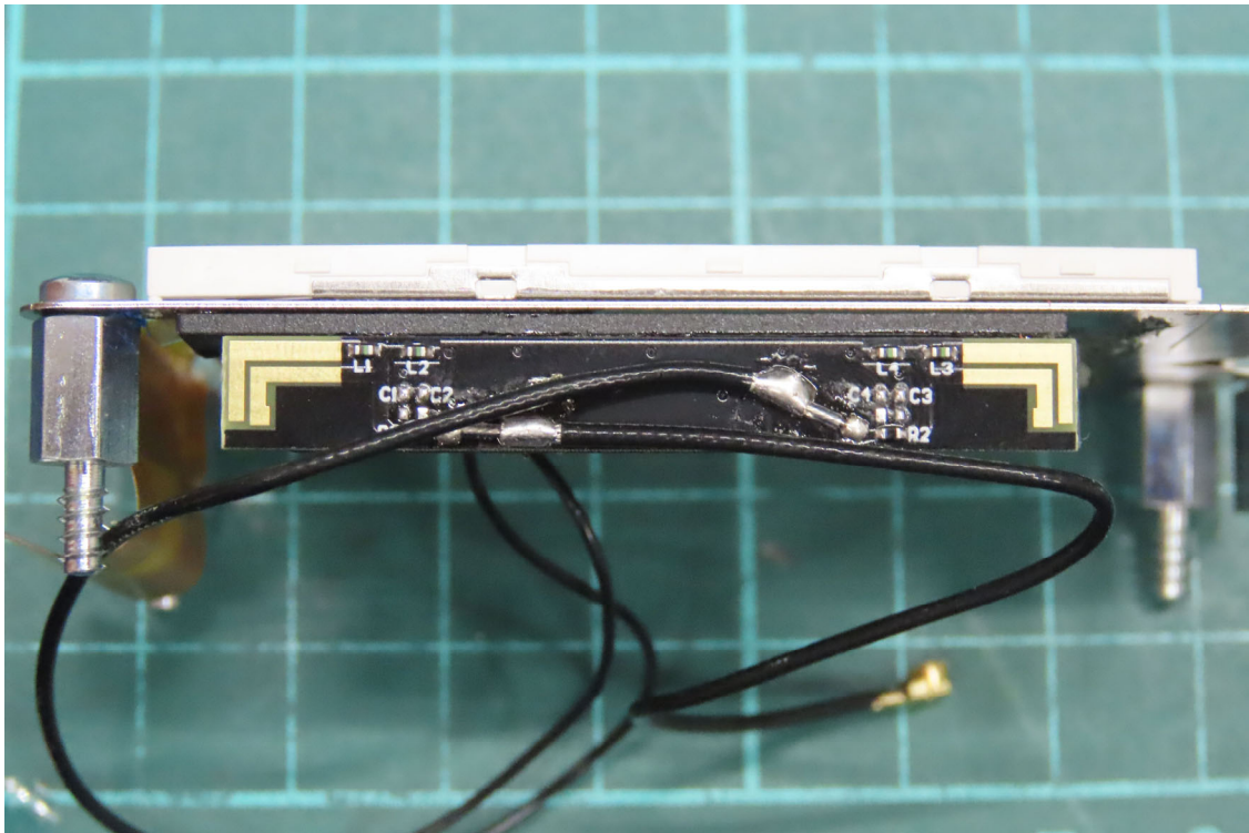
(52) EUT Photo
