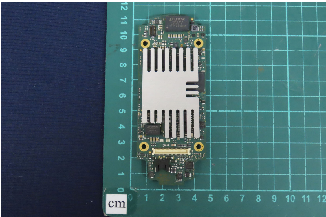
(54) EUT Photo
