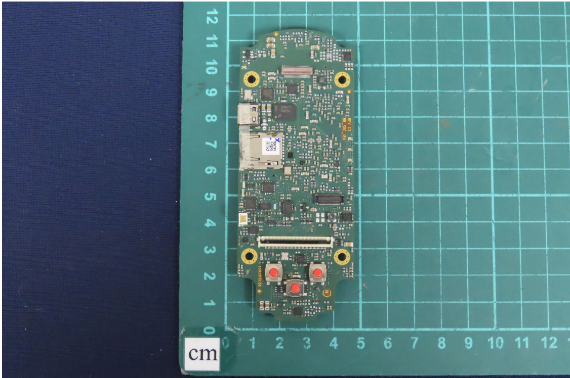
(53) EUT Photo
