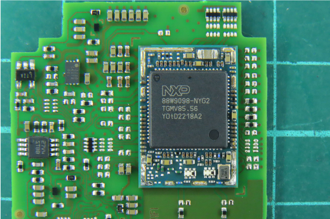
(49) EUT Photo
