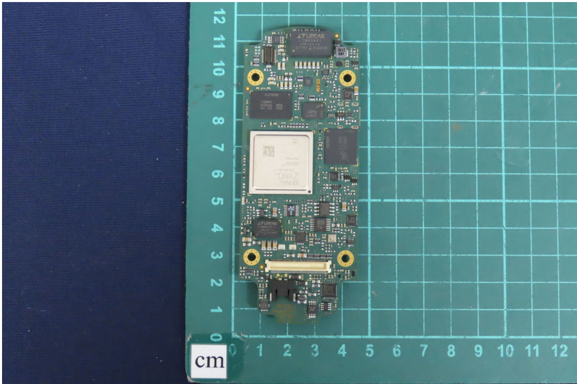
(56) EUT Photo
