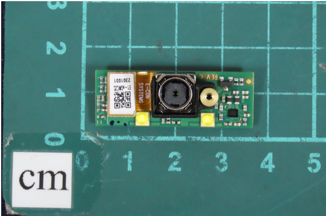
(44) EUT Photo
