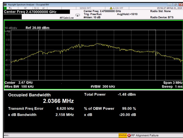
2470MHz
