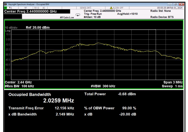
2440MHz
