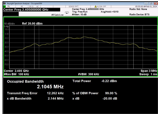
2405MHz
