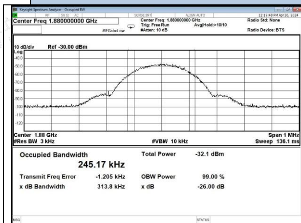
GSM-PCS band UL input
