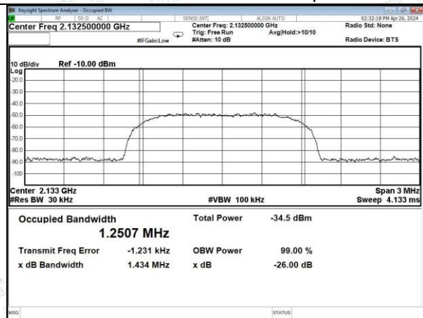
CDMA-AWS band DL input
