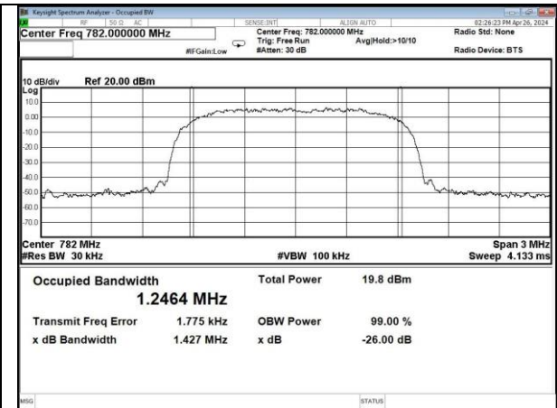
CDMA-Upper 700 band UL output
