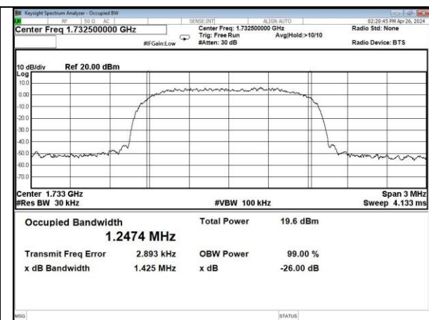
CDMA-AWS band UL output
