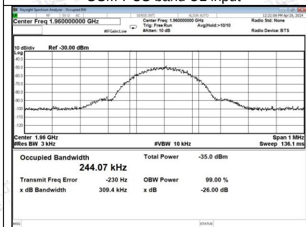
GSM-PCS band DL input
