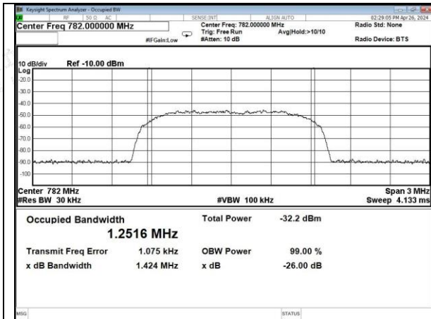
CDMA-Upper 700 band UL input
