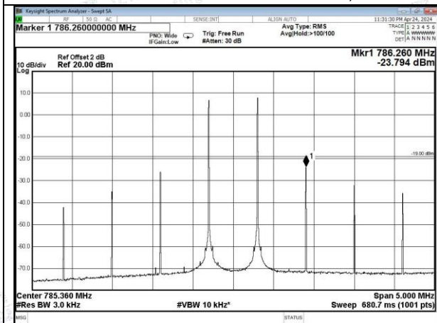
Upper 700MHz band Pre AGC, UL
