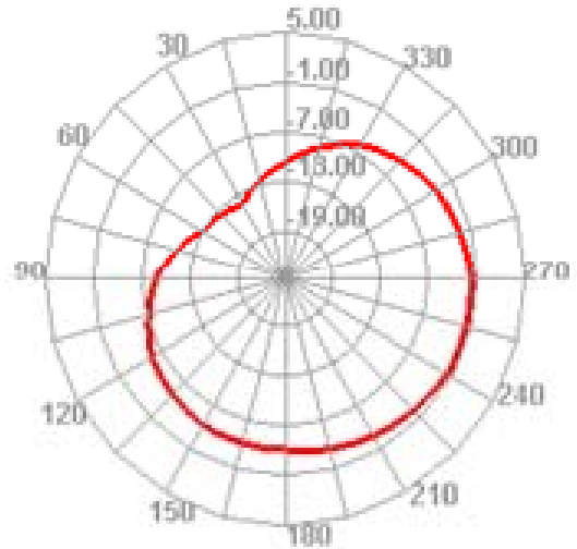
915.000MHz H
