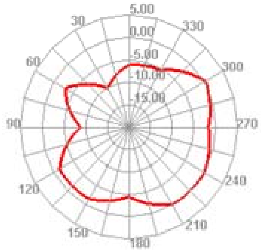
915.000MHz E2
