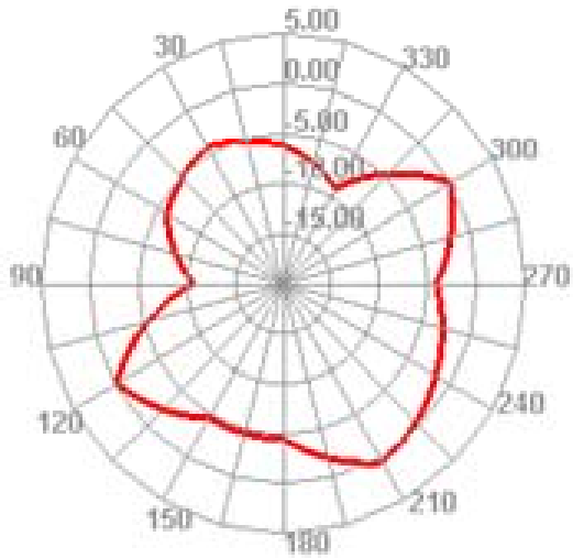
915.000MHz E1
