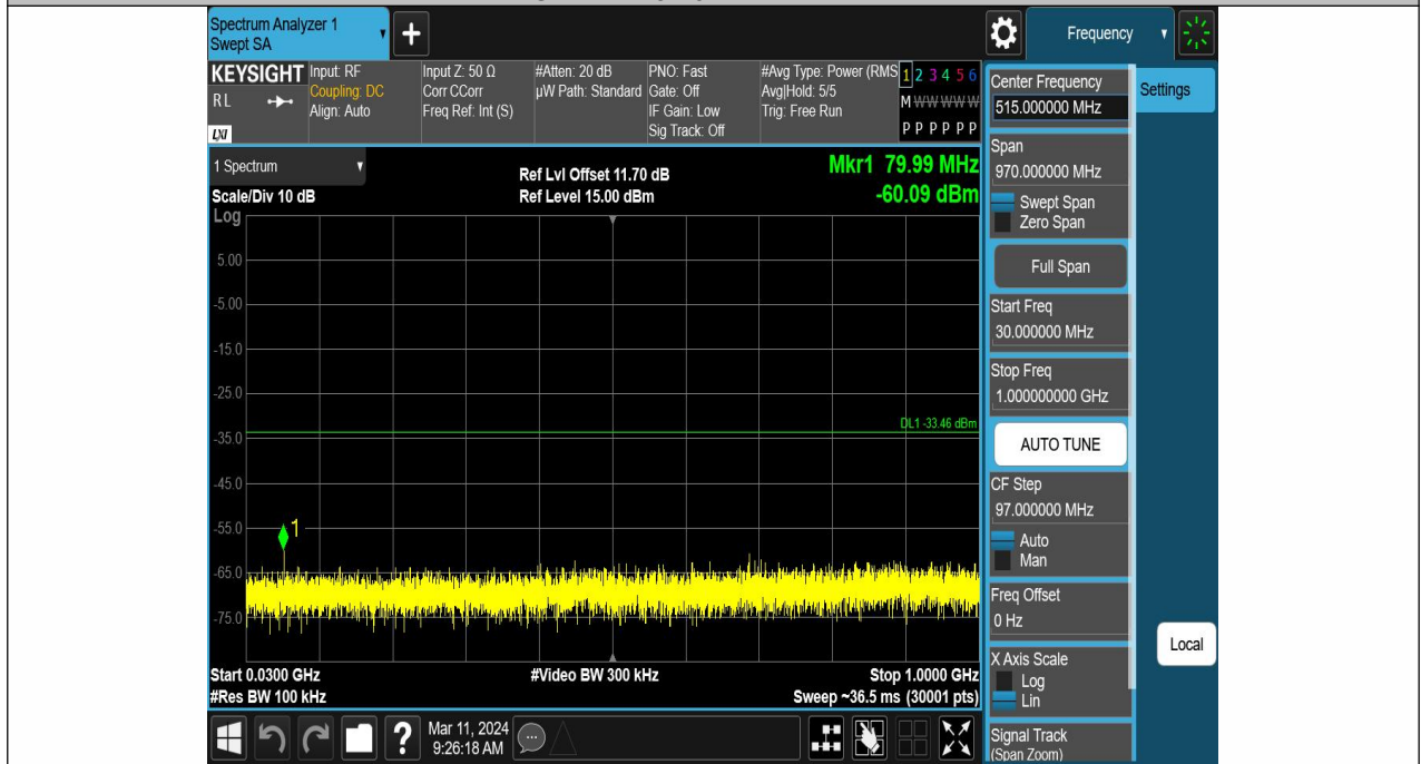
11G-Ant1-2437-30~1000-PASS
