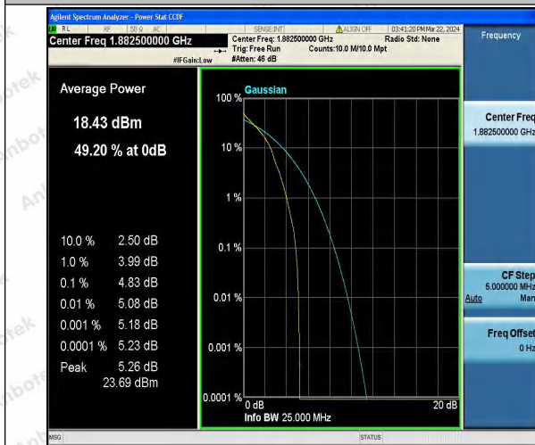
Band25-20MHz-QPSK-26365-1RB#0-PASS
