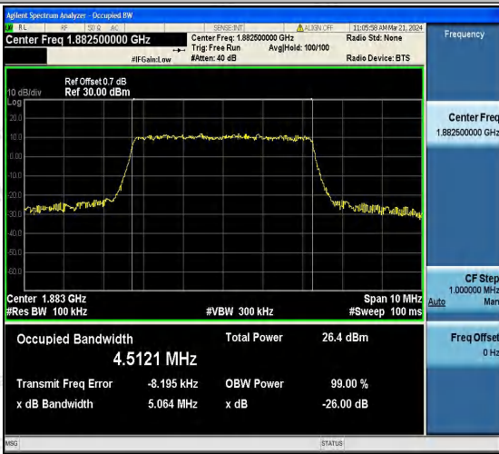
Band25-5MHz-QPSK-26365-25RB#0-PASS
