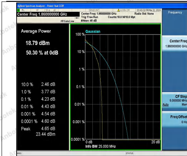
Band25-20MHz-QPSK-26140-1RB#0-PASS
