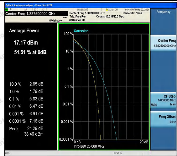
Band25-20MHz-QPSK-26365-100RB#0-PASS
