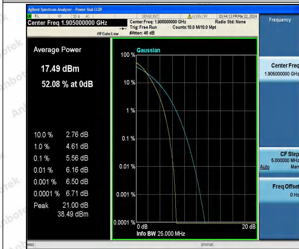
Band25-20MHz-QPSK-26590-100RB#0-PASS
