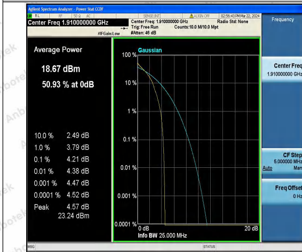
Band25-10MHz-QPSK-26640-1RB#0-PASS
