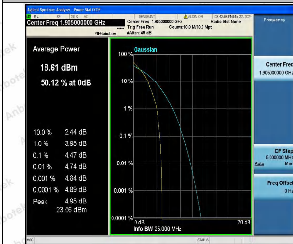
Band25-20MHz-QPSK-26590-1RB#0-PASS
