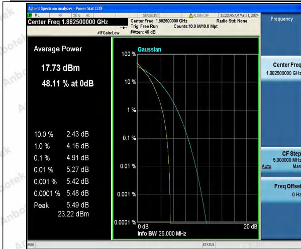
Band25-5MHz-QPSK-26365-25RB#0-PASS
