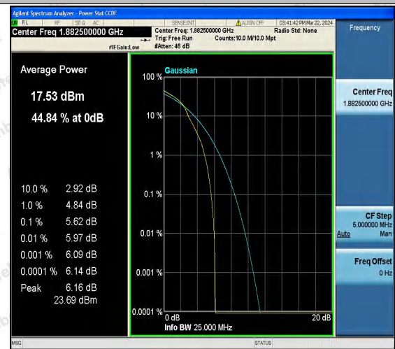
Band25-20MHz-16QAM-26365-1RB#0-PASS
