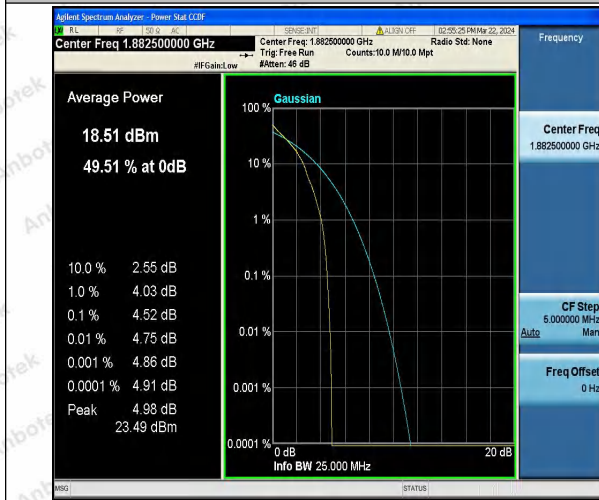
Band25-10MHz-QPSK-26365-1RB#0-PASS
