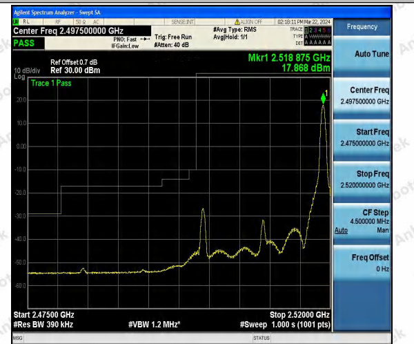
Band7_20MHz_16QAM_20850_1RB#99
