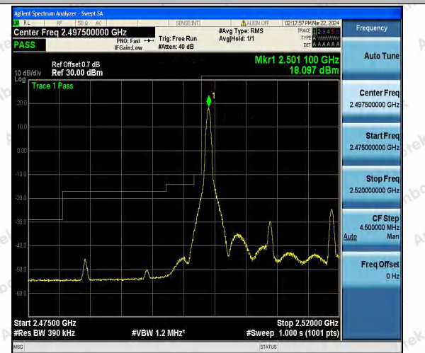
Band7_20MHz_16QAM_20850_1RB#0
