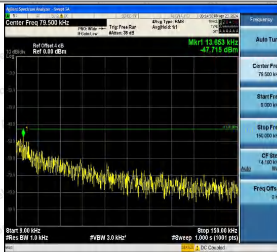
Band4-1513-5-0.009~0.15MHz-PASS
