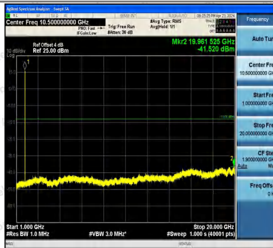
Band4-1513-5-1000~20000MHz-PASS
