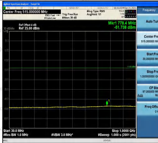
Band4-1413-4-30~1000MHz-PASS
