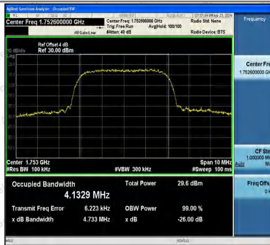
Band4-1513-5-PASS
