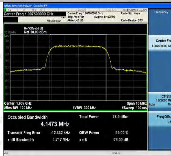
Band2-9538-3-PASS
