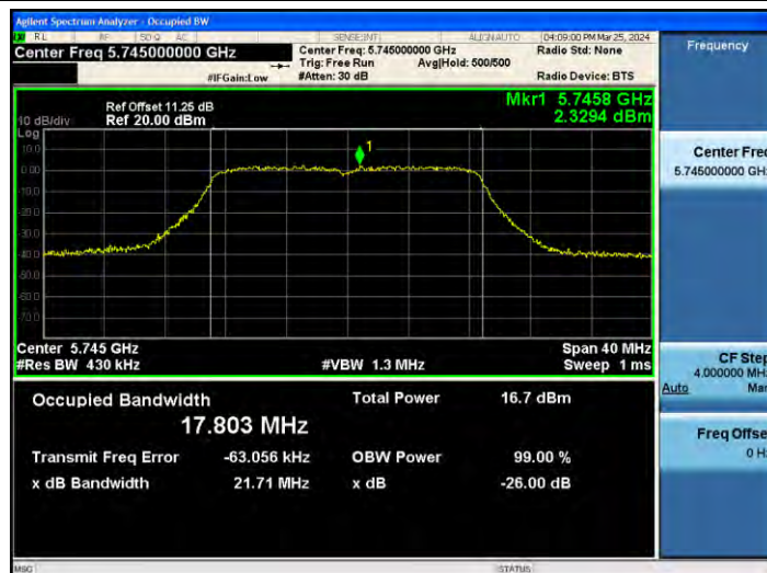
11AC20MIMO_Ant1_5745
