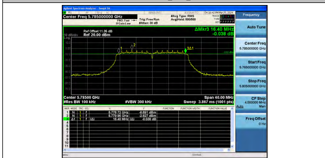
11AC20MIMO_Ant2_5785
