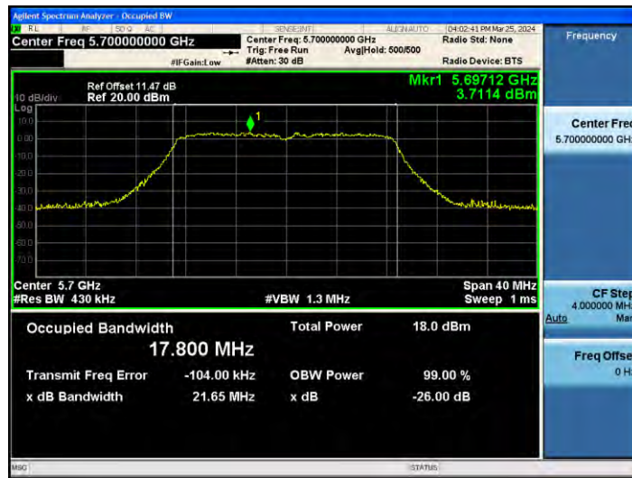
11AC20MIMO_Ant2_5700
