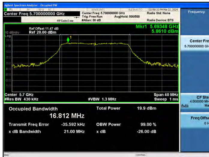
11A_Ant2_5700
