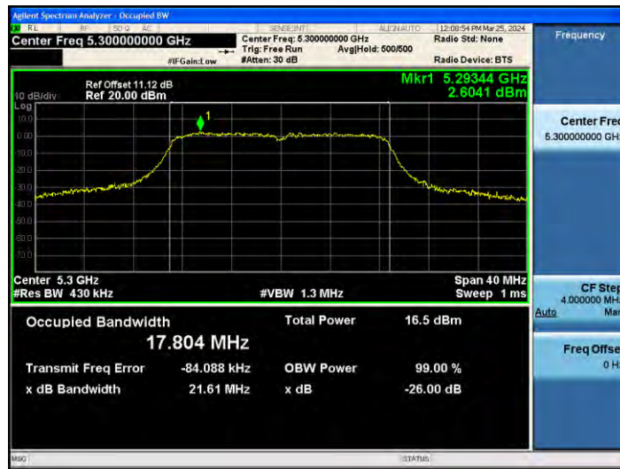
11N20MIMO_Ant2_5300
