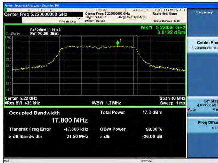
11N20MIMO_Ant2_5220
