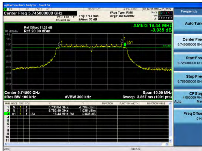
11N20MIMO_Ant2_5745
