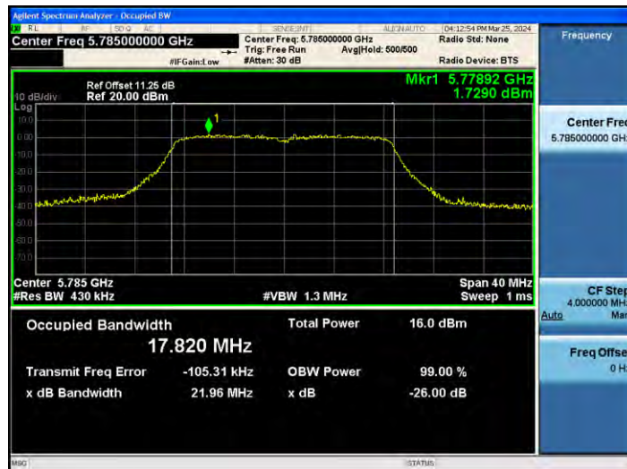
11AC20MIMO_Ant2_5785
