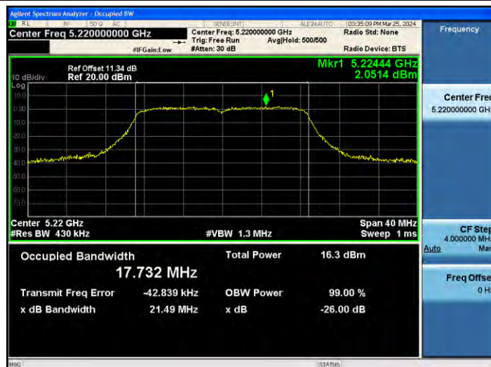
11AC20MIMO_Ant2_5220
