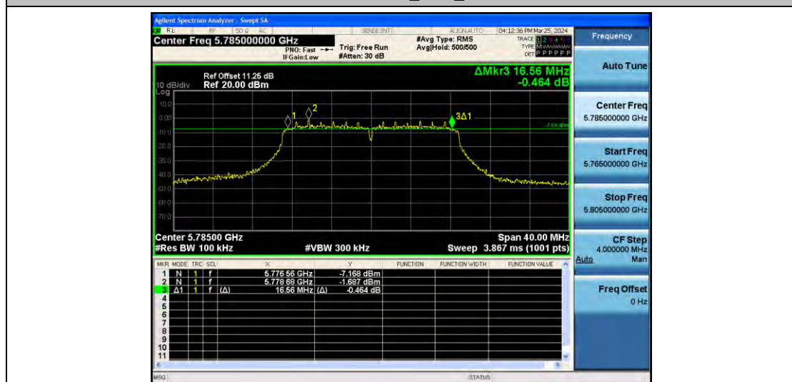
11AC20MIMO_Ant2_5785
