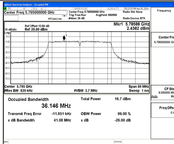
11AC40MIMO-Ant1-5795
