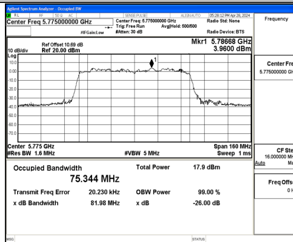
11AC80MIMO-Ant1-5775
