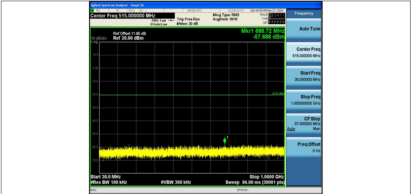
11G-Ant1-2412-30~1000-PASS
