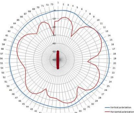
天线垂直辐射图
