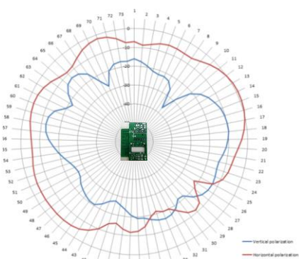
天线水平辐射图
