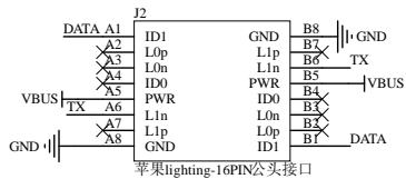
苹果lighting接口输入
