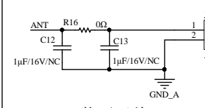
蓝牙天线
