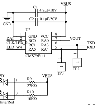
MCU电路
