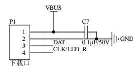
烧录下载接口
