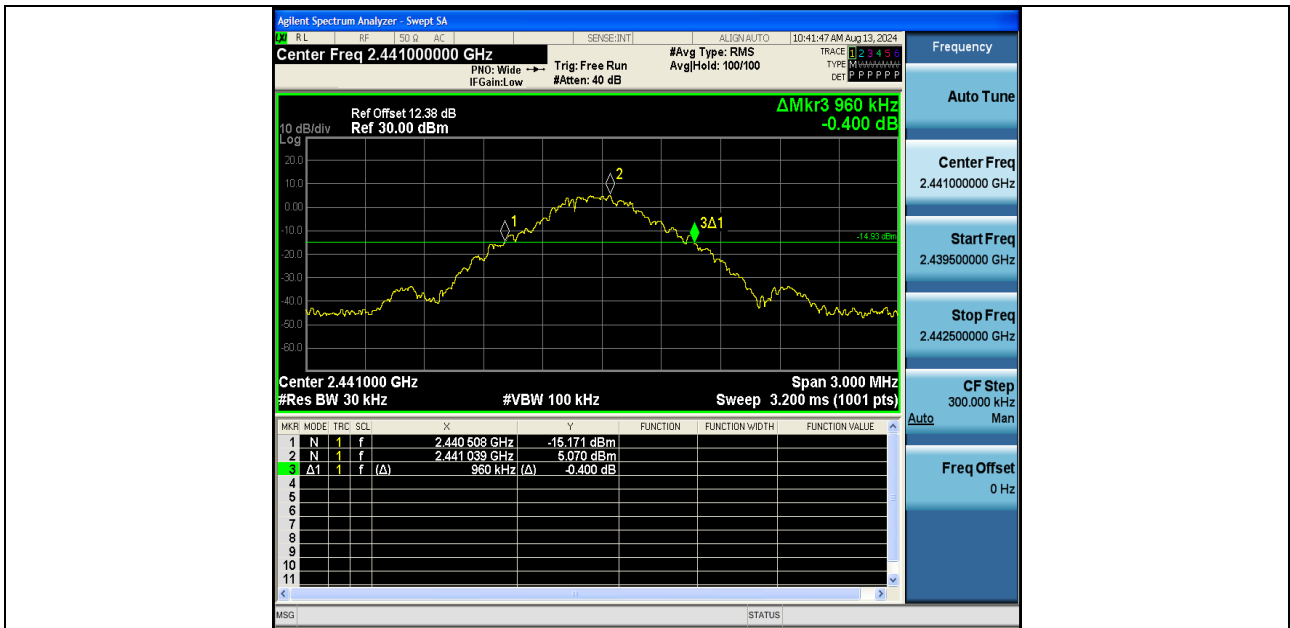
DH5-Ant1-2441
