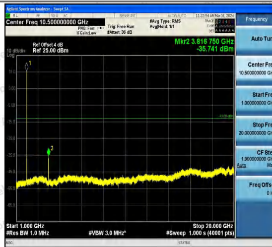
Band2-9538-1-1000~20000MHz-PASS
