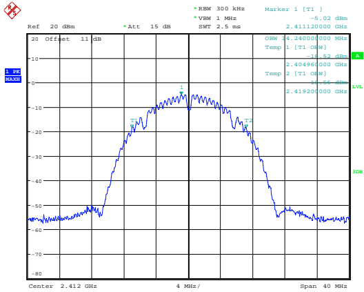
b_2412MHz_Chain 0
