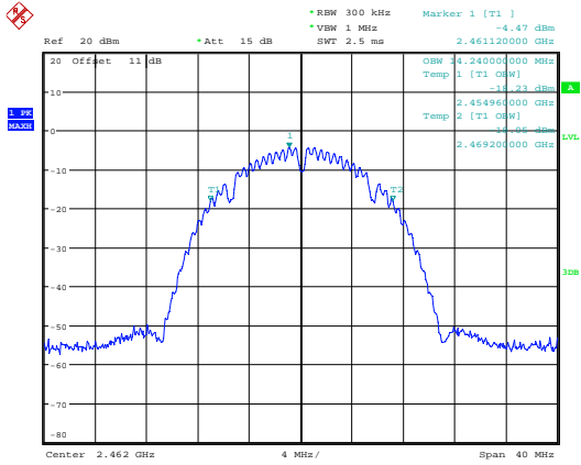
b_2462MHz_Chain 0
