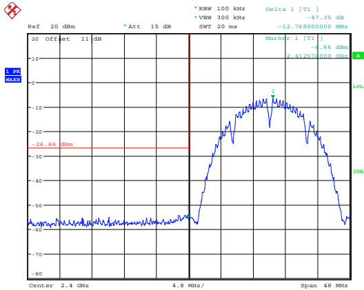
b_2412MHz_Chain 0
