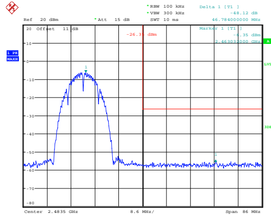
b_2462MHz_Chain 0
