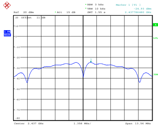
b_2437MHz_Chain 0
