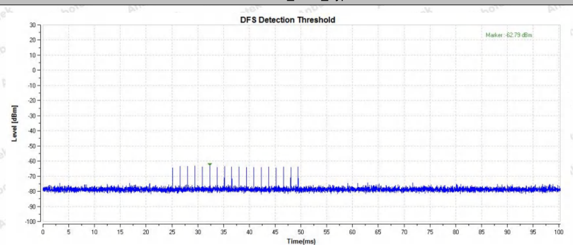
11AC80SISO_5290_Type0
