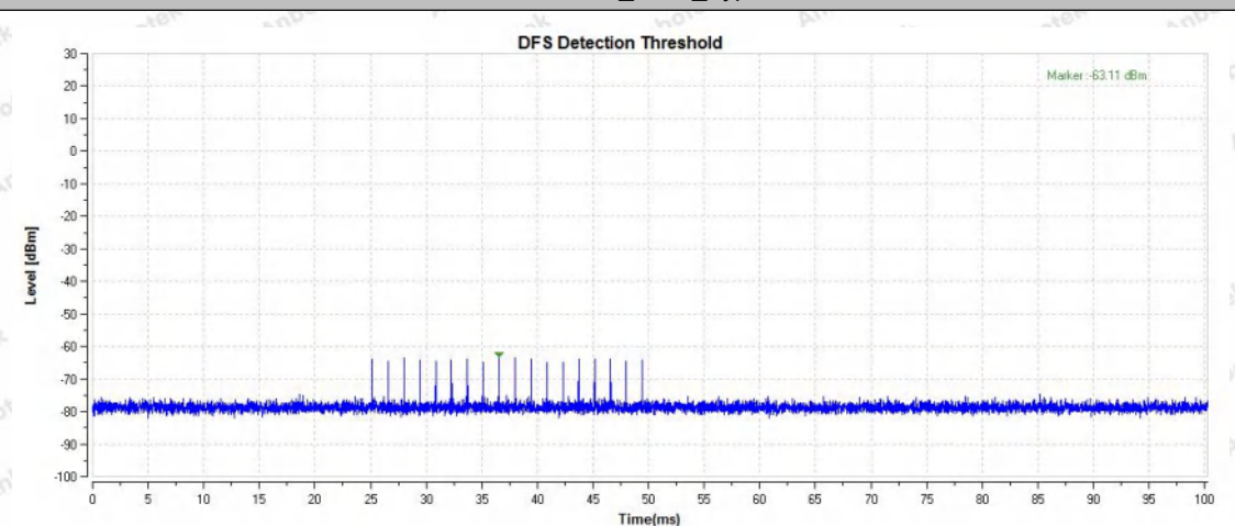
11AC80SISO_5610_Type0
