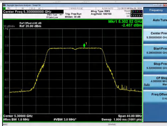
11A-Ant0-5300-PASS
