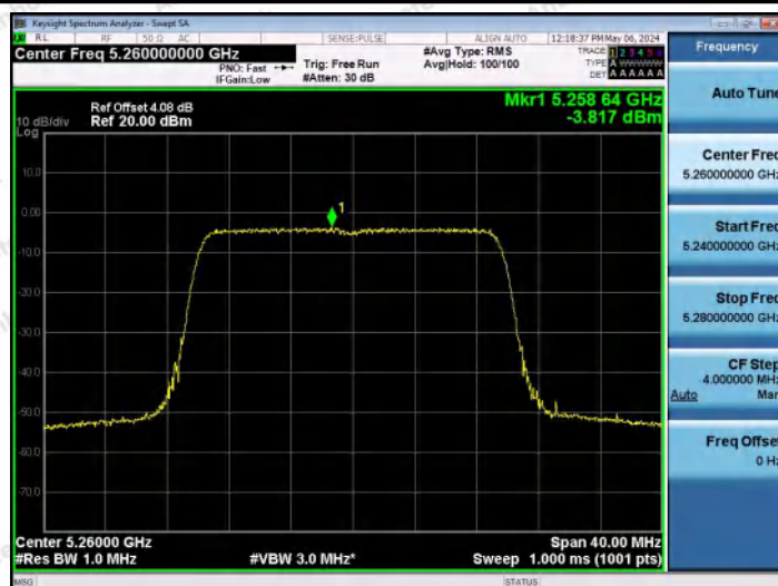
11AX20MIMO-Ant0-5260-PASS
