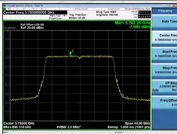
11AX20MIMO-Ant1-5785-PASS
