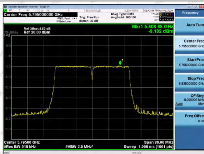
11N40MIMO-Ant1-5795-PASS
