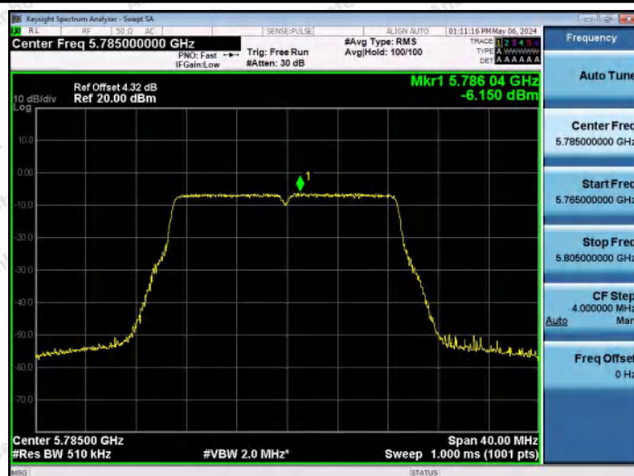
11N20MIMO-Ant0-5785-PASS
