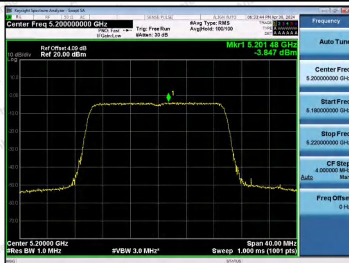
11AX20MIMO-Ant1-5200-PASS
