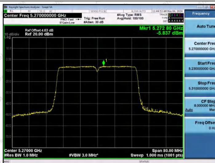
11N40MIMO-Ant0-5270-PASS
