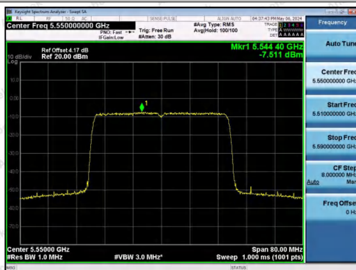
11AX40MIMO-Ant0-5550-PASS
