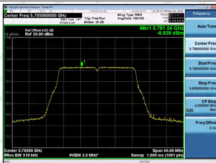
11AC20MIMO-Ant0-5785-PASS
