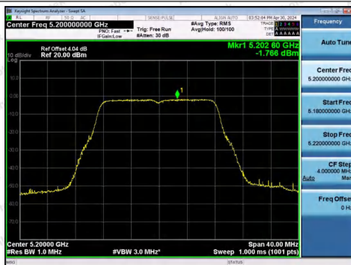
11A-Ant0-5200-PASS
