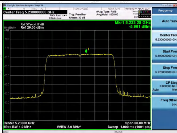
11AX40MIMO-Ant1-5230-PASS
