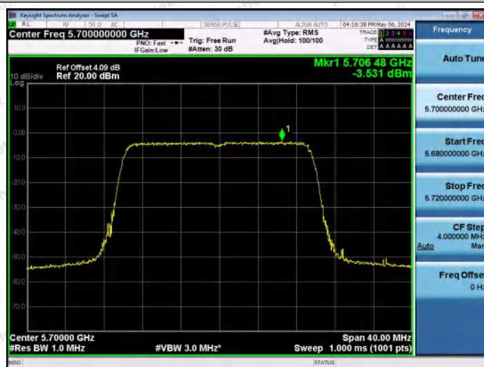
11AX20MIMO-Ant1-5700-PASS
