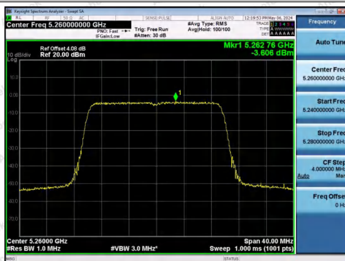
11AX20MIMO-Ant1-5260-PASS
