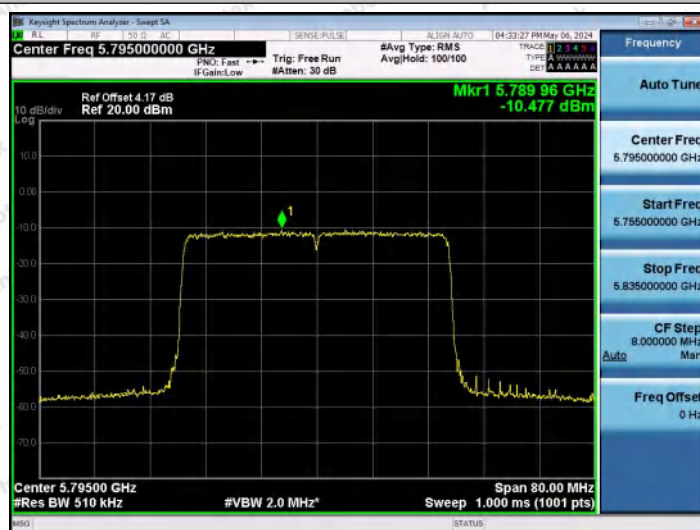
11AX40MIMO-Ant1-5795-PASS
