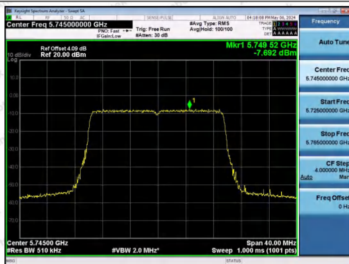
11AX20MIMO-Ant0-5745-PASS
