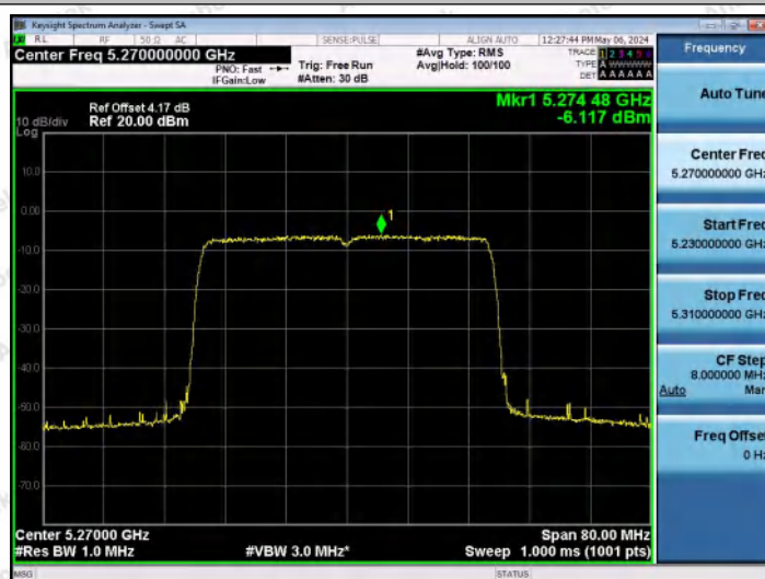
11AX40MIMO-Ant0-5270-PASS
