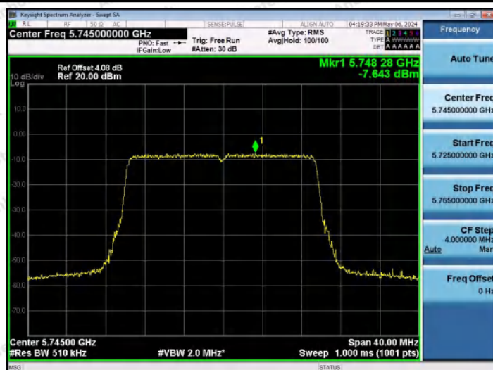
11AX20MIMO-Ant1-5745-PASS
