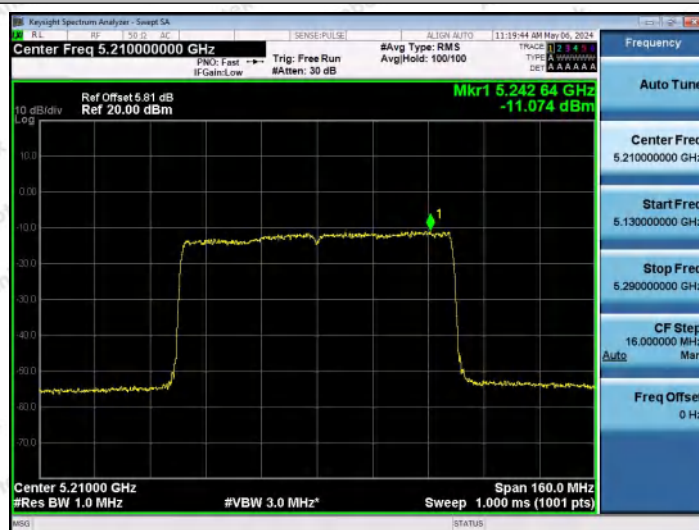
11AX80MIMO-Ant0-5210-PASS
