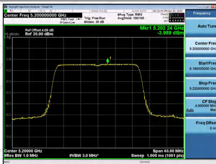
11AX20MIMO-Ant0-5200-PASS
