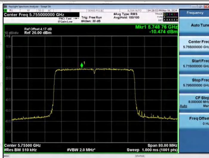
11AX40MIMO-Ant0-5755-PASS
