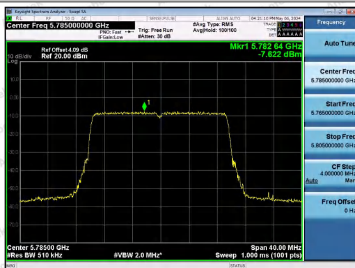
11AX20MIMO-Ant0-5785-PASS
