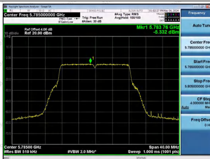
11A-Ant0-5785-PASS
