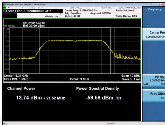
11N20MIMO-Ant0-5260-PASS
