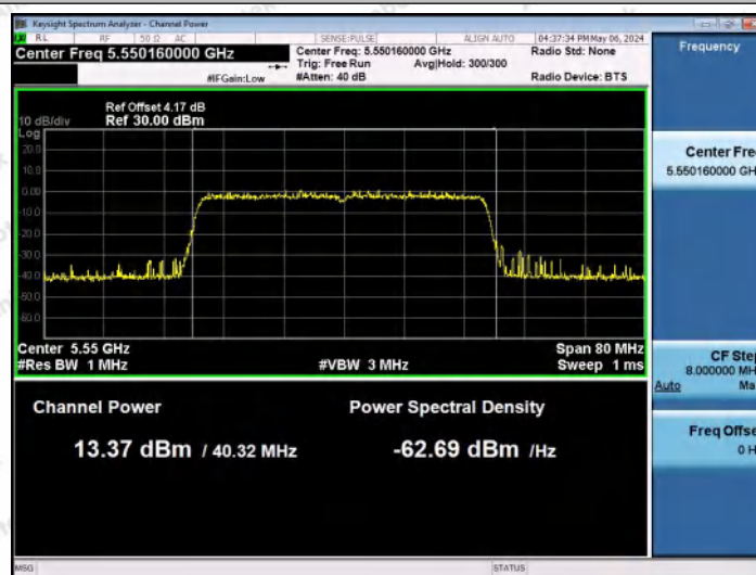
11AX40MIMO-Ant0-5550-PASS
