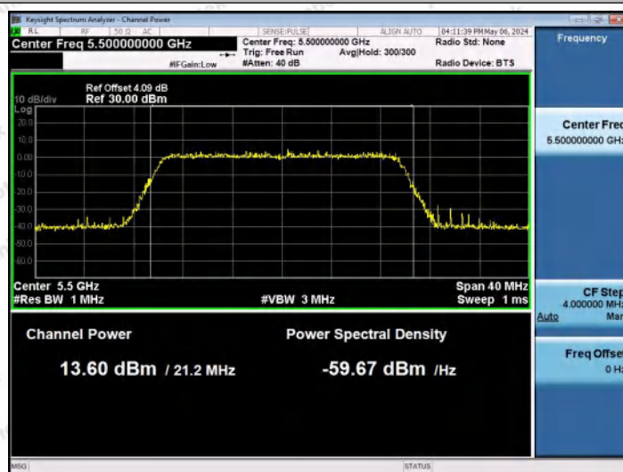
11AX20MIMO-Ant1-5500-PASS
