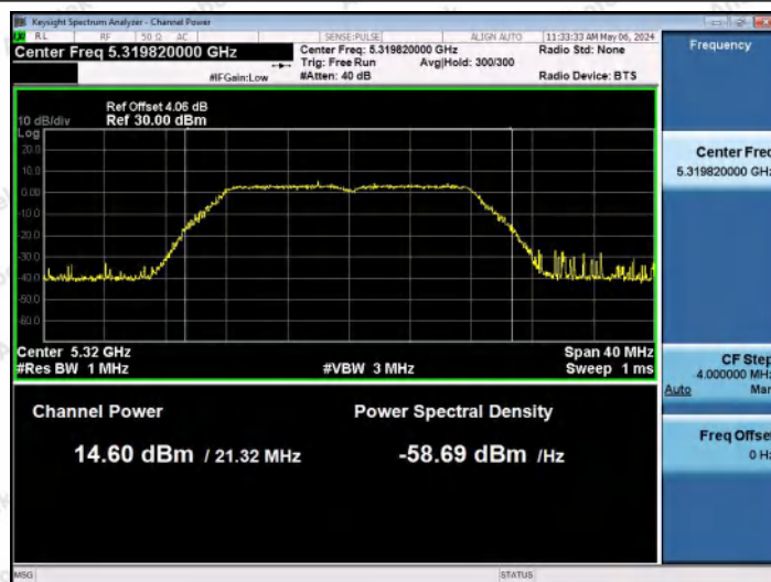
11A-Ant0-5320-PASS
