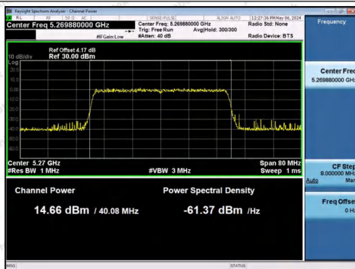
11AX40MIMO-Ant0-5270-PASS
