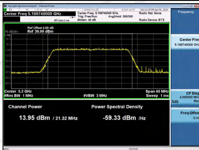
11AX20MIMO-Ant0-5200-PASS
