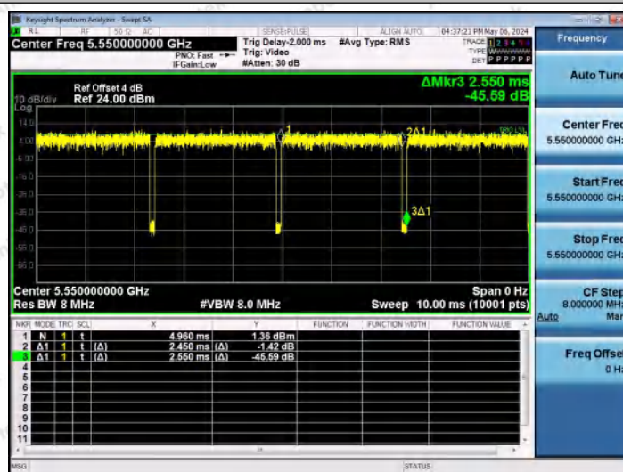
NTNV-11AX40MIMO-Ant0-5550
