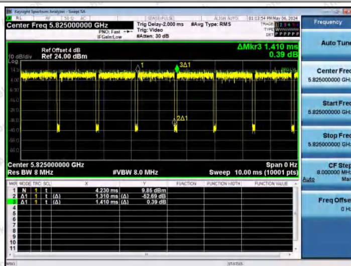
NTVN-11N20MIMO-Ant0-5825
