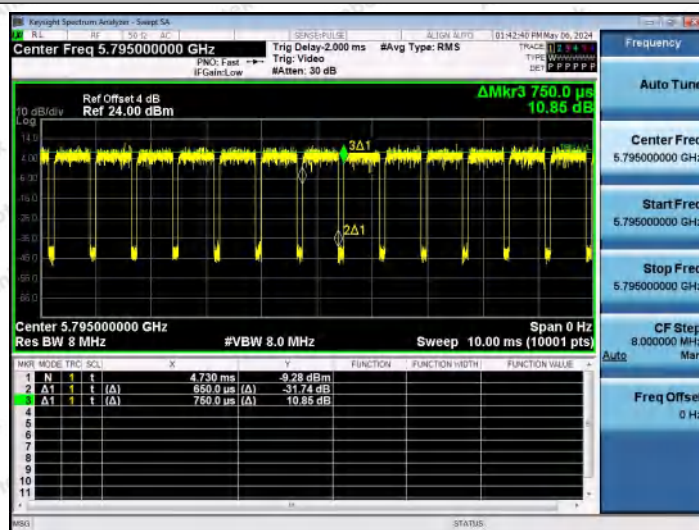
NTNV-11N40MIMO-Ant1-5795
