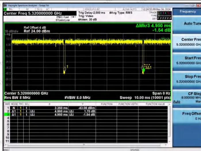
NTNV-11AX20MIMO-Ant1-5320
