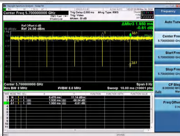
NTNV-11AC20MIMO-Ant0-5700
