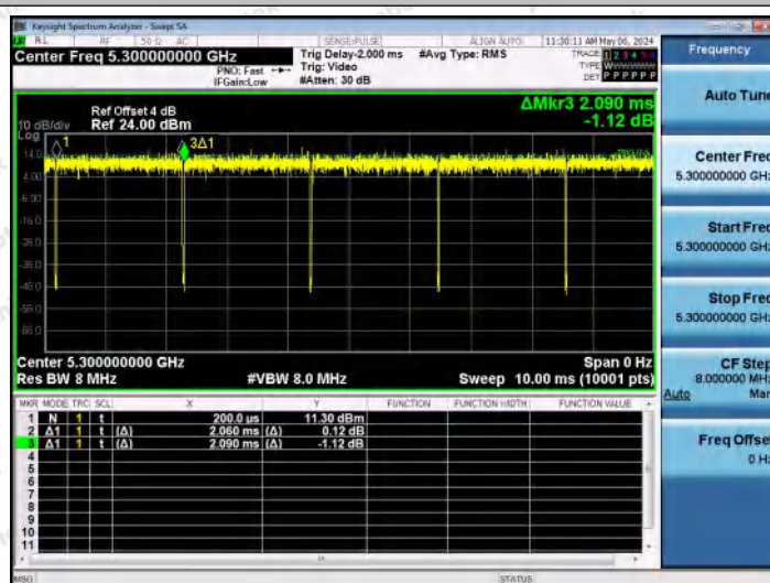
NTNV-11A-Ant0-5300
