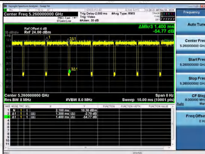
NTNV-11N20MIMO-Ant0-5260
