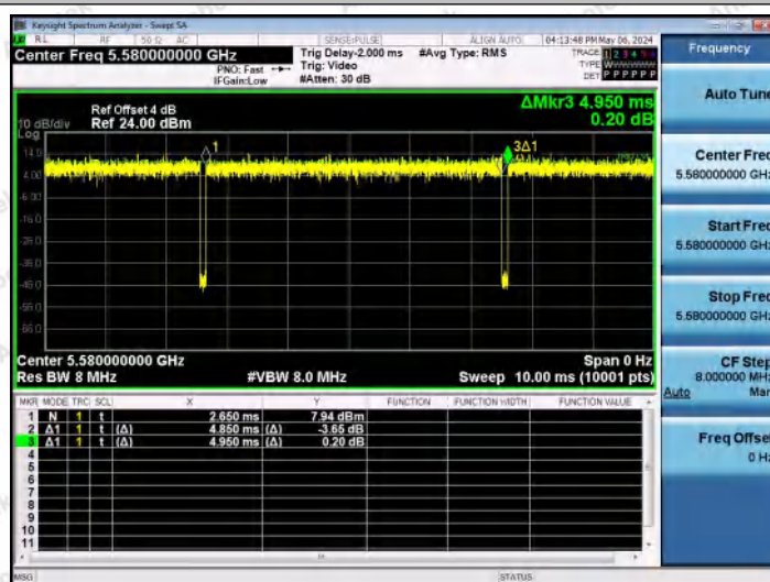
NTNV-11AX20MIMO-Ant1-5580
