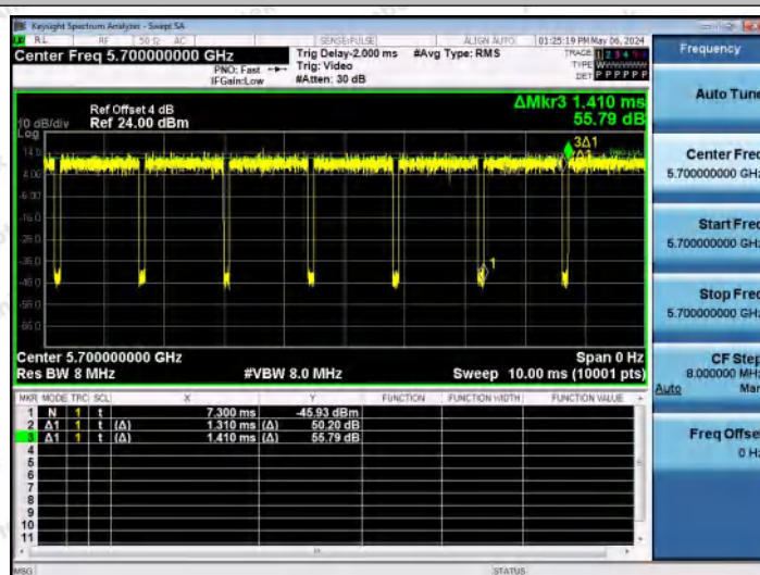
NTNV-11N20MIMO-Ant1-5700
