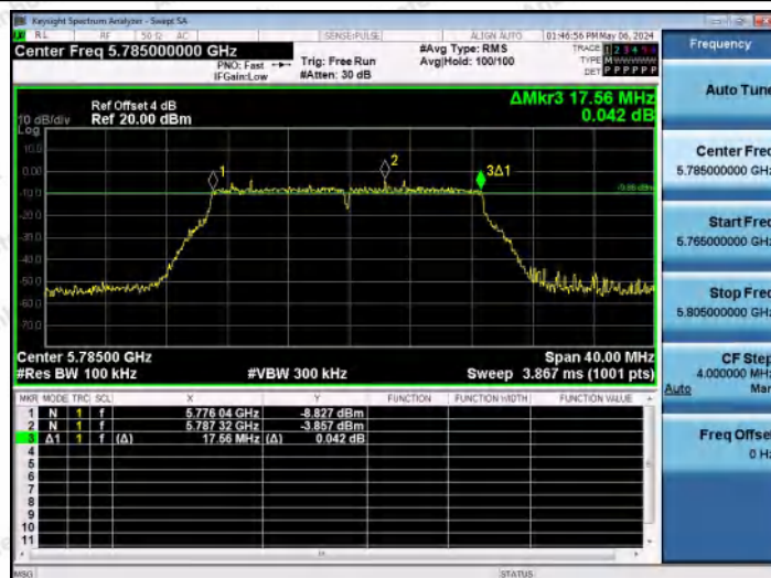
11AC20MIMO-Ant0-5785-PASS
