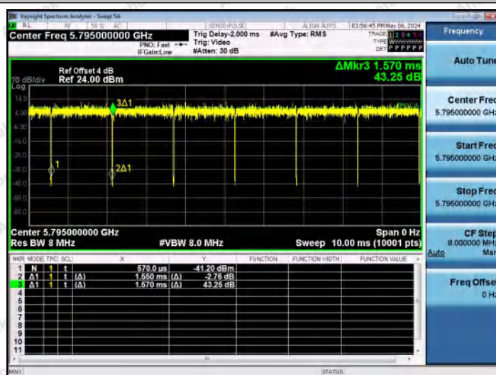
NTNV-11AC40MIMO-Ant0-5795
