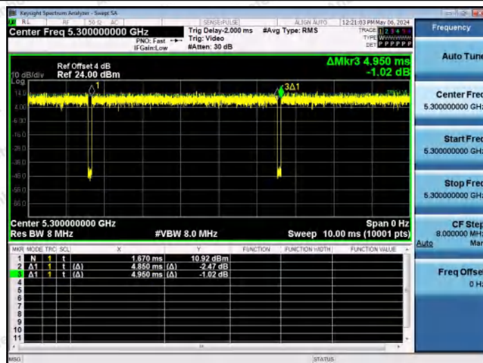
NTNV-11AX20MIMO-Ant0-5300
