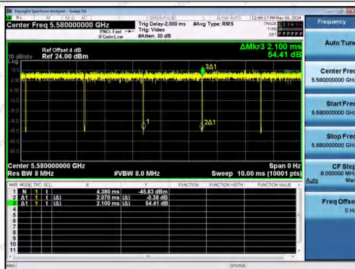
NTNV-11A-Ant0-5580
