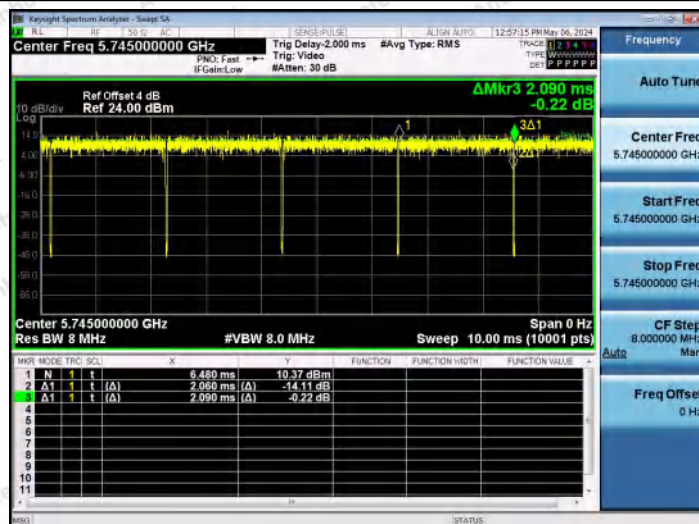
NTNV-11A-Ant0-5745
