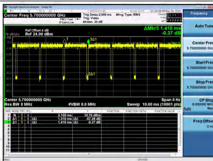
NTNV-11N20MIMO-Ant0-5700
