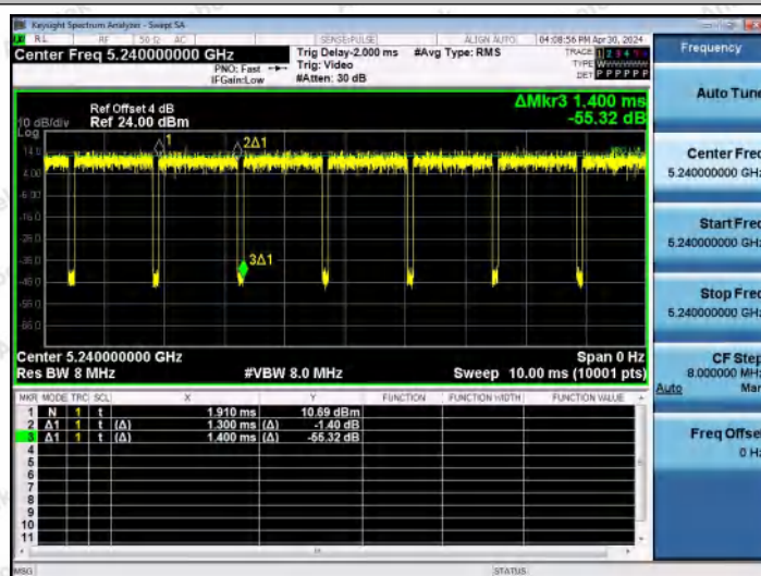
NTNV-11N20MIMO-Ant0-5240
