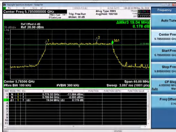
11AX20MIMO-Ant0-5785-PASS
