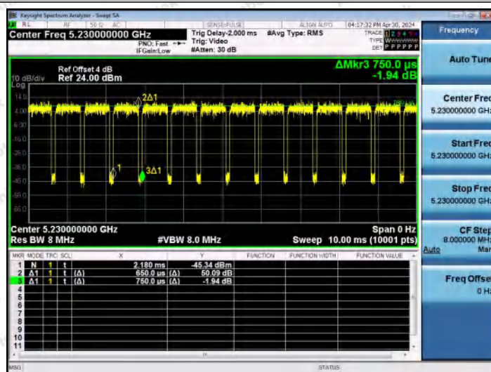
NTVN-11N40MIMO-Ant0-5230
