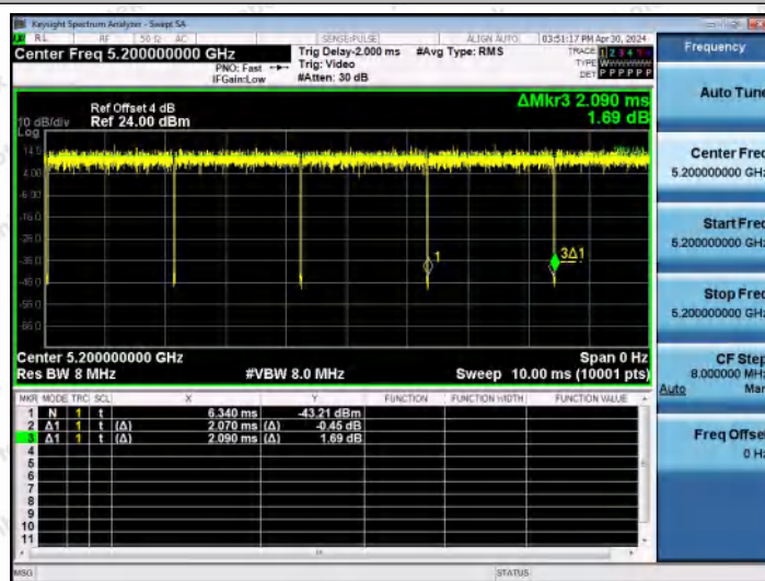
NTNV-11A-Ant0-5200
