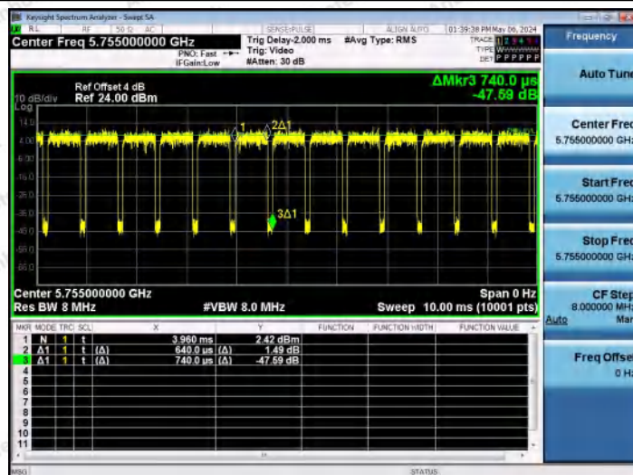
NTNV-11N40MIMO-Ant1-5755
