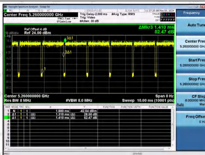
NTNV-11N20MIMO-Ant1-5260
