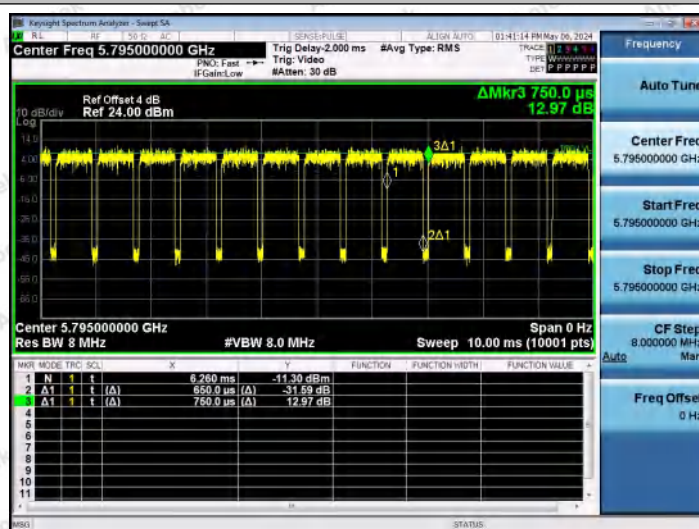
NTNV-11N40MIMO-Ant0-5795
