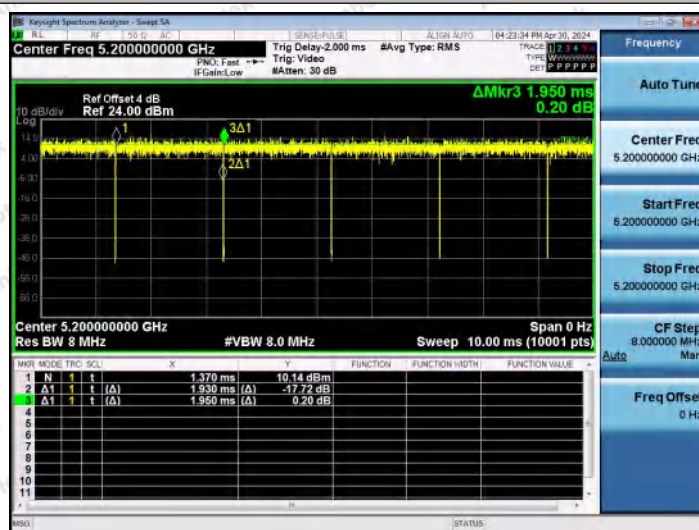
NTNV-11AC20MIMO-Ant0-5200
