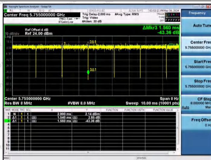
NTNV-11AC40MIMO-Ant0-5755
