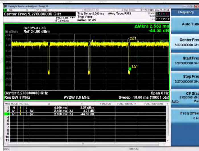
NTNV-11AX40MIMO-Ant0-5270
