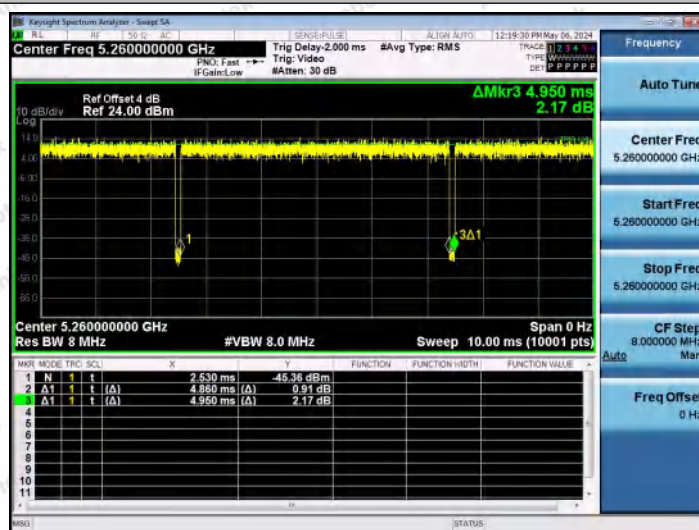
NTNV-11AX20MIMO-Ant1-5260
