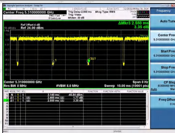
NTNV-11AX40MIMO-Ant1-5310
