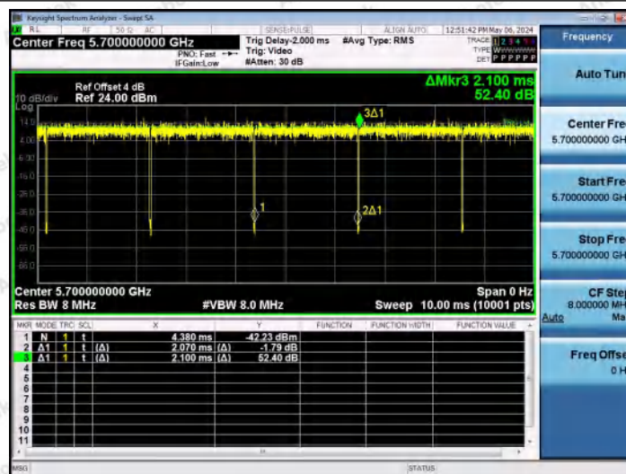
NTNV-11A-Ant0-5700
