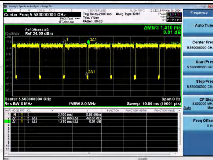
NTNV-11N20MIMO-Ant1-5580
