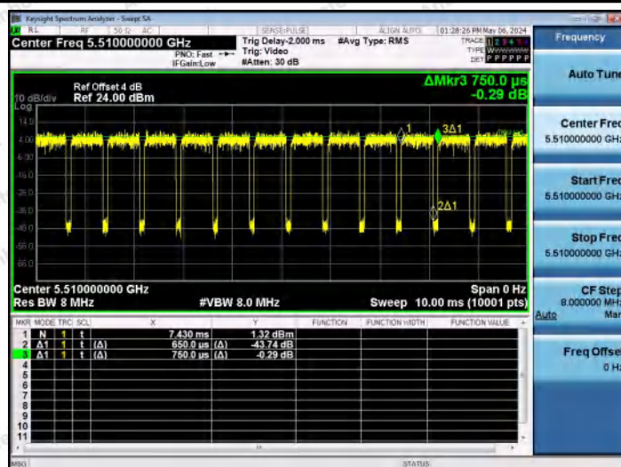
NTNV-11N40MIMO-Ant1-5510
