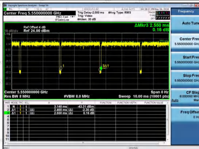
NTNV-11AX40MIMO-Ant1-5550
