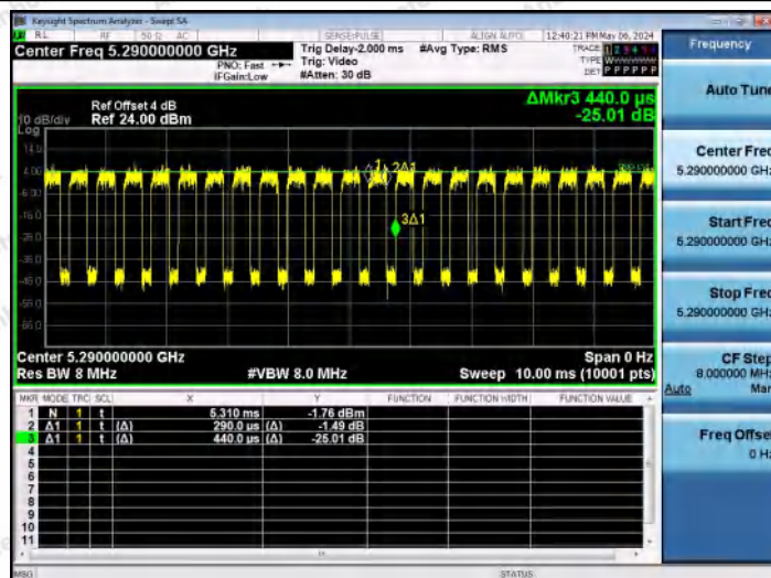
NTNV-11AX80MIMO-Ant0-5290
