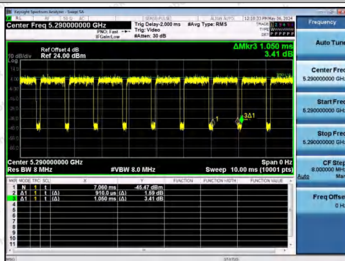
NTNV-11AC80MIMO-Ant0-5290
