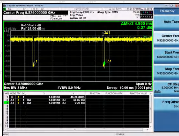
NTNV-11AX20MIMO-Ant0-5825
