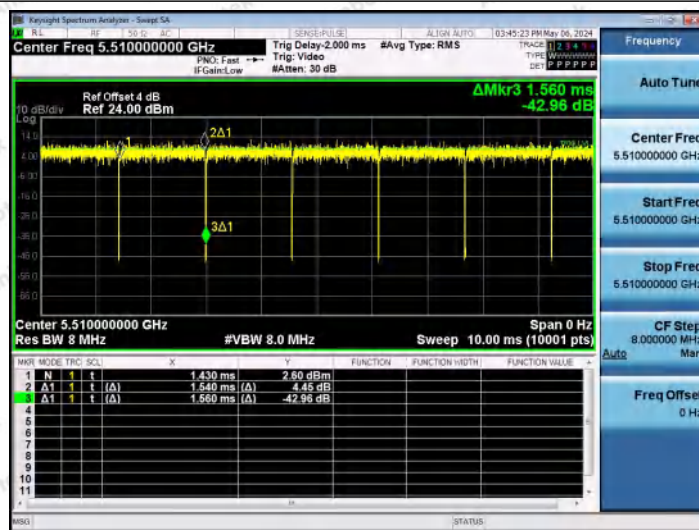
NTNV-11AC40MIMO-Ant0-5510
