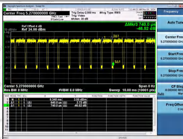
NTNV-11N40MIMO-Ant0-5270
