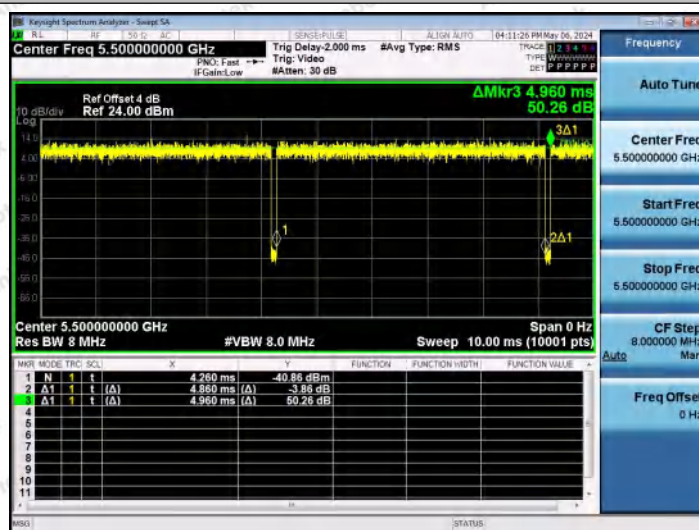
NTNV-11AX20MIMO-Ant1-5500
