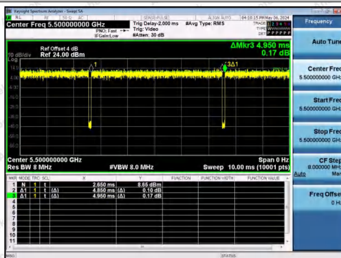
NTNV-11AX20MIMO-Ant0-5500
