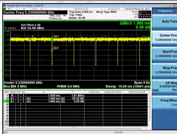
NTNV-11AC40MIMO-Ant0-5230
