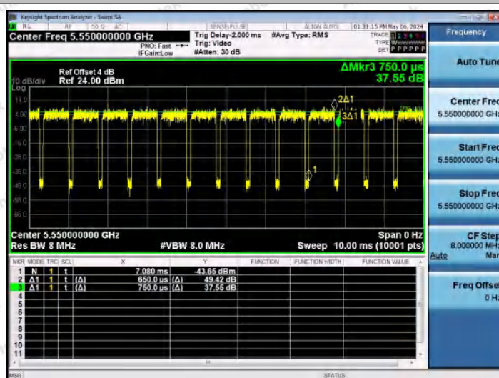
NTNV-11N40MIMO-Ant1-5550
