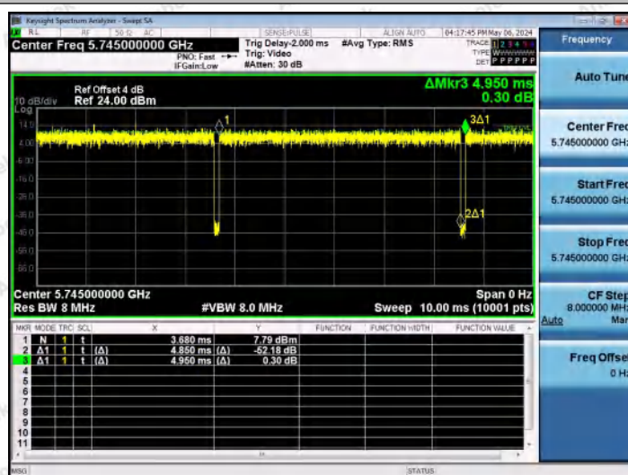
NTNV-11AX20MIMO-Ant0-5745
