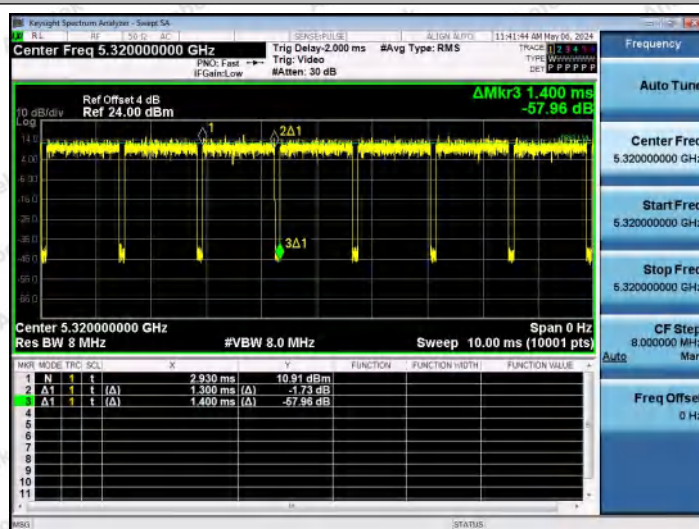
NTVN-11N20MIMO-Ant0-5320
