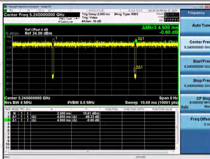
NTNV-11AX20MIMO-Ant0-5240
