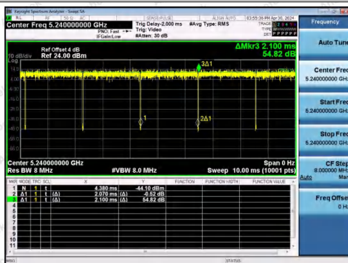
NTNV-11A-Ant0-5240
