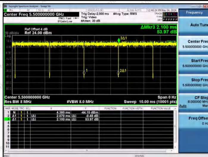
NTNV-11A-Ant0-5500
