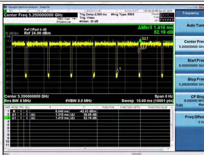
NTVN-11N20MIMO-Ant0-5200
