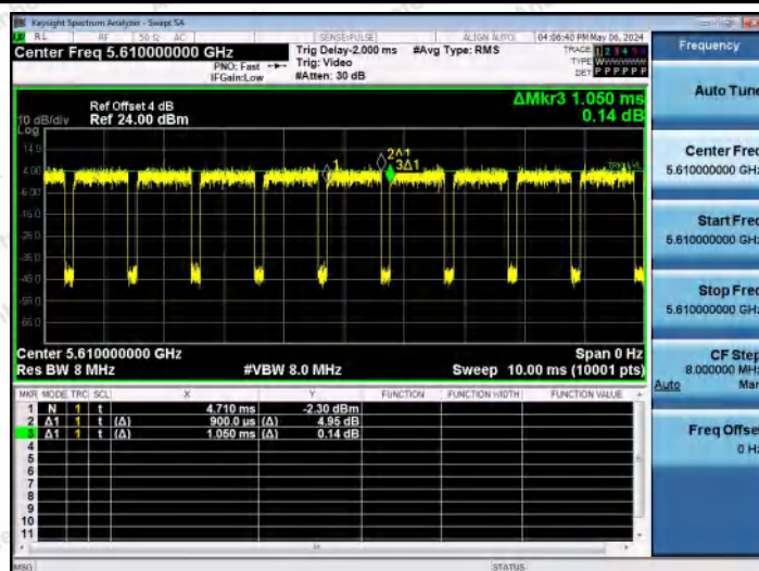
NTNV-11AC80MIMO-Ant0-5610
