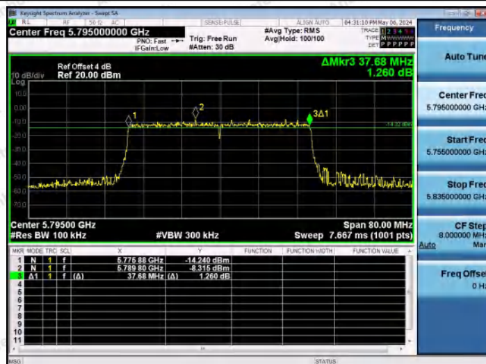
11AX40MIMO-Ant0-5795-PASS
