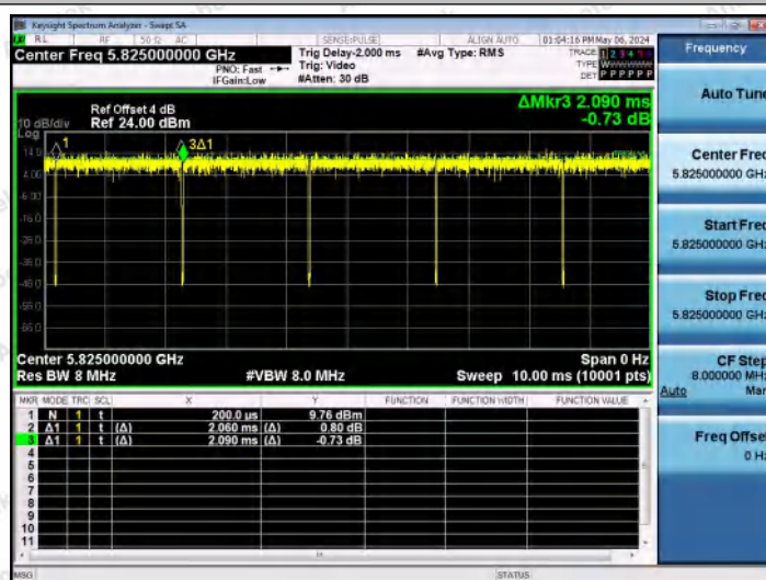
NTNV-11A-Ant0-5825
