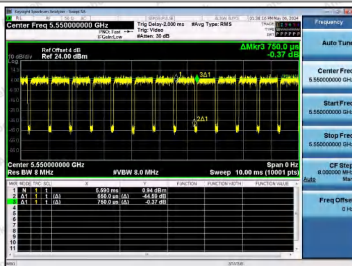
NTNV-11N40MIMO-Ant0-5550
