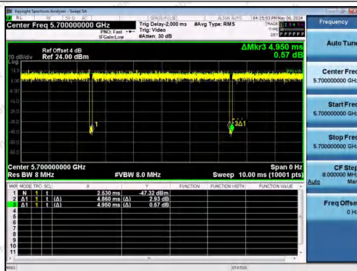
NTNV-11AX20MIMO-Ant0-5700
