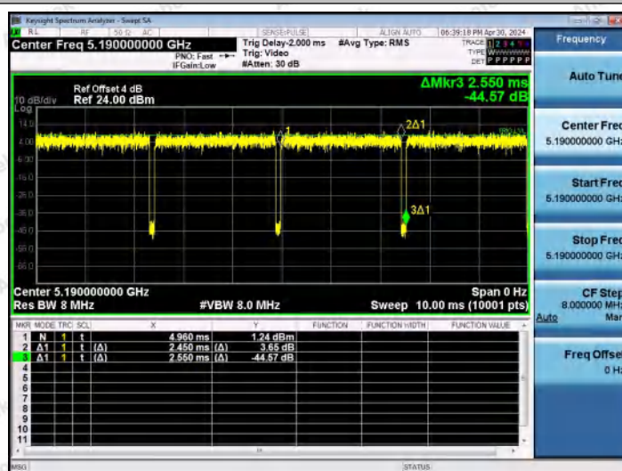
NTNV-11AX40MIMO-Ant0-5190
