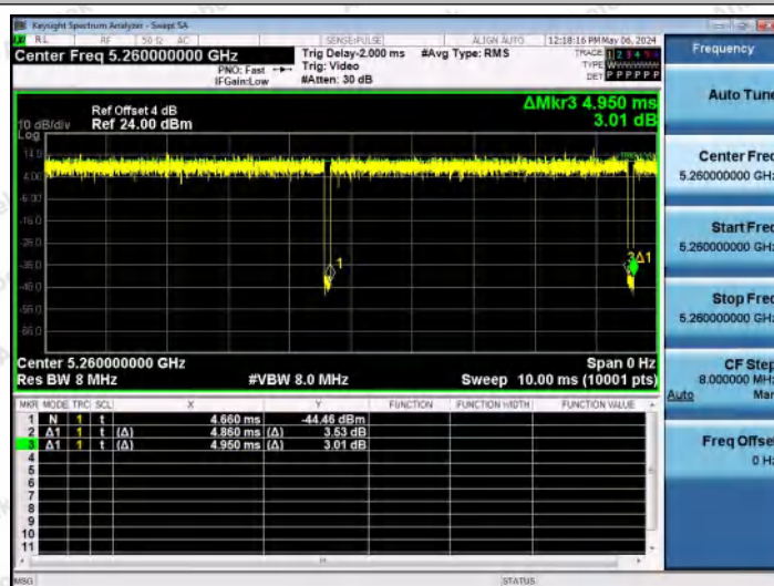
NTNV-11AX20MIMO-Ant0-5260
