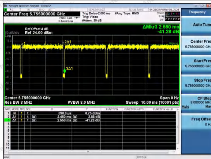
NTNV-11AX40MIMO-Ant0-5755
