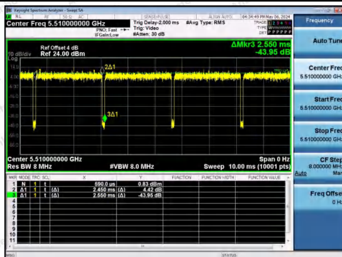
NTNV-11AX40MIMO-Ant0-5510
