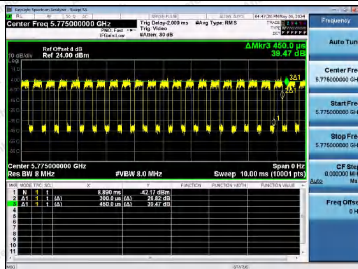
NTNV-11AX80MIMO-Ant0-5775
