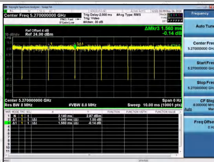
NTNV-11AC40MIMO-Ant0-5270
