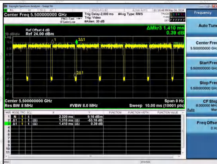
NTNV-11N20MIMO-Ant1-5500
