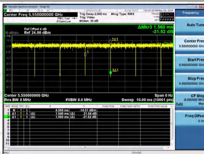
NTNV-11AC40MIMO-Ant0-5550
