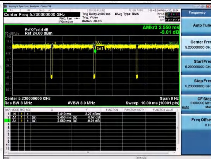
NTNV-11AX40MIMO-Ant0-5230
