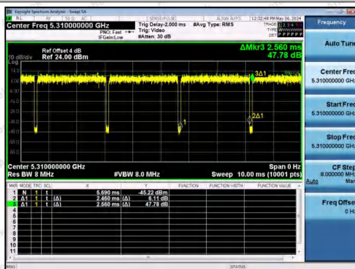
NTNV-11AX40MIMO-Ant0-5310
