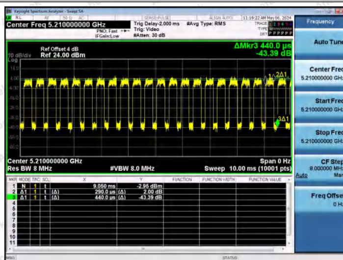
NTNV-11AX80MIMO-Ant0-5210
