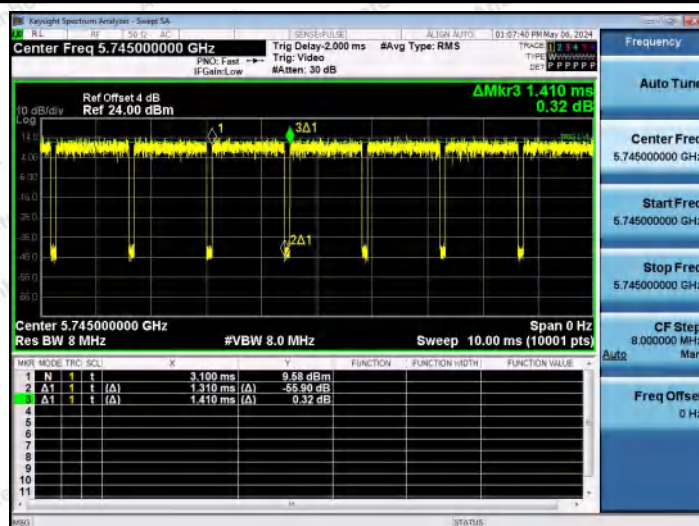
NTVN-11N20MIMO-Ant0-5745
