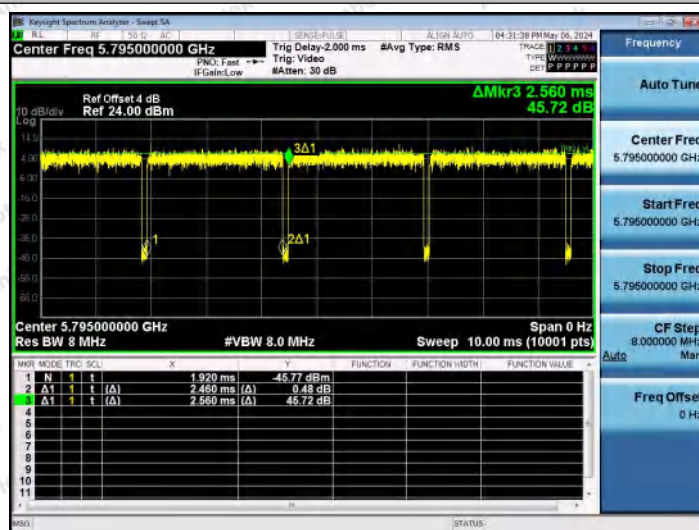
NTNV-11AX40MIMO-Ant0-5795
