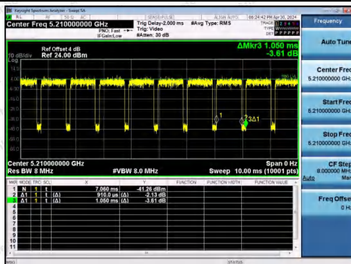
NTNV-11AC80MIMO-Ant0-5210
