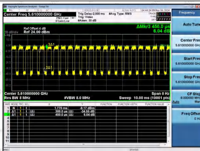
NTNV-11AX80MIMO-Ant0-5610
